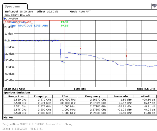
20MHz_15kHz_2560MHz_DFT-s-OFDM QPSK_RB100@0&-21.05 dBm
