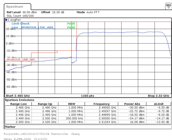
20MHz_15kHz_2510MHz_DFT-s-OFDM QPSK_RB100@0&-30.50 dBm
