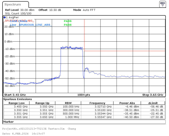
30MHz_30kHz_3535MHz_DFT-s-OFDM QPSK_RB75@0&-35.45 dBm
