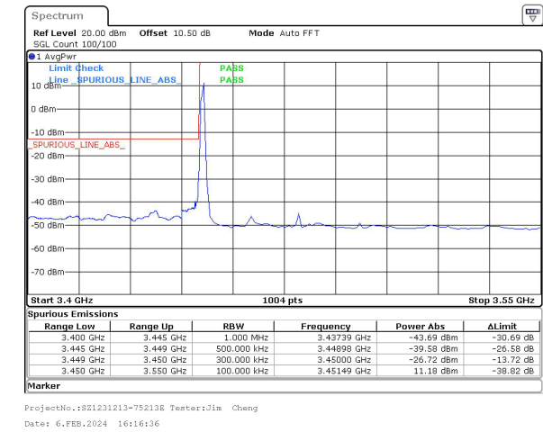
30MHz_30kHz_3465MHz_DFT-s-OFDM QPSK_RB1@0&-26.72 dBm
