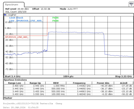
70MHz_30kHz_3485MHz_DFT-s-OFDM QPSK_RB180@0&-36.17 dBm
