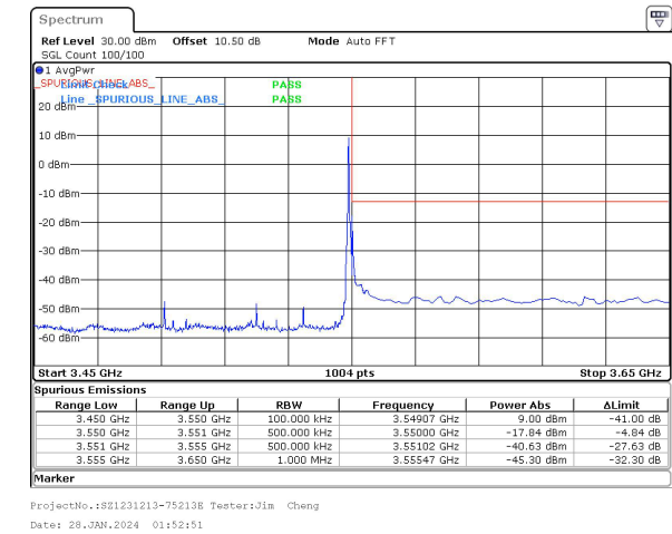
60MHz_30kHz_3520MHz_DFT-s-OFDM QPSK_RB1@161&-17.84 dBm
