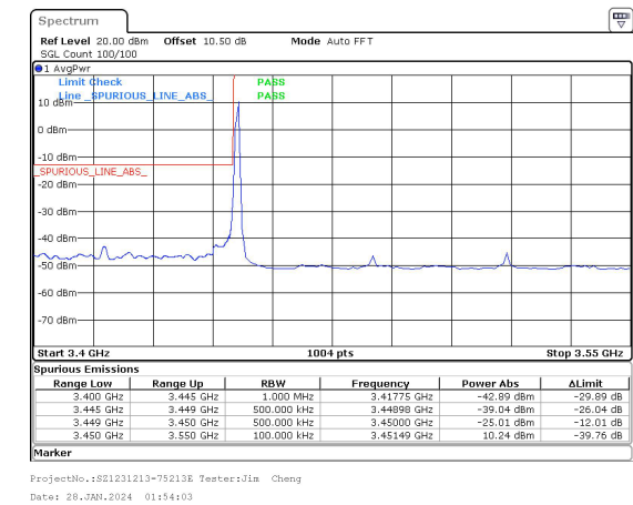
70MHz_30kHz_3485MHz_DFT-s-OFDM QPSK_RB1@0&-25.01 dBm
