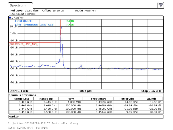
40MHz_30kHz_3470MHz_DFT-s-OFDM QPSK_RB1@0&-25.98 dBm
