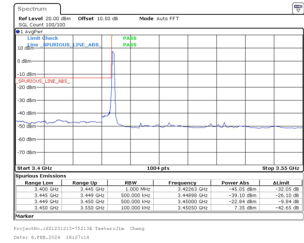
60MHz_30kHz_3480MHz_DFT-s-OFDM QPSK_RB1@0&-22.84 dBm
