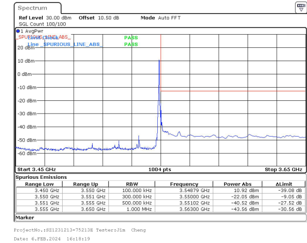
30MHz_30kHz_3535MHz_DFT-s-OFDM QPSK_RB1@77&-22.05 dBm
