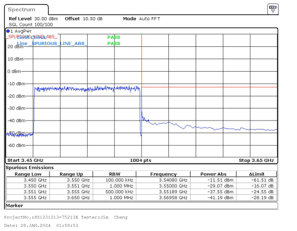
80MHz_30kHz_3510MHz_DFT-s-OFDM QPSK_RB216@0&-29.07 dBm
