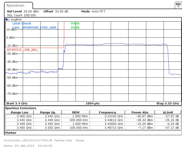
90MHz_30kHz_3495MHz_DFT-s-OFDM QPSK_RB243@0&-15.24 dBm
