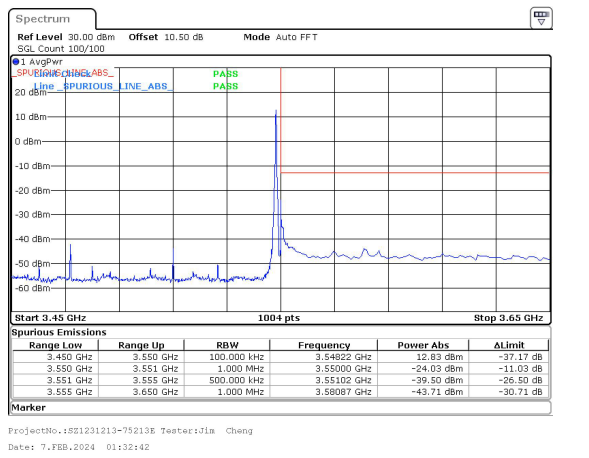
80MHz_30kHz_3510MHz_DFT-s-OFDM QPSK_RB1@216&-24.03 dBm
