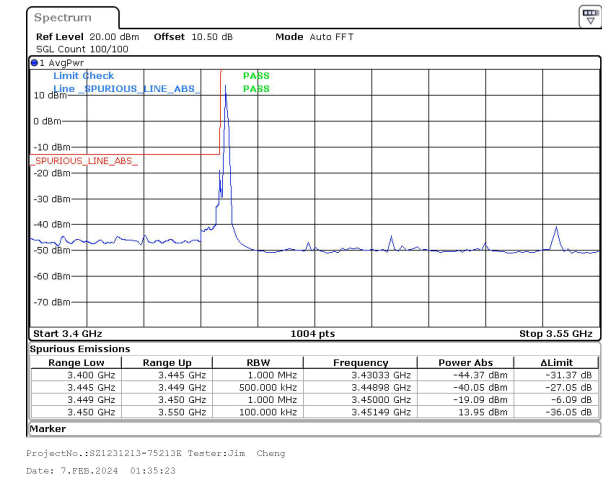
90MHz_30kHz_3495MHz_DFT-s-OFDM QPSK_RB1@0&-19.09 dBm
