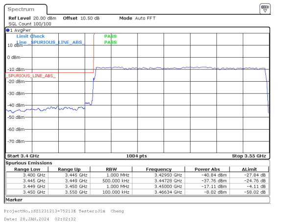
100MHz_30kHz_3500MHz_DFT-s-OFDM QPSK_RB270@0&-17.11 dBm
