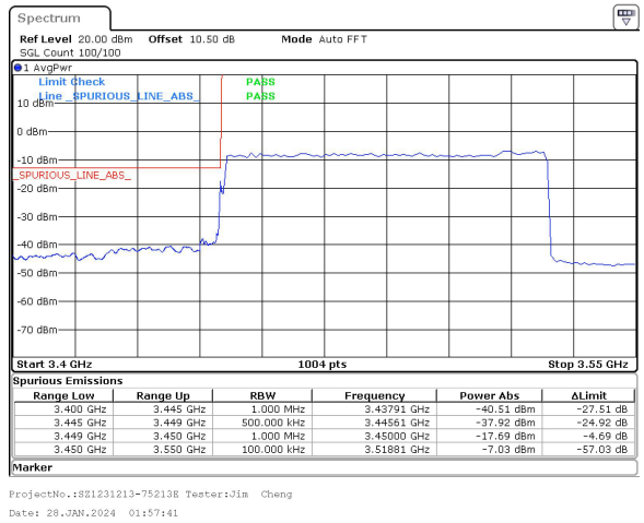
80MHz_30kHz_3490MHz_DFT-s-OFDM QPSK_RB216@0&-17.69 dBm
