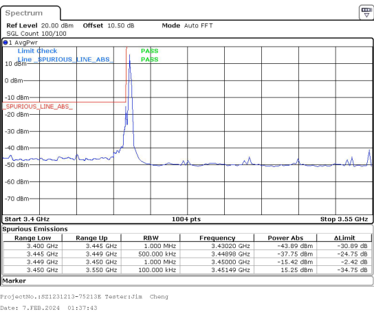
100MHz_30kHz_3500MHz_DFT-s-OFDM QPSK_RB1@0&-15.42 dBm
