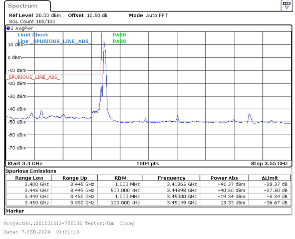
80MHz_30kHz_3490MHz_DFT-s-OFDM QPSK_RB1@0&-19.34 dBm
