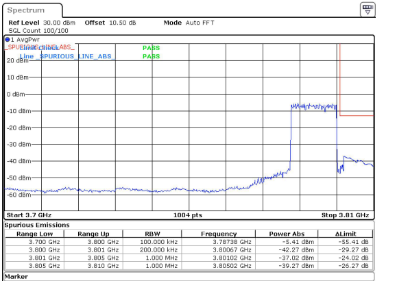
15MHz_15kHz_3792.5MHz_DFT-s-OFDM QPSK_RB75@0&-37.02 dBm
