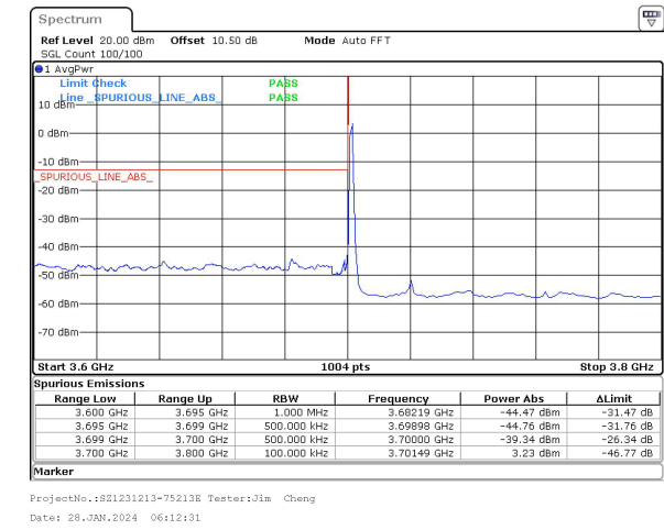
40MHz_30kHz_3720MHz_DFT-s-OFDM QPSK_RB1@0&-39.34 dBm
