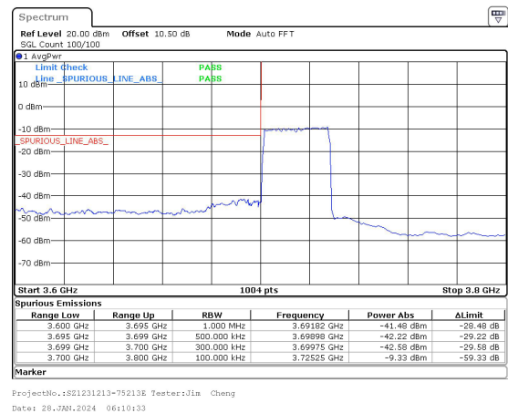
30MHz_30kHz_3715MHz_DFT-s-OFDM QPSK_RB75@0&-41.48 dBm
