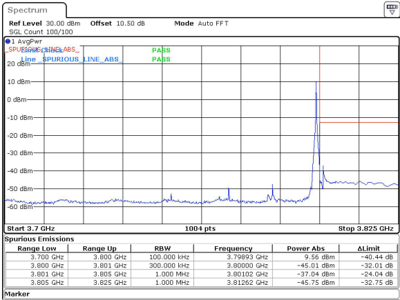
30MHz_30kHz_3785MHz_DFT-s-OFDM QPSK_RB1@77&-37.04 dBm
