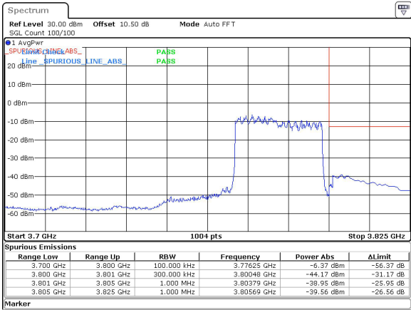
30MHz_30kHz_3785MHz_DFT-s-OFDM QPSK_RB75@0&-38.95 dBm
