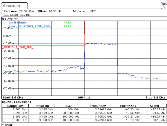
40MHz_15kHz_3720MHz_DFT-s-OFDM QPSK_RB216@0&-29.27 dBm
