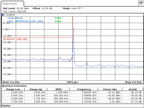
40MHz_15kHz_3720MHz_DFT-s-OFDM QPSK_RB1@0&-36.26 dBm
