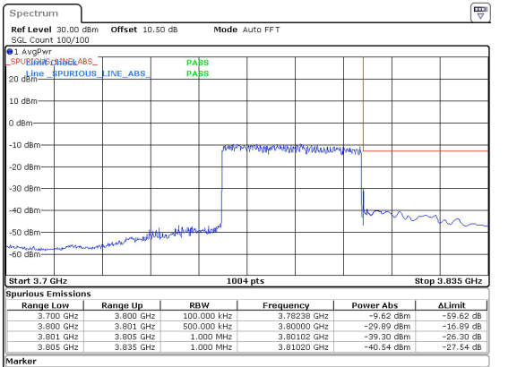
40MHz_15kHz_3780MHz_DFT-s-OFDM QPSK_RB216@0&-29.89 dBm
