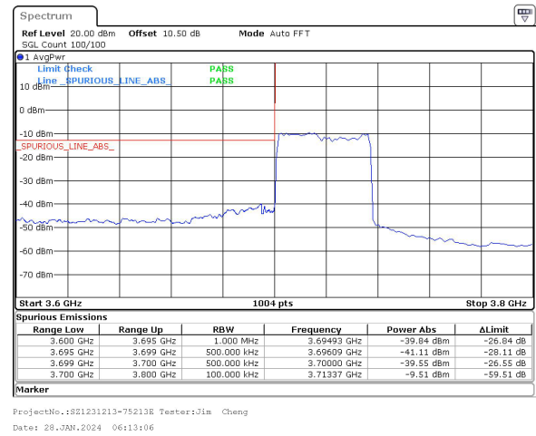
40MHz_30kHz_3720MHz_DFT-s-OFDM QPSK_RB100@0&-39.55 dBm
