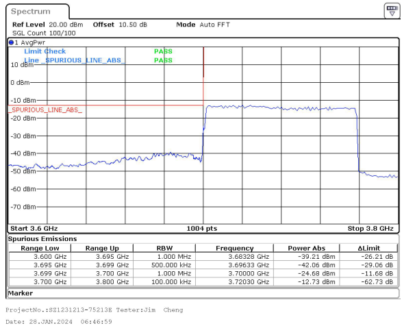
80MHz_30kHz_3740MHz_DFT-s-OFDM QPSK_RB216@0&-24.68 dBm
