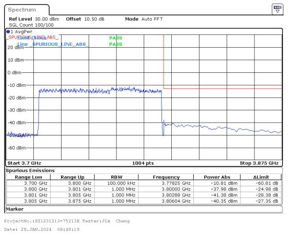
80MHz_30kHz_3760MHz_DFT-s-OFDM QPSK_RB216@0&-37.98 dBm
