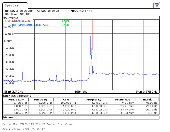
80MHz_30kHz_3760MHz_DFT-s-OFDM QPSK_RB1@216&-35.71 dBm
