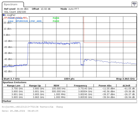
70MHz_30kHz_3765MHz_DFT-s-OFDM QPSK_RB180@0&-39.57 dBm
