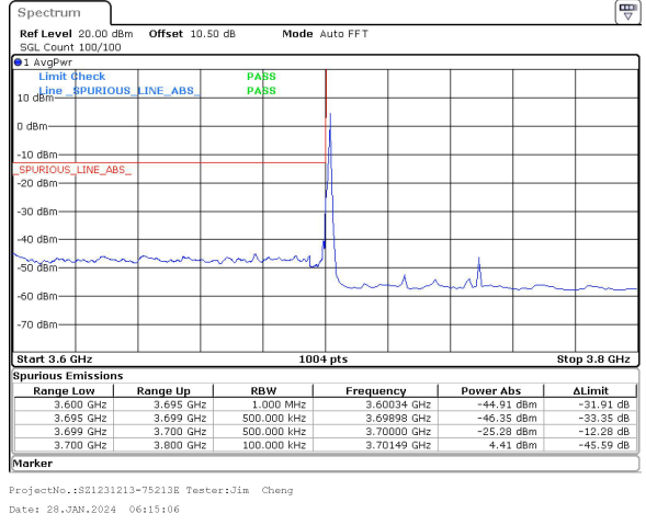
50MHz_30kHz_3725MHz_DFT-s-OFDM QPSK_RB1@0&-25.28 dBm
