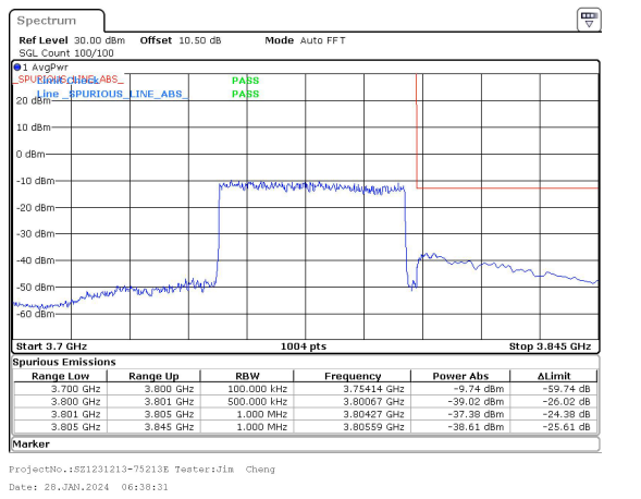
50MHz_30kHz_3775MHz_DFT-s-OFDM QPSK_RB128@0&-37.38 dBm
