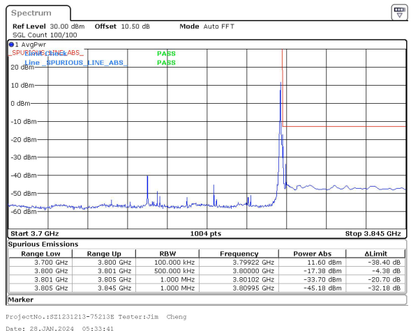
50MHz_15kHz_3775MHz_DFT-s-OFDM QPSK_RB1@269&-17.38 dBm
