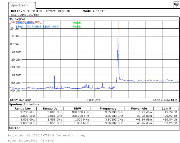
60MHz_30kHz_3770MHz_DFT-s-OFDM QPSK_RB1@161&-33.92 dBm
