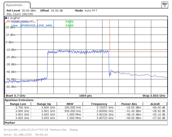
60MHz_30kHz_3770MHz_DFT-s-OFDM QPSK_RB162@0&-38.15 dBm
