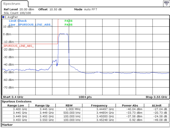
10MHz_30kHz_3455MHz_DFT-s-OFDM QPSK_RB24@0 -33.73 dBm
