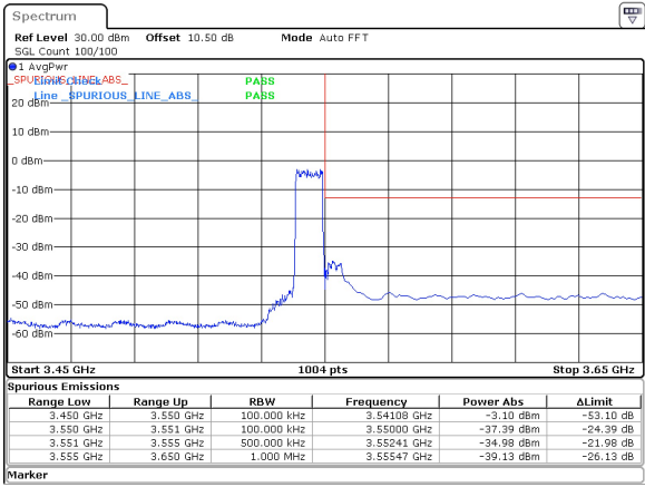
10MHz_30kHz_3455MHz_DFT-s-OFDM QPSK_RB24@0 -34.98 dBm
