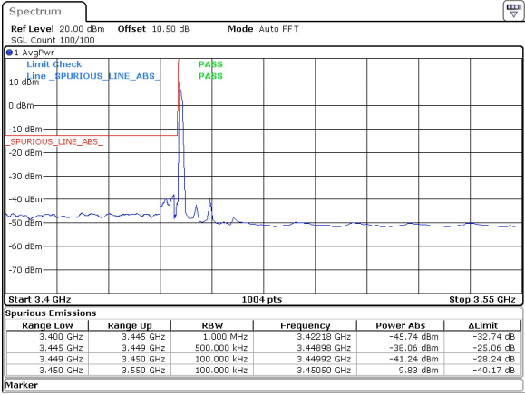
10MHz_30kHz_3455MHz_DFT-s-OFDM QPSK_RB1@0 -38.06 dBm
