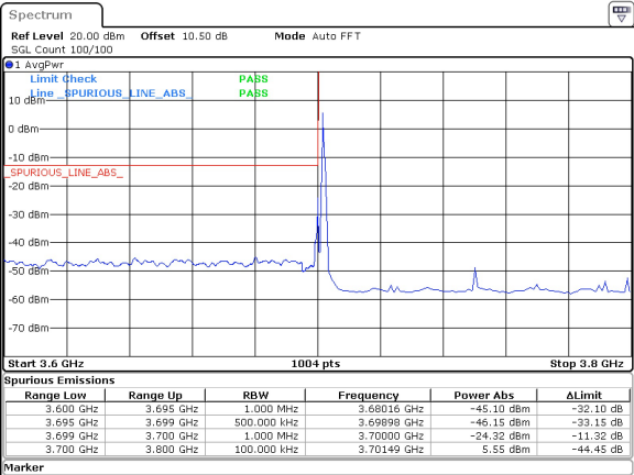
100MHz_30kHz_3750MHz_DFT-s-OFDM QPSK_RB1@0 -24.32 dBm
