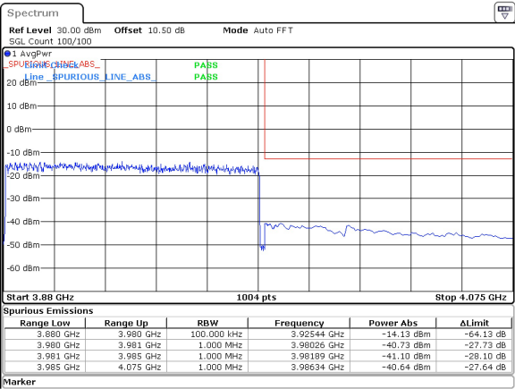
100MHz_30kHz_3930MHz_DFT-s-OFDM QPSK_RB270@0 -40.64 dBm
