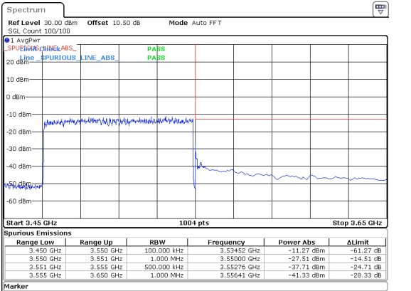
80MHz_30kHz_3510MHz_DFT-s-OFDM QPSK_RB216@0 -27.51 dBm
