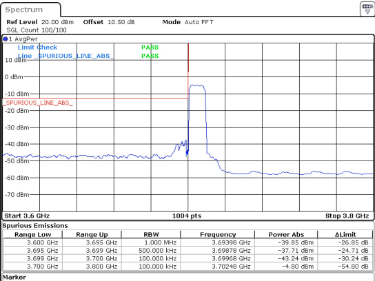
10MHz_15kHz_3705MHz_DFT-s-OFDM QPSK_RB50@0 -37.71 dBm
