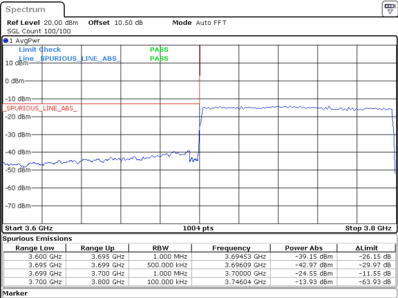
100MHz_30kHz_3750MHz_DFT-s-OFDM QPSK_RB270@0 -24.55 dBm
