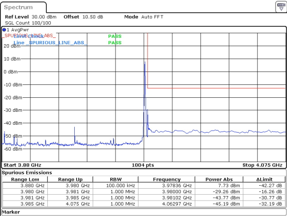
100MHz_30kHz_3930MHz_DFT-s-OFDM QPSK_RB1@272 -29.26 dBm
