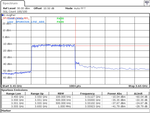
60MHz_30kHz_3520MHz_DFT-s-OFDM QPSK_RB162@0 -35.35 dBm
