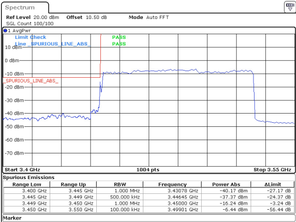
80MHz_30kHz_3490MHz_DFT-s-OFDM QPSK_RB216@0 -16.24 dBm
