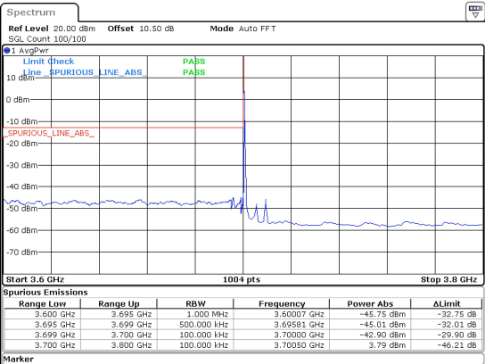
10MHz_15kHz_3705MHz_DFT-s-OFDM QPSK_RB1@0 -42.90 dBm
