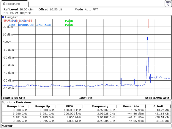
20MHz_30kHz_3970MHz_DFT-s-OFDM QPSK_RB1@50 -41.51 dBm
