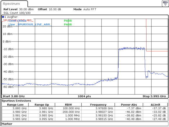
20MHz_30kHz_3970MHz_DFT-s-OFDM QPSK_RB50@0 -38.82 dBm
