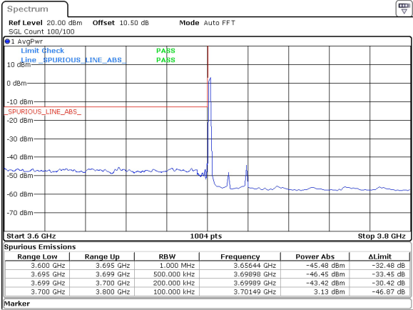
20MHz_30kHz_3710MHz_DFT-s-OFDM QPSK_RB1@0 -43.42 dBm
