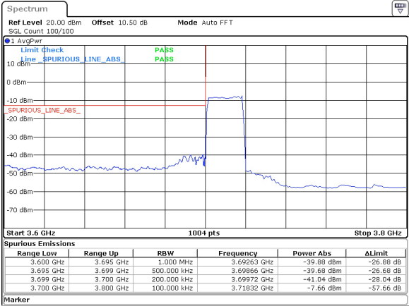
20MHz_30kHz_3710MHz_DFT-s-OFDM QPSK_RB50@0 -39.68 dBm
