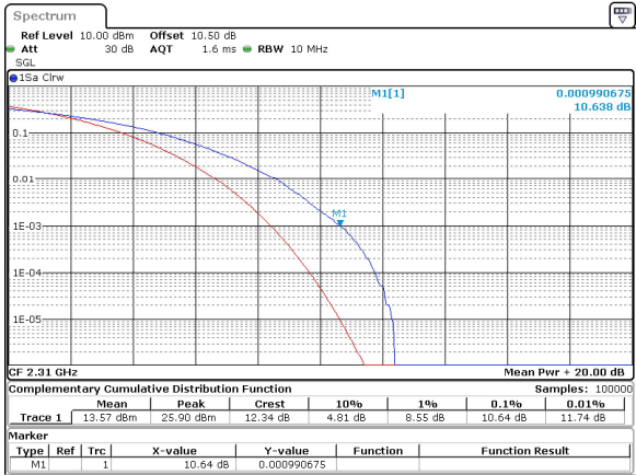
10MHz_30kHz_2310MHz_CP-OFDM 256 QAM_RB24@0 10.64 dB
