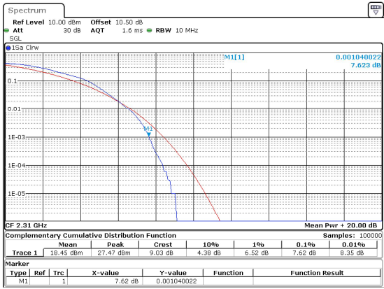
10MHz_30kHz_2310MHz_DFT-s-OFDM 16 QAM_RB24@0 7.62 dB
