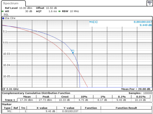
10MHz_30kHz_2310MHz_CP-OFDM QPSK_RB24@0 9.45 dB
