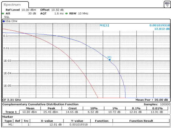
10MHz_30kHz_2310MHz_DFT-s-OFDM 256 QAM_RB24@0 12.81 dB
