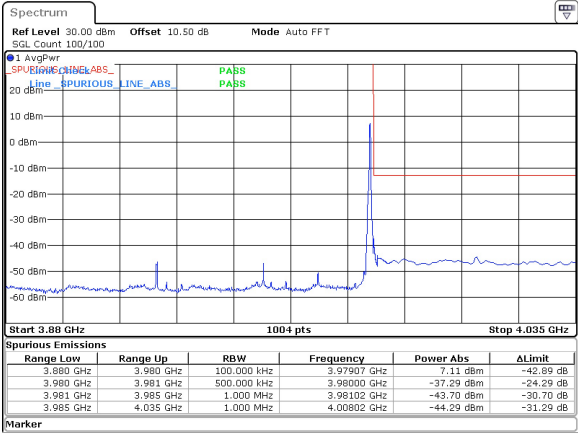
60MHz_30kHz_3950MHz_DFT-s-OFDM QPSK_RB1@161 -37.29 dBm
