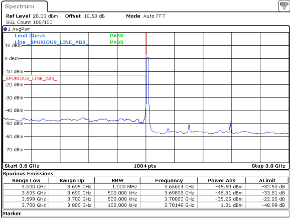
60MHz_30kHz_3730MHz_DFT-s-OFDM QPSK_RB1@0 -35.25 dBm
