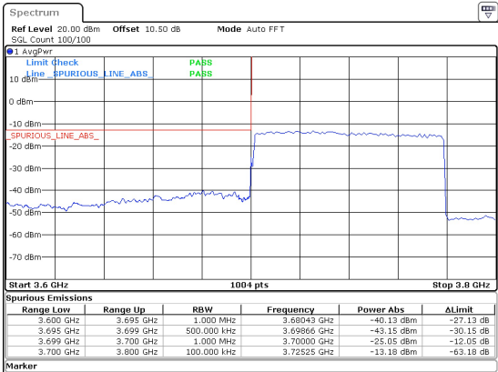
80MHz_30kHz_3740MHz_DFT-s-OFDM QPSK_RB216@0 -25.05 dBm
