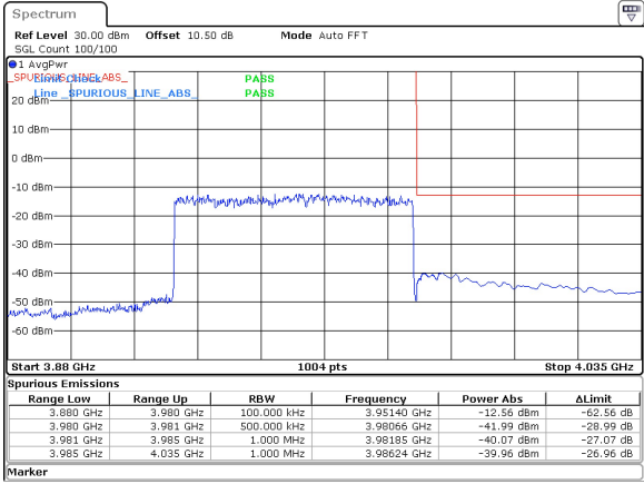
60MHz_30kHz_3950MHz_DFT-s-OFDM QPSK_RB162@0 -39.96 dBm
