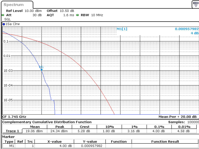
10MHz_15kHz_1745MHz_DFT-s-OFDM PI/2 BPSK_RB50@0 4.00 dB
