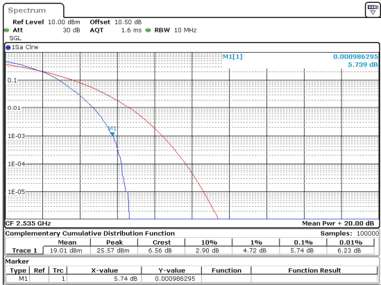
10MHz_15kHz_2535MHz_DFT-s-OFDM 16 QAM_RB50@0 5.74 dB
