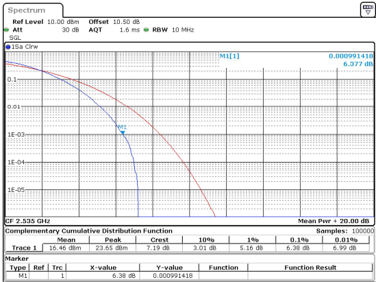
10MHz_15kHz_2535MHz_DFT-s-OFDM 256 QAM_RB50@0 6.38 dB
