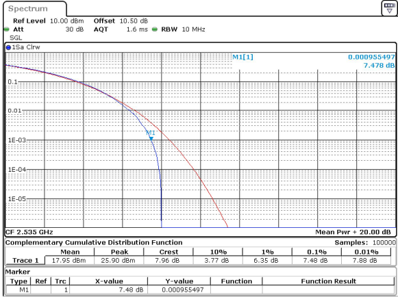
10MHz_15kHz_2535MHz_CP-OFDM QPSK_RB52@0 7.48 dB
