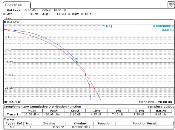
10MHz_15kHz_3500MHz_DFT-s-OFDM 64 QAM_RB50@0 8.58 dB
