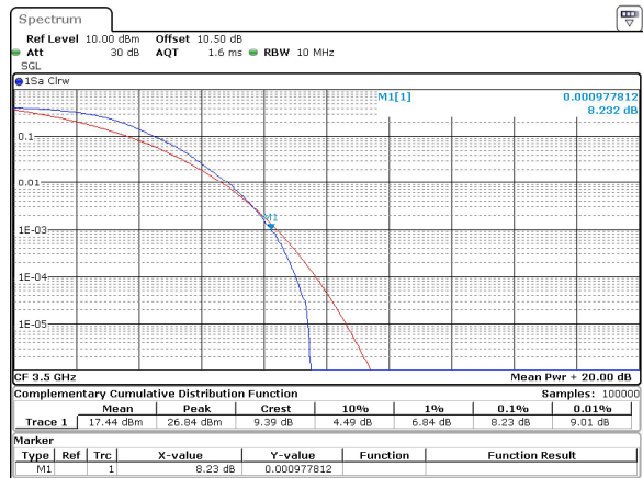
10MHz_15kHz_3500MHz_DFT-s-OFDM QPSK_RB50@0 8.23 dB
