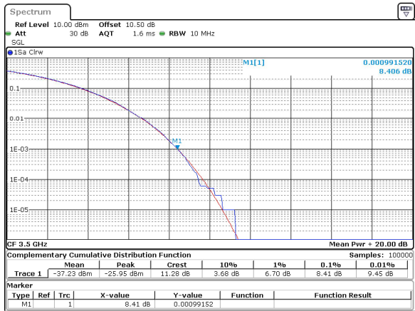
10MHz_15kHz_3500MHz_DFT-s-OFDM PI/2 BPSK_RB50@0 8.41 dB
