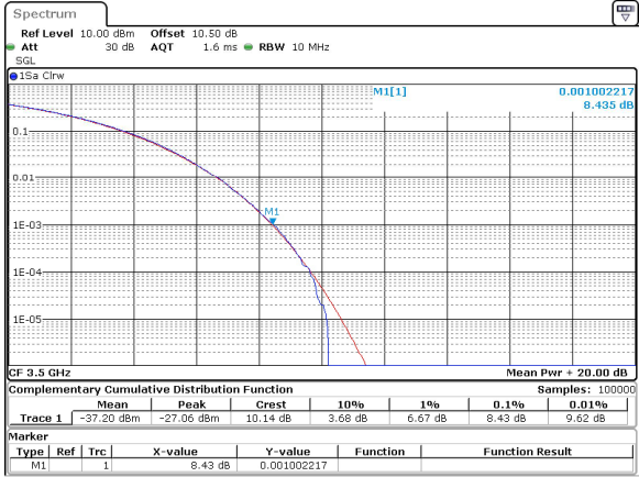
10MHz_15kHz_3500MHz_CP-OFDM QPSK_RB52@0 8.43 dB
