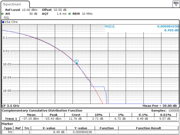
10MHz_30kHz_3500MHz_CP-OFDM QPSK_RB24@0 8.49 dB
