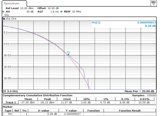
10MHz_30kHz_3500MHz_DFT-s-OFDM QPSK_RB24@0 8.58 dB
