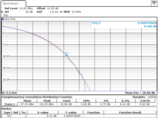
10MHz_30kHz_3500MHz_DFT-s-OFDM PI/2 BPSK_RB24@0 8.41 dB
