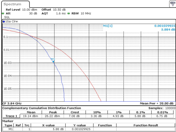
10MHz_15kHz_3840MHz_DFT-s-OFDM PI/2 BPSK_RB50@0 5.88 dB
