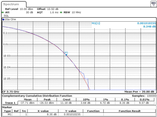
10MHz_15kHz_3750MHz_DFT-s-OFDM 256 QAM_RB50@0 8.35 dB
