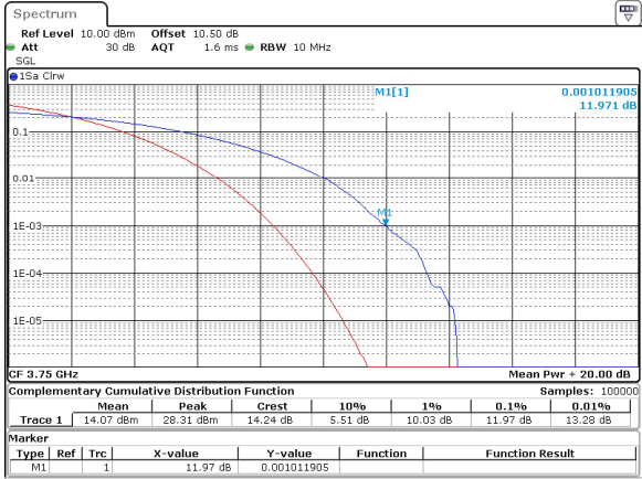
10MHz_15kHz_3750MHz_CP-OFDM QPSK_RB52@0 11.97 dB
