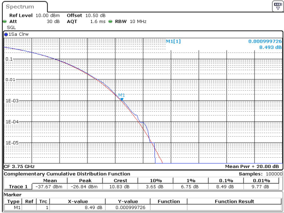
10MHz_30kHz_3750MHz_CP-OFDM 16 QAM_RB24@0 8.49 dB
