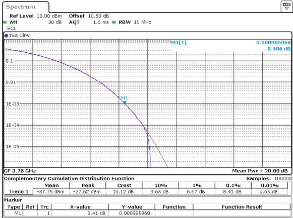
10MHz_15kHz_3750MHz_DFT-s-OFDM PI/2 BPSK_RB50@0 8.41 dB
