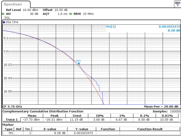
10MHz_30kHz_3750MHz_DFT-s-OFDM 16 QAM_RB24@0 8.58 dB
