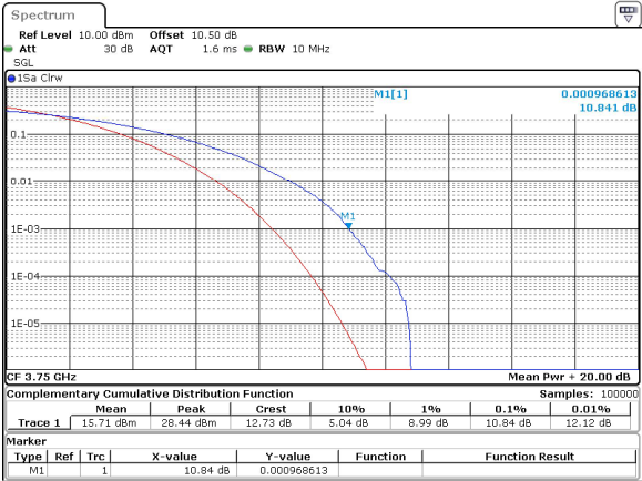
10MHz_30kHz_3750MHz_CP-OFDM QPSK_RB24@0 10.84 dB
