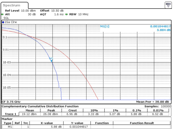
10MHz_30kHz_3750MHz_DFT-s-OFDM PI/2 BPSK_RB24@0 5.88 dB
