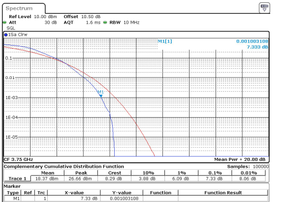
10MHz_30kHz_3750MHz_DFT-s-OFDM QPSK_RB24@0 7.33 dB
