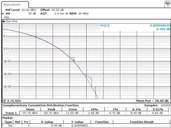
10MHz_30kHz_3750MHz_DFT-s-OFDM 64 QAM_RB24@0 8.49 dB
