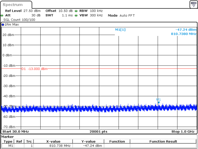
20MHz_15kHz_1770MHz_DFT-s-OFDM QPSK_RB1@105 -47.24 dBm
