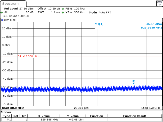
20MHz_15kHz_1720MHz_DFT-s-OFDM QPSK_RB1@0 -46.48 dBm
