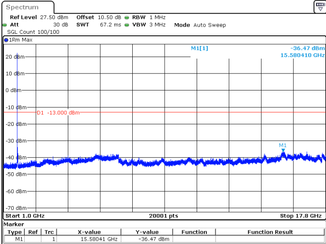
20MHz_15kHz_1720MHz_DFT-s-OFDM QPSK_RB1@0 -36.47 dBm
