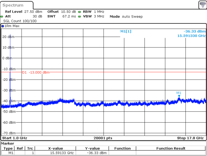
20MHz_15kHz_1745MHz_DFT-s-OFDM QPSK_RB1@0 -36.33 dBm
