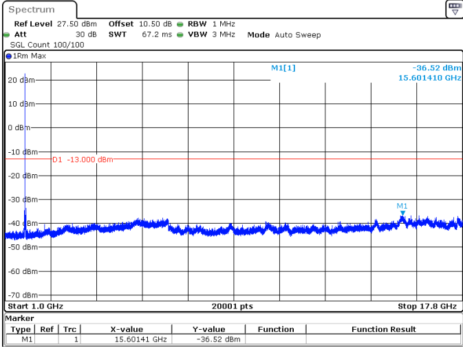
20MHz_15kHz_1720MHz_DFT-s-OFDM QPSK_RB1@105 -36.52 dBm
