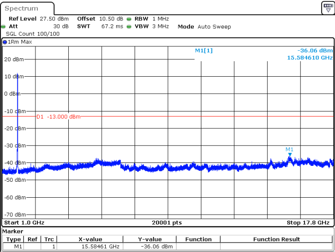
20MHz_15kHz_1770MHz_DFT-s-OFDM QPSK_RB100@0 -36.06 dBm
