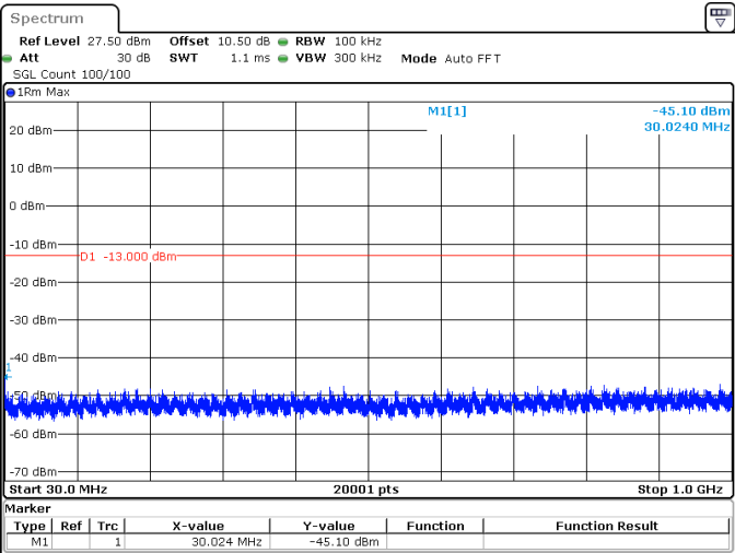
20MHz_15kHz_1770MHz_DFT-s-OFDM QPSK_RB1@0 -45.10 dBm
