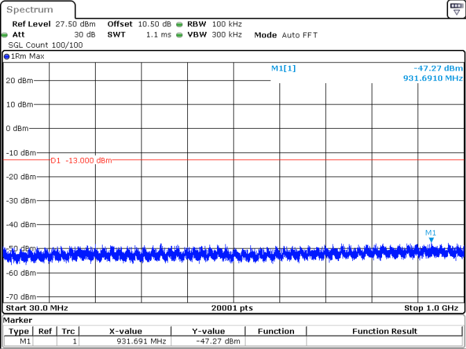
20MHz_15kHz_1720MHz_DFT-s-OFDM QPSK_RB1@105 -47.27 dBm
