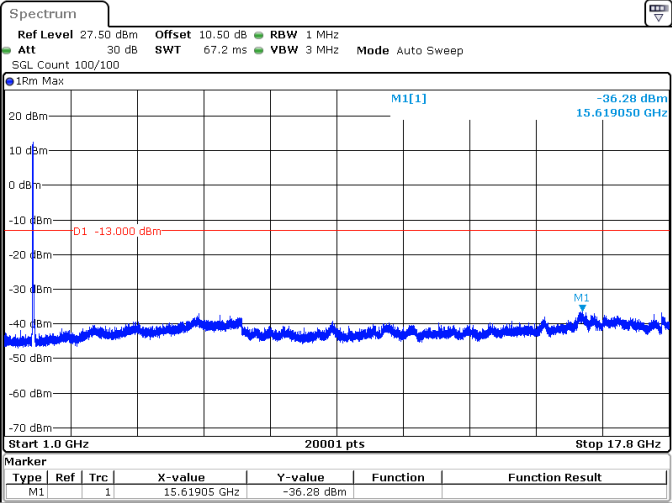
20MHz_15kHz_1720MHz_DFT-s-OFDM QPSK_RB100@0 -36.28 dBm
