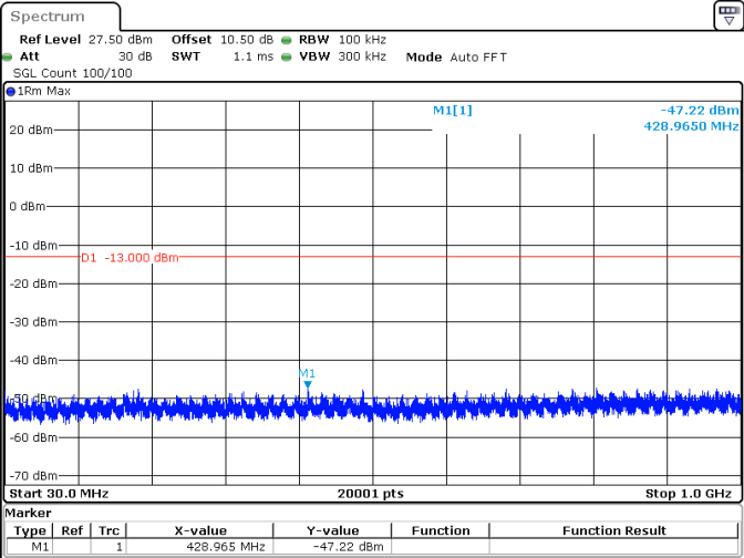
40MHz_15kHz_1760MHz_DFT-s-OFDM QPSK_RB1@0 -47.22 dBm
