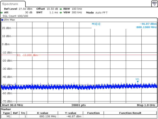
20MHz_15kHz_1770MHz_DFT-s-OFDM QPSK_RB100@0 -46.87 dBm
