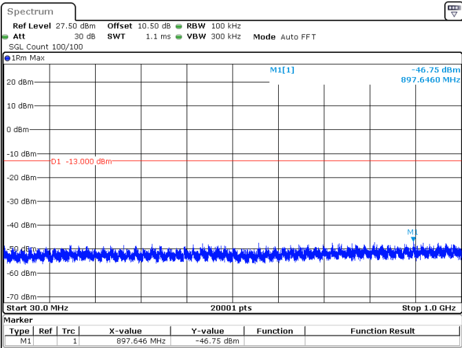
20MHz_15kHz_1745MHz_DFT-s-OFDM QPSK_RB1@0 -46.75 dBm
