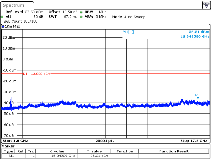
20MHz_15kHz_1770MHz_DFT-s-OFDM QPSK_RB1@0 -36.51 dBm
