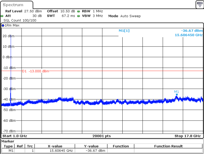
20MHz_15kHz_1770MHz_DFT-s-OFDM QPSK_RB1@105 -36.67 dBm
