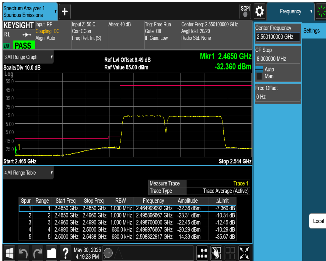
7C 16QAM PCC BW=15MHz Ch=3179 RB=1@0,SCC BW=20MHz Ch=3350 RB=1@99
