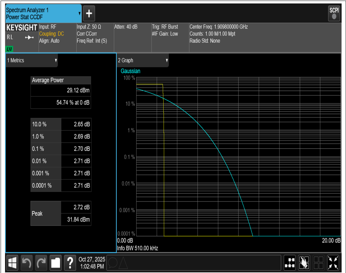
GPRS1900 Channel=810
