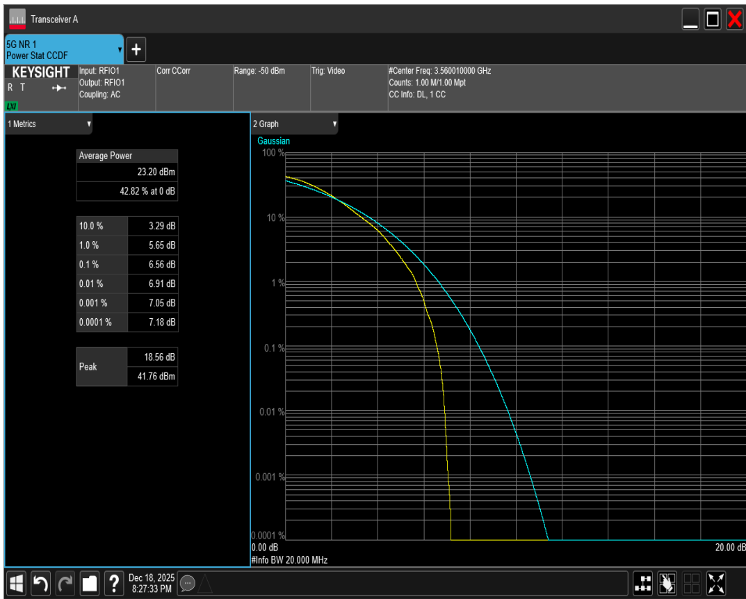
n78(3550-3700) SCS=30kHz DFT_QAM64 BW=20MHz Channel=641666 RB=50@0
