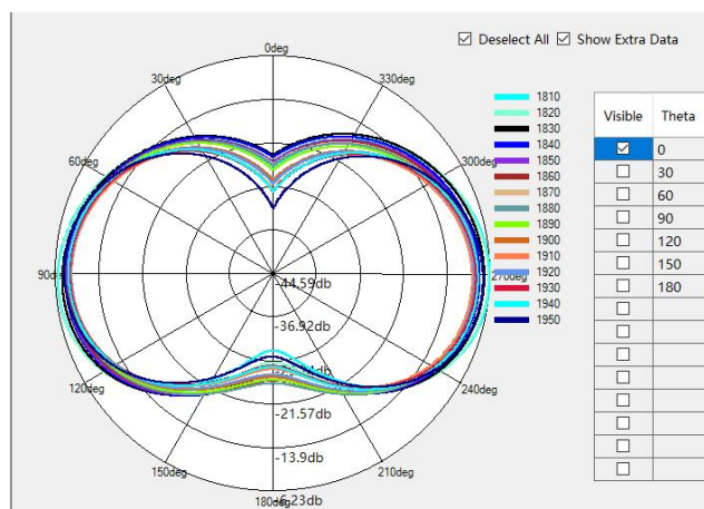
PCS / WCDMA B2 / LTE B2 Phi=0deg
