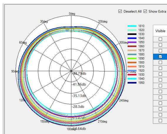
PCS / WCDMA B2 / LTE B2 Theta=90deg
