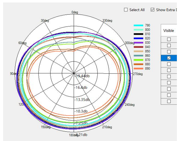
GSM 850 / WCDMA B5 / LTE B5/B20 \Theta=90^\circ
