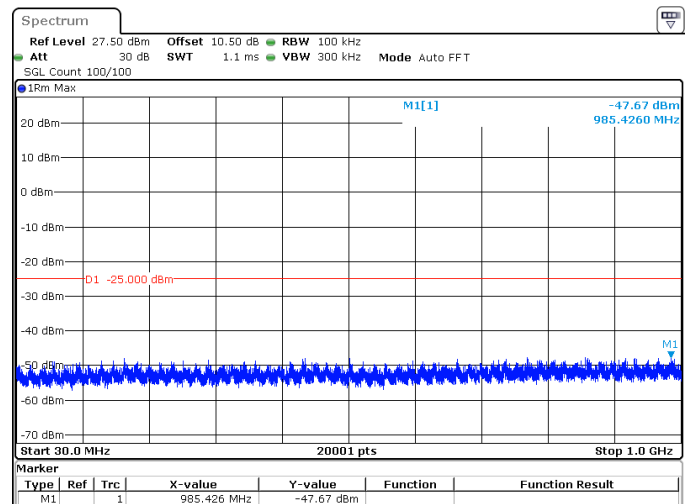
10MHz_30kHz_2615MHz_DFT-s-OFDM QPSK_RB24@0 -47.67 dBm
