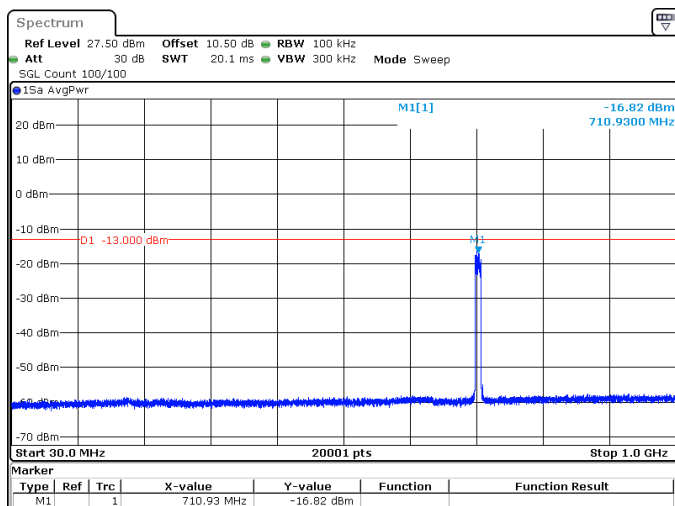
10MHz_15kHz_711MHz_DFT-s-OFDM QPSK_RB50@0 -16.82 dBm
