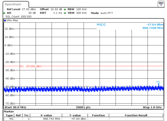
30MHz_30kHz_2595MHz_DFT-s-OFDM QPSK_RB1@77 -47.64 dBm
