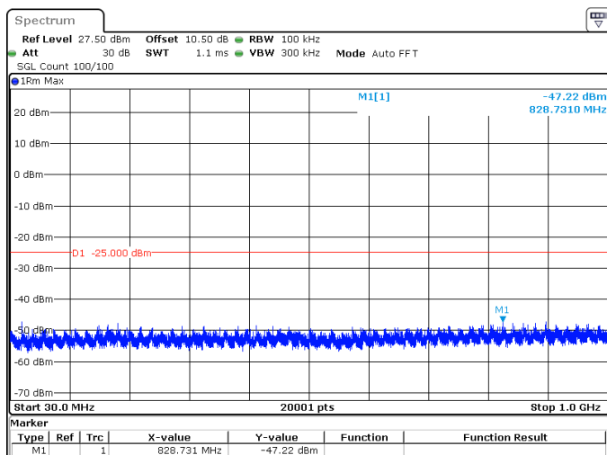
10MHz_30kHz_2595MHz_DFT-s-OFDM QPSK_RB24@0 -47.22 dBm
