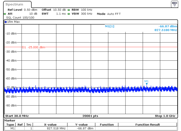
40MHz_30kHz_2590MHz_DFT-s-OFDM QPSK_RB1@0 -66.87 dBm
