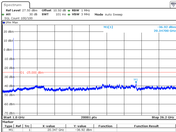
25MHz_30kHz_2595MHz_DFT-s-OFDM QPSK_RB1@0 -36.92 dBm
