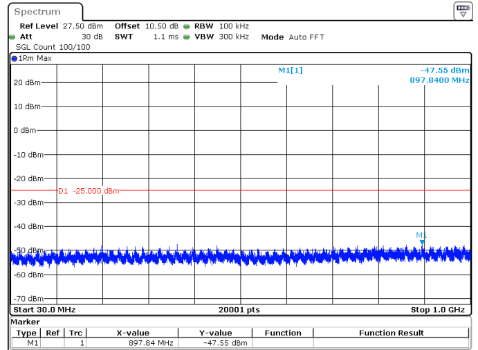
25MHz_30kHz_2582.5MHz_DFT-s-OFDM QPSK_RB1@0 -47.55 dBm
