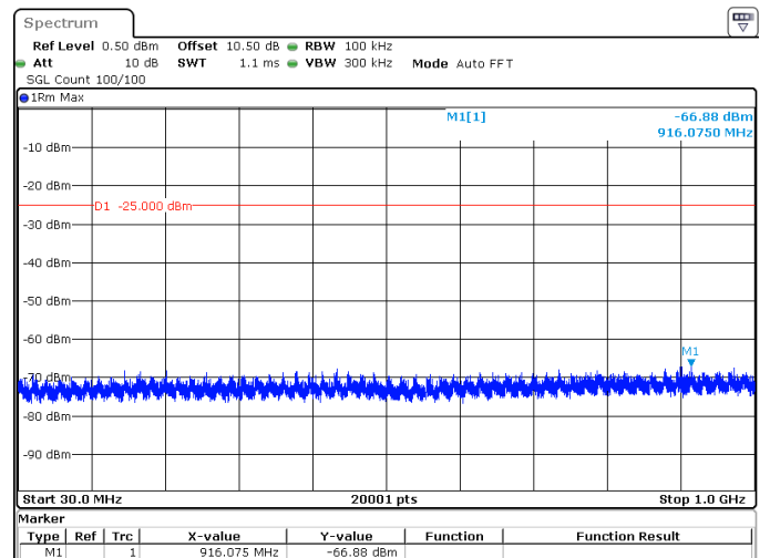
30MHz_30kHz_2605MHz_DFT-s-OFDM QPSK_RB75@0 -66.88 dBm
