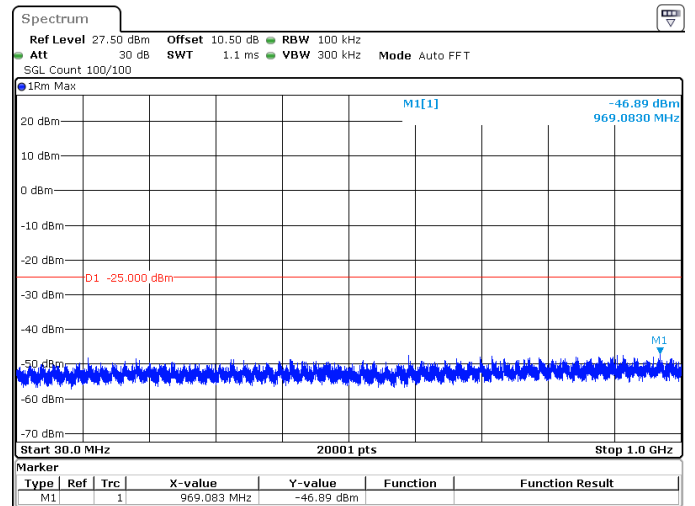
10MHz_30kHz_2575MHz_DFT-s-OFDM QPSK_RB1@0 -46.89 dBm
