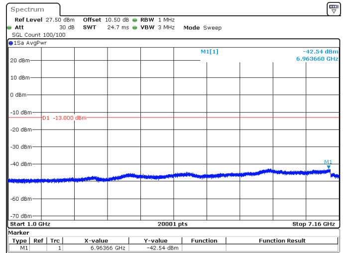
10MHz_15kHz_707.5MHz_DFT-s-OFDM QPSK_RB1@0 -42.54 dBm
