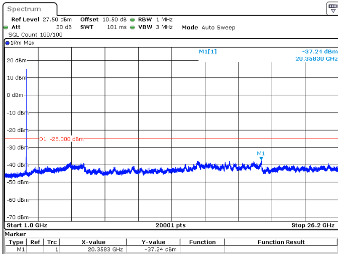
20MHz_30kHz_2610MHz_DFT-s-OFDM QPSK_RB1@50 -37.24 dBm
