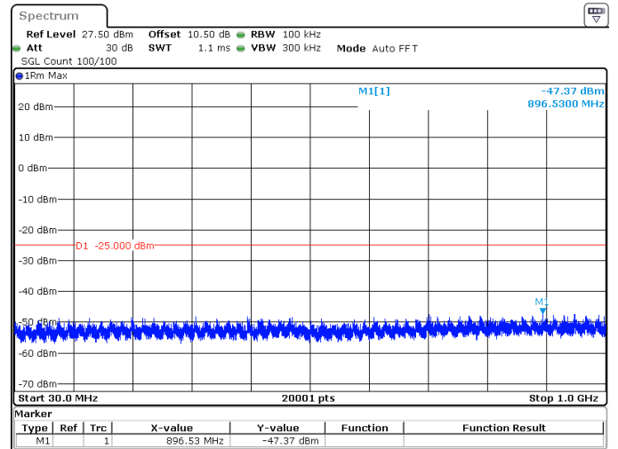
10MHz_30kHz_2615MHz_DFT-s-OFDM QPSK_RB1@23 -47.37 dBm
