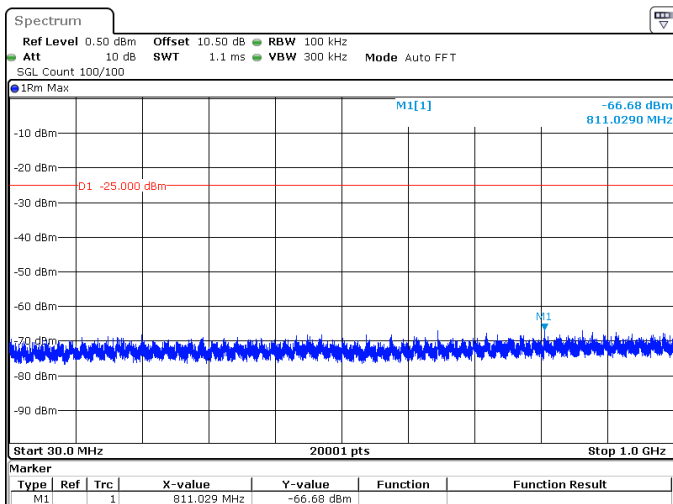
5MHz_15kHz_2617.5MHz_DFT-s-OFDM QPSK_RB25@0 -66.68 dBm
