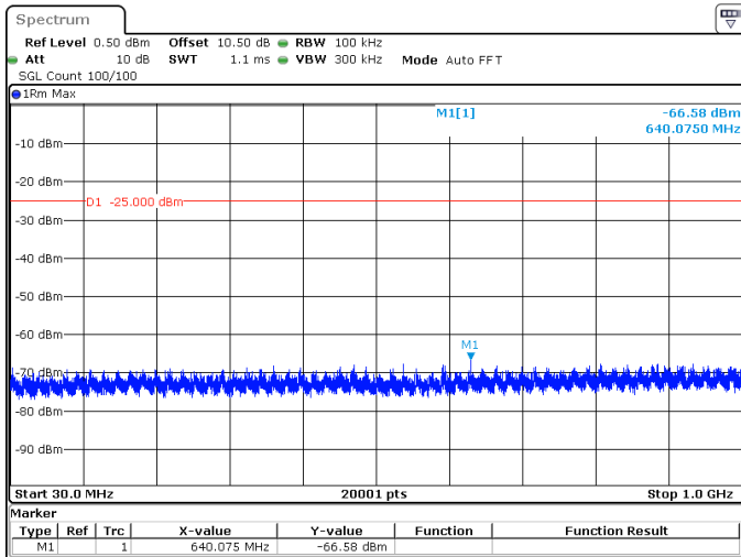
5MHz_15kHz_2617.5MHz_DFT-s-OFDM QPSK_RB1@24 -66.58 dBm
