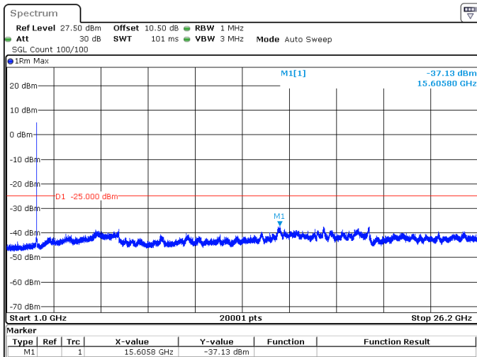
20MHz_30kHz_2595MHz_DFT-s-OFDM QPSK_RB50@0 -37.13 dBm
