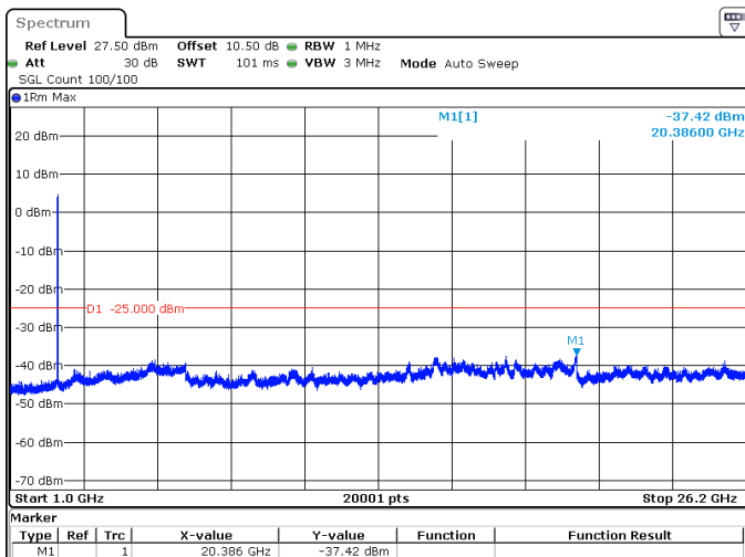
20MHz_30kHz_2610MHz_DFT-s-OFDM QPSK_RB50@0 -37.42 dBm
