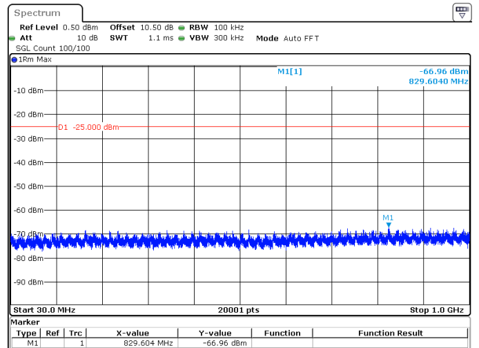
20MHz_30kHz_2595MHz_DFT-s-OFDM QPSK_RB50@0 -66.96 dBm
