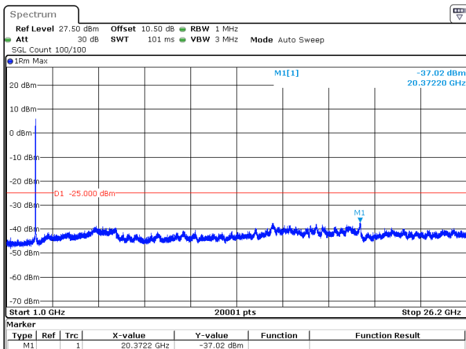
40MHz_30kHz_2590MHz_DFT-s-OFDM QPSK_RB100@0 -37.02 dBm
