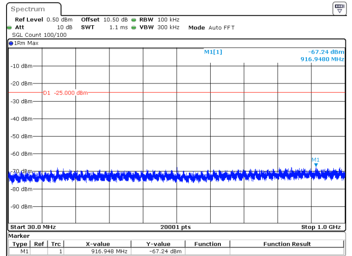
40MHz_30kHz_2590MHz_DFT-s-OFDM QPSK_RB1@105 -67.24 dBm
