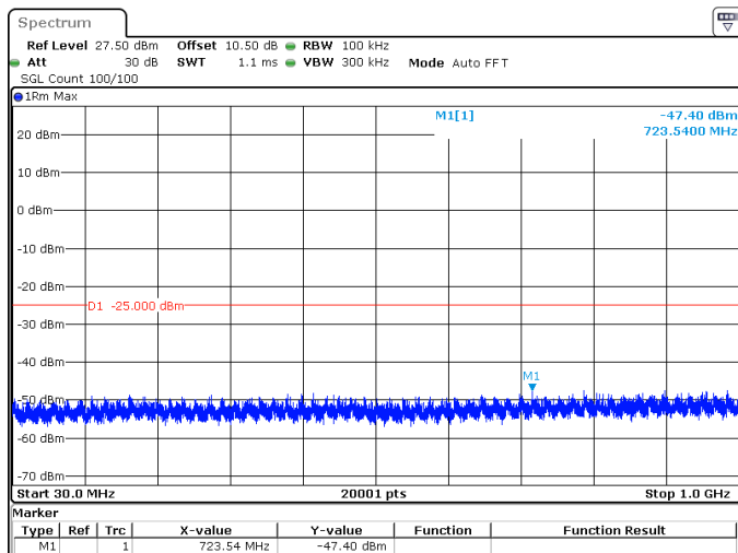
10MHz_30kHz_2575MHz_DFT-s-OFDM QPSK_RB1@23 -47.40 dBm
