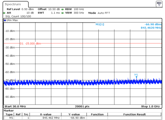
40MHz_30kHz_2600MHz_DFT-s-OFDM QPSK_RB1@105 -66.90 dBm
