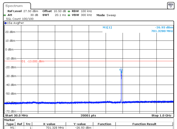
10MHz_15kHz_704MHz_DFT-s-OFDM QPSK_RB50@0 -26.93 dBm
