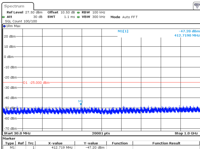
30MHz_30kHz_2585MHz_DFT-s-OFDM QPSK_RB75@0 -47.20 dBm
