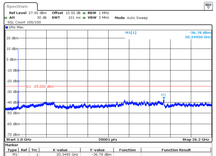
5MHz_15kHz_2595MHz_DFT-s-OFDM QPSK_RB25@0 -36.78 dBm
