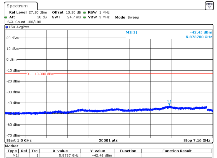
10MHz_15kHz_711MHz_DFT-s-OFDM QPSK_RB1@0 -42.45 dBm
