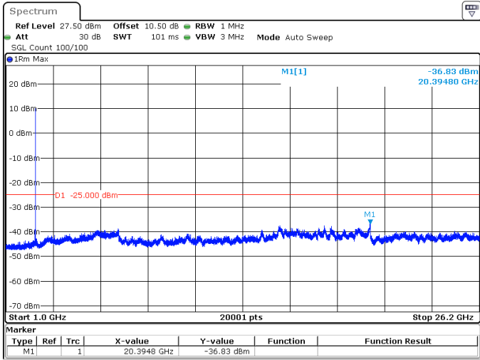
5MHz_15kHz_2572.5MHz_DFT-s-OFDM QPSK_RB25@0 -36.83 dBm
