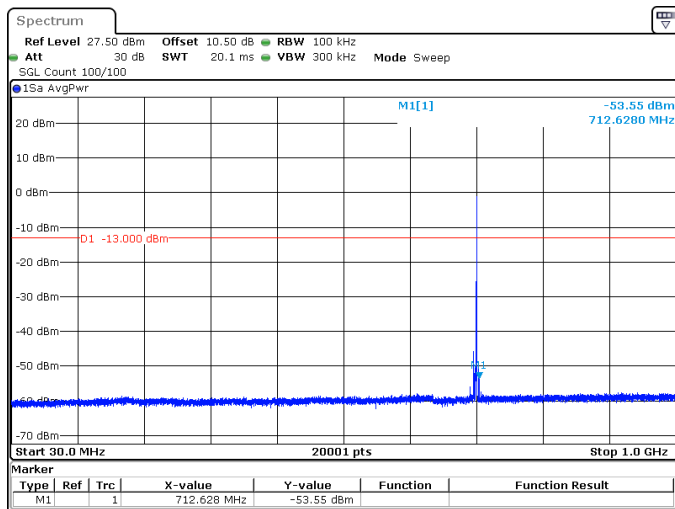
10MHz_15kHz_704MHz_DFT-s-OFDM QPSK_RB1@51 -53.55 dBm
