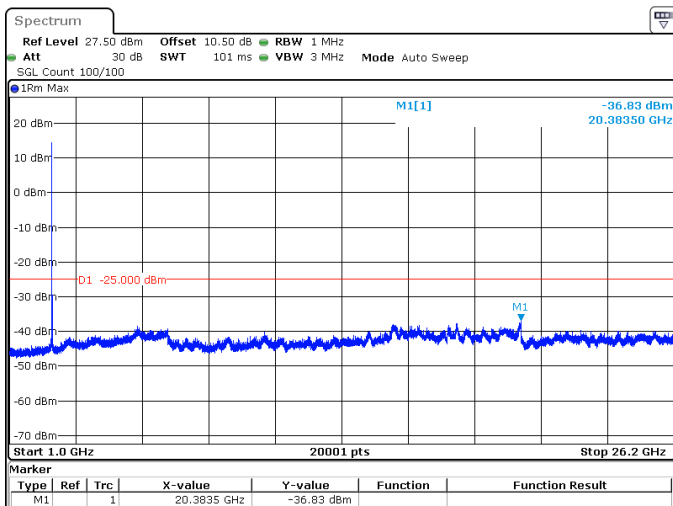
25MHz_30kHz_2595MHz_DFT-s-OFDM QPSK_RB1@64 -36.83 dBm
