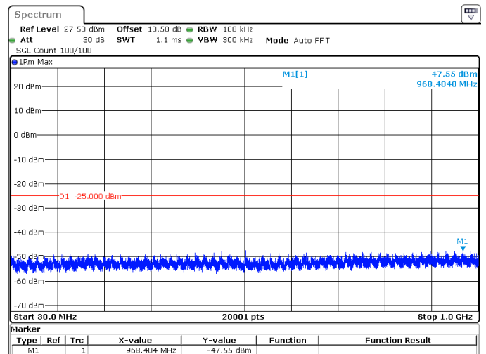
25MHz_30kHz_2582.5MHz_DFT-s-OFDM QPSK_RB64@0 -47.55 dBm
