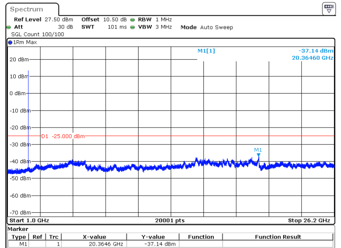
10MHz_30kHz_2595MHz_DFT-s-OFDM QPSK_RB1@0 -37.14 dBm
