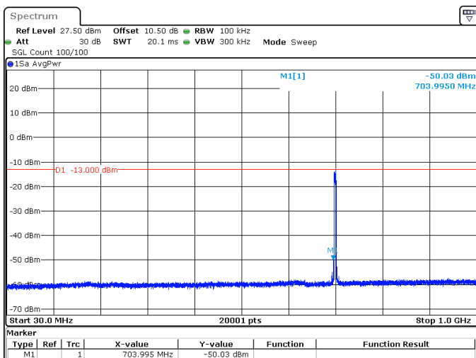
5MHz_15kHz_707.5MHz_DFT-s-OFDM QPSK_RB25@0 -50.03 dBm
