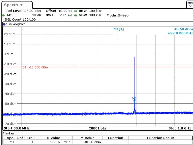
15MHz_15kHz_707.5MHz_DFT-s-OFDM QPSK_RB1@0 -48.58 dBm
