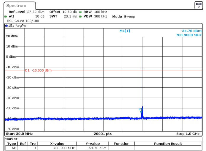
5MHz_15kHz_707.5MHz_DFT-s-OFDM QPSK_RB1@0 -54.78 dBm
