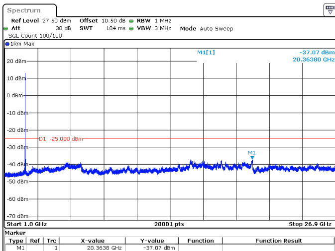
10MHz_15kHz_2593.005MHz_DFT-s-OFDM QPSK_RB1@51 -37.07 dBm
