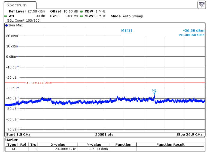
10MHz_15kHz_2685MHz_DFT-s-OFDM QPSK_RB1@0 -36.38 dBm
