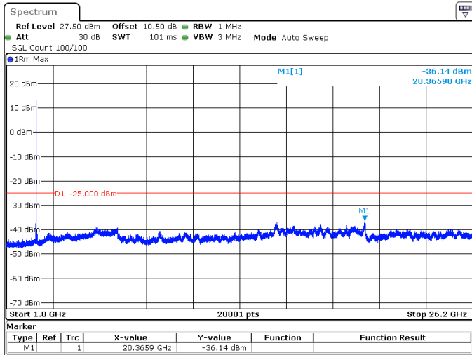
30MHz_30kHz_2605MHz_DFT-s-OFDM QPSK_RB1@0 -36.14 dBm
