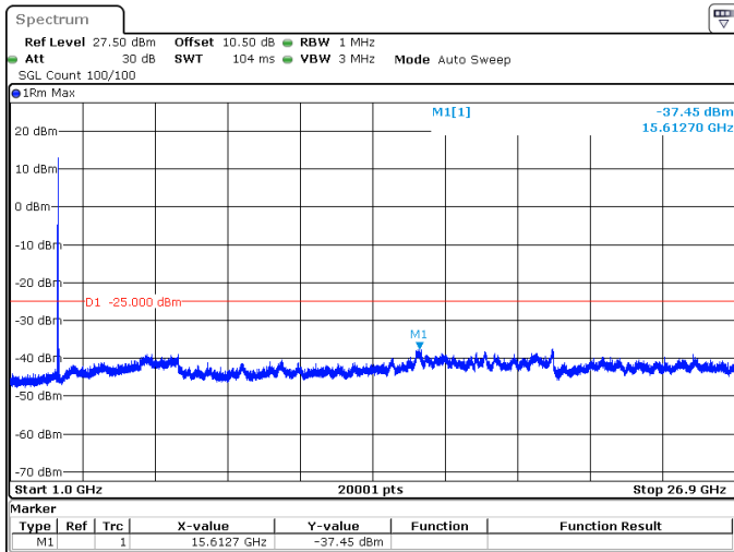
10MHz_15kHz_2685MHz_DFT-s-OFDM QPSK_RB1@51 -37.45 dBm
