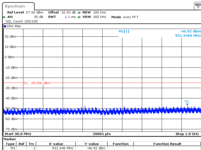
10MHz_30kHz_2501.01MHz_DFT-s-OFDM QPSK_RB1@23 -46.92 dBm
