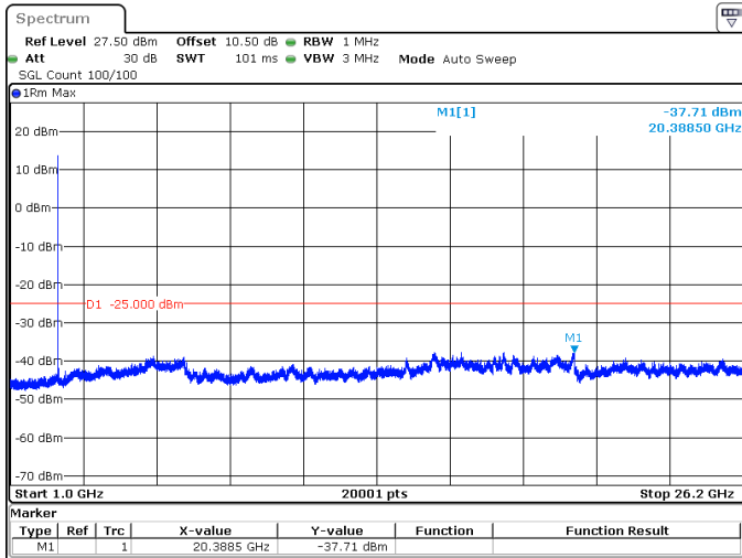
5MHz_15kHz_2617.5MHz_DFT-s-OFDM QPSK_RB1@0 -37.71 dBm
