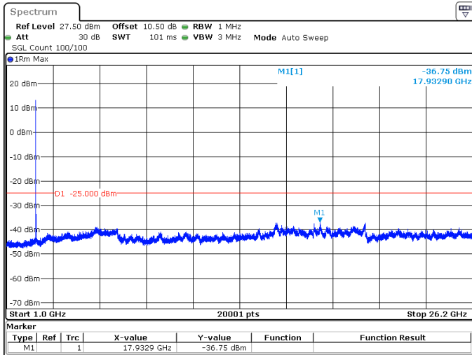
40MHz_30kHz_2590MHz_DFT-s-OFDM QPSK_RB1@0 -36.75 dBm
