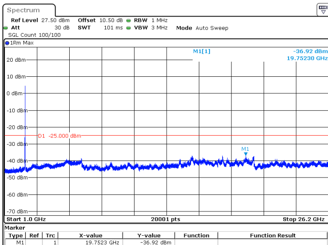
30MHz_30kHz_2595MHz_DFT-s-OFDM QPSK_RB75@0 -36.92 dBm
