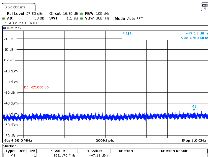
10MHz_15kHz_2593.005MHz_DFT-s-OFDM QPSK_RB50@0 -47.11 dBm
