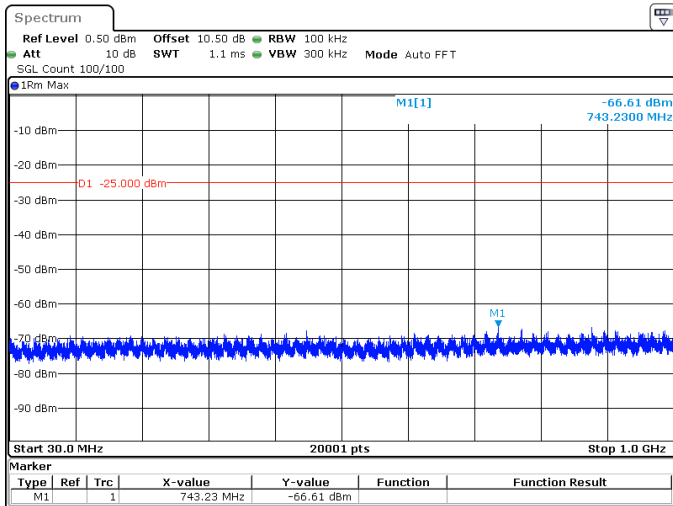
30MHz_30kHz_2585MHz_DFT-s-OFDM QPSK_RB1@77 -66.61 dBm
