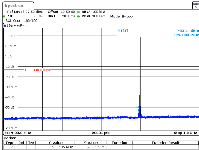
10MHz_15kHz_707.5MHz_DFT-s-OFDM QPSK_RB1@0 -53.24 dBm
