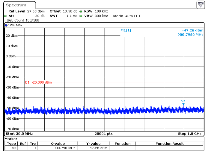
30MHz_30kHz_2585MHz_DFT-s-OFDM QPSK_RB1@0 -47.26 dBm
