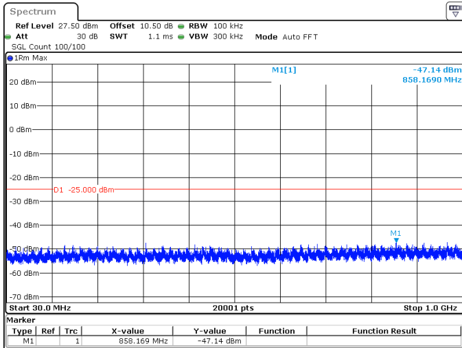
10MHz_15kHz_2685MHz_DFT-s-OFDM QPSK_RB1@0 -47.14 dBm
