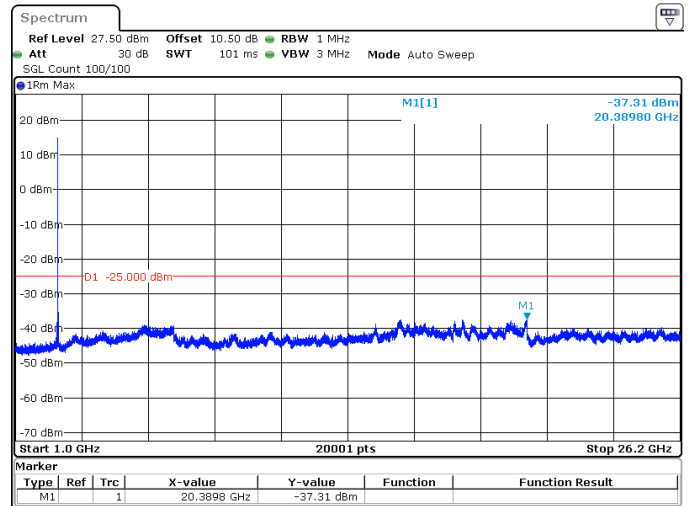
30MHz_30kHz_2585MHz_DFT-s-OFDM QPSK_RB1@77 -37.31 dBm
