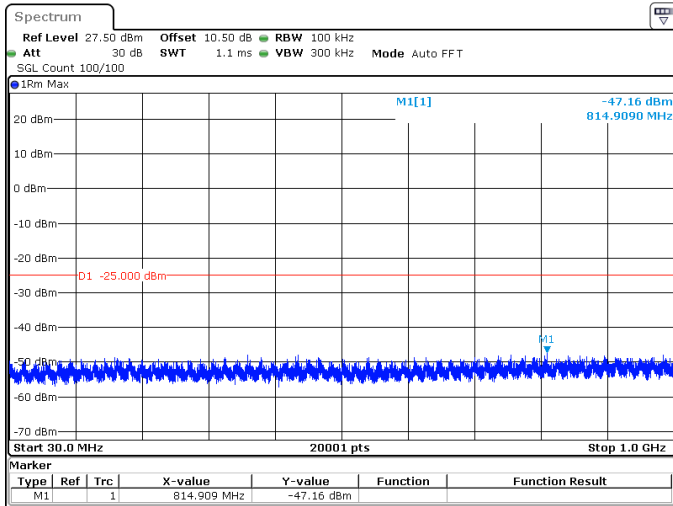
30MHz_30kHz_2595MHz_DFT-s-OFDM QPSK_RB1@0 -47.16 dBm
