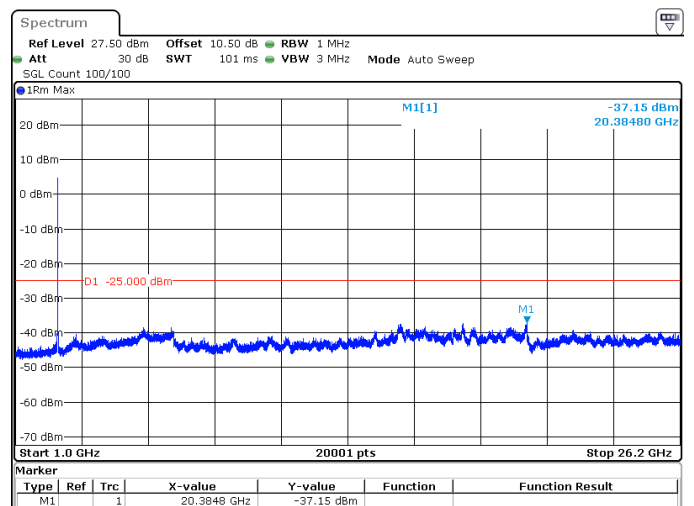
25MHz_30kHz_2595MHz_DFT-s-OFDM QPSK_RB64@0 -37.15 dBm
