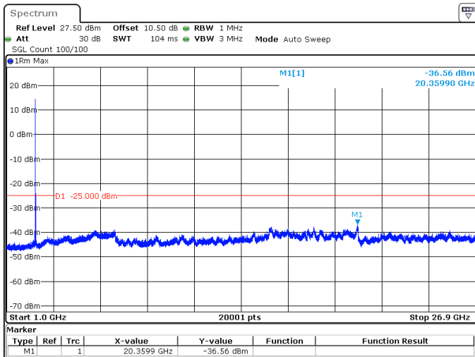
10MHz_15kHz_2593.005MHz_DFT-s-OFDM QPSK_RB1@0 -36.56 dBm
