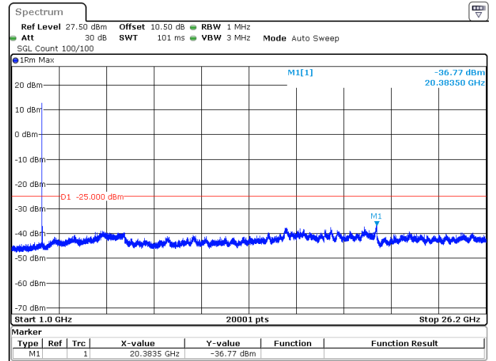
15MHz_30kHz_2612.5MHz_DFT-s-OFDM QPSK_RB1@0 -36.77 dBm
