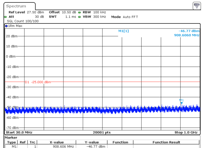
10MHz_15kHz_2685MHz_DFT-s-OFDM QPSK_RB50@0 -46.77 dBm
