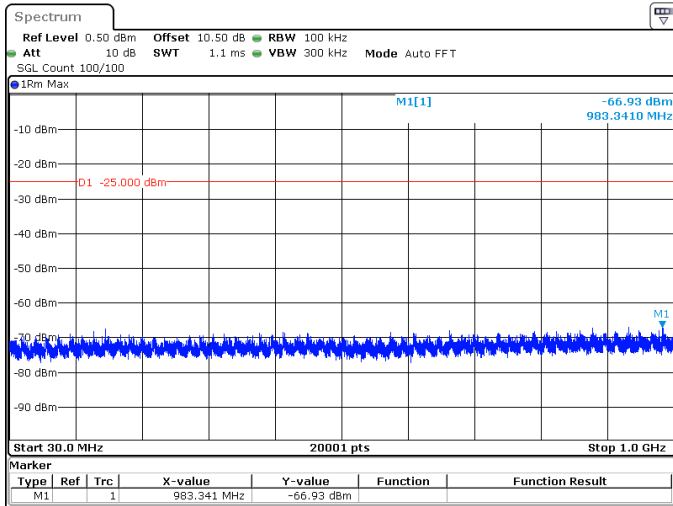
40MHz_30kHz_2595MHz_DFT-s-OFDM QPSK_RB1@0 -66.93 dBm
