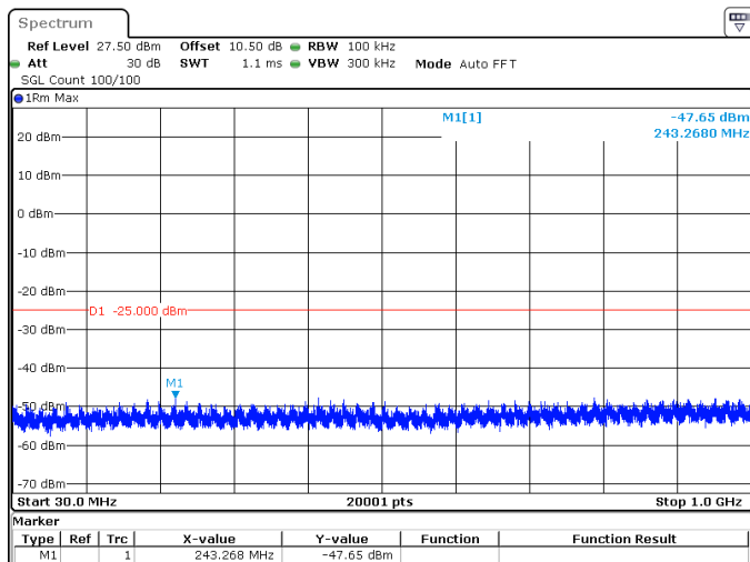
10MHz_30kHz_2595MHz_DFT-s-OFDM QPSK_RB1@23 -47.65 dBm
