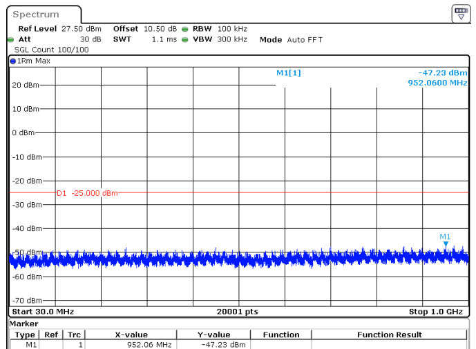
10MHz_15kHz_2593.005MHz_DFT-s-OFDM QPSK_RB1@51 -47.23 dBm
