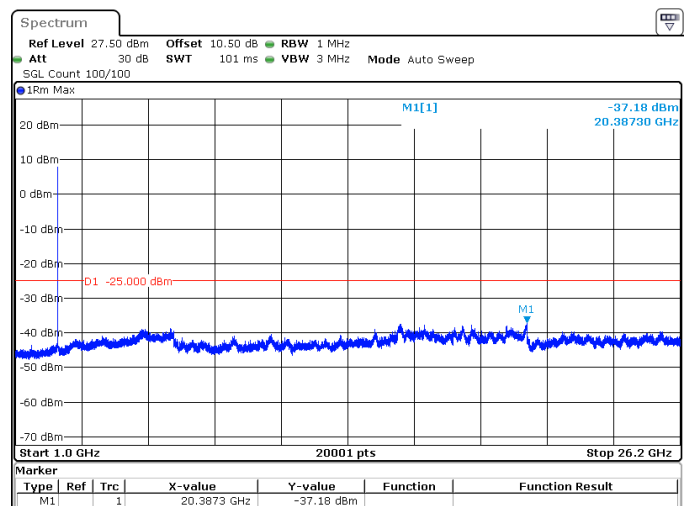
10MHz_30kHz_2595MHz_DFT-s-OFDM QPSK_RB24@0 -37.18 dBm
