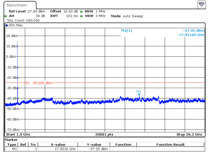
40MHz_30kHz_2595MHz_DFT-s-OFDM QPSK_RB1@0 -37.35 dBm
