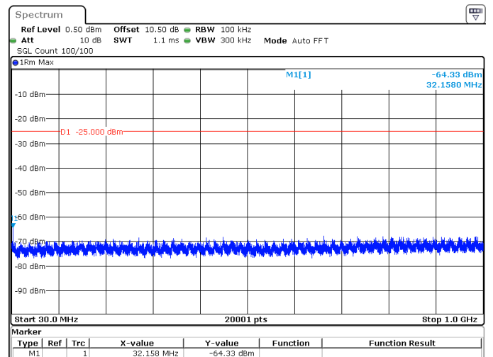
40MHz_30kHz_2590MHz_DFT-s-OFDM QPSK_RB100@0 -64.33 dBm
