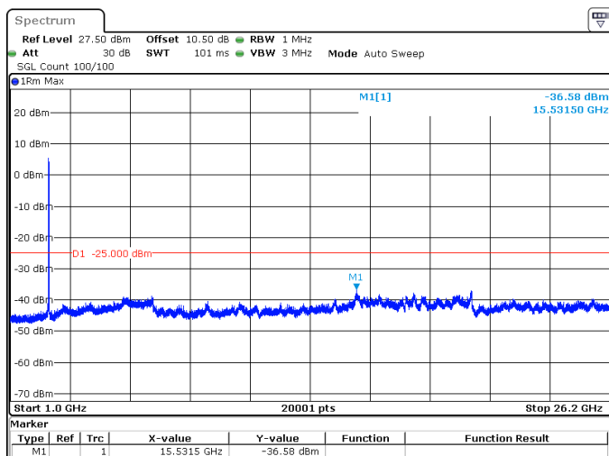
25MHz_30kHz_2607.5MHz_DFT-s-OFDM QPSK_RB64@0 -36.58 dBm
