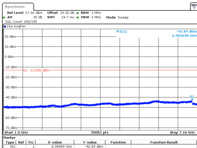
10MHz_15kHz_704MHz_DFT-s-OFDM QPSK_RB50@0 -42.84 dBm
