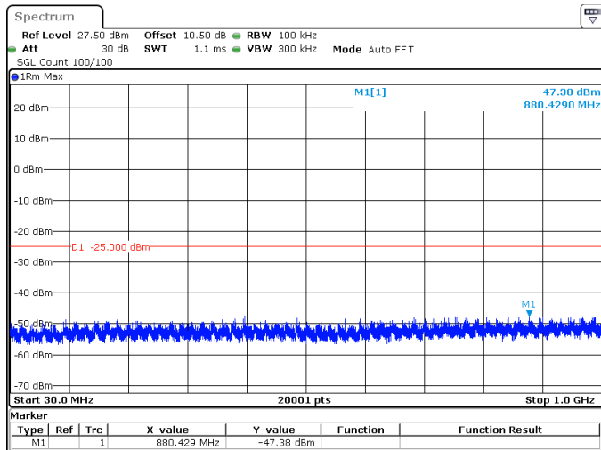
25MHz_30kHz_2607.5MHz_DFT-s-OFDM QPSK_RB1@0 -47.38 dBm
