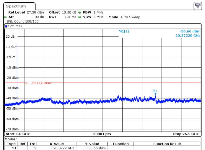
10MHz_30kHz_2595MHz_DFT-s-OFDM QPSK_RB1@23 -36.66 dBm
