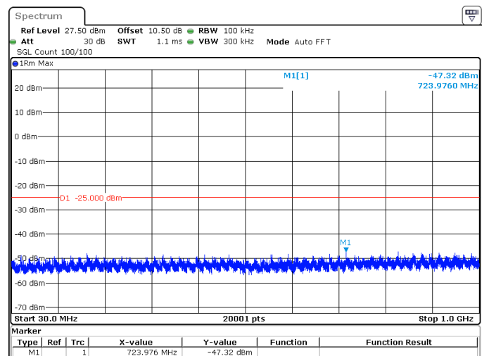
25MHz_30kHz_2607.5MHz_DFT-s-OFDM QPSK_RB64@0 -47.32 dBm
