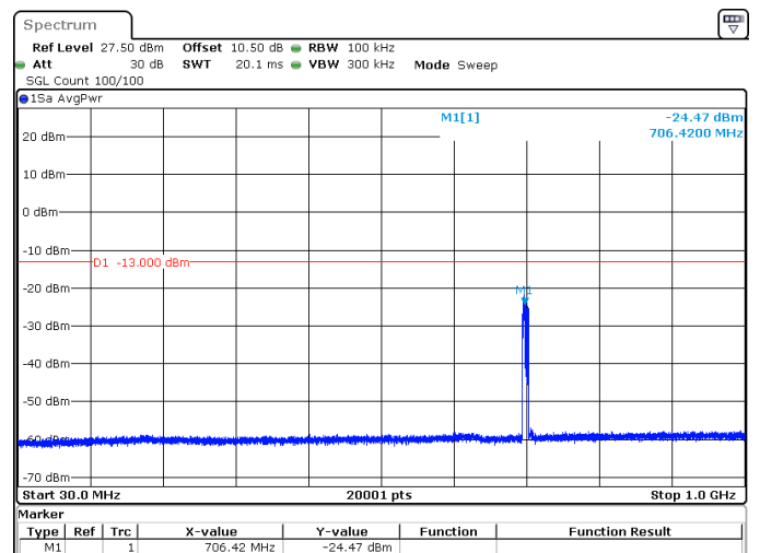
10MHz_15kHz_707.5MHz_DFT-s-OFDM QPSK_RB50@0 -24.47 dBm
