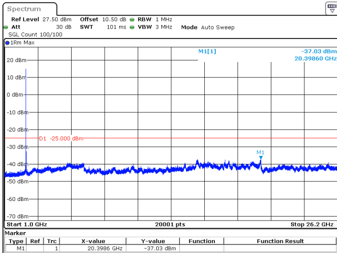
40MHz_30kHz_2590MHz_DFT-s-OFDM QPSK_RB1@105 -37.03 dBm
