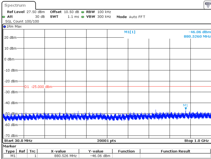
20MHz_30kHz_2610MHz_DFT-s-OFDM QPSK_RB1@0 -46.06 dBm
