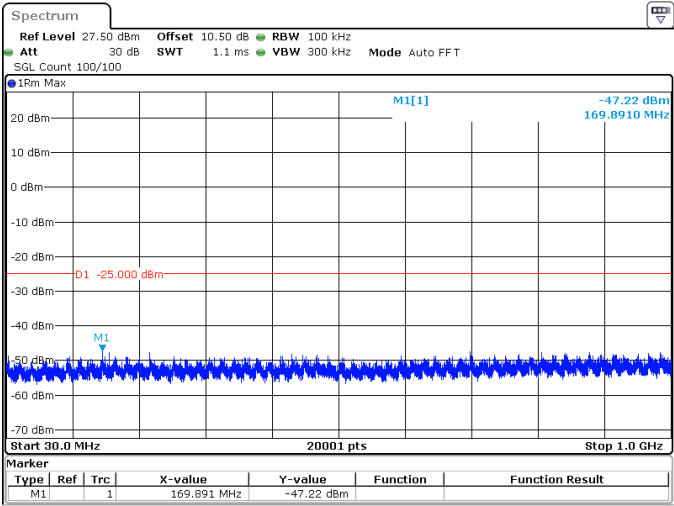
5MHz_15kHz_2572.5MHz_DFT-s-OFDM QPSK_RB25@0 -47.22 dBm
