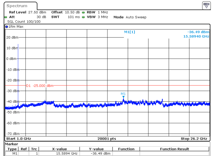
25MHz_30kHz_2607.5MHz_DFT-s-OFDM QPSK_RB1@0 -36.49 dBm
