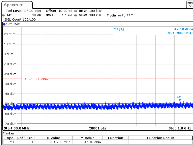
20MHz_30kHz_2580MHz_DFT-s-OFDM QPSK_RB1@0 -47.18 dBm
