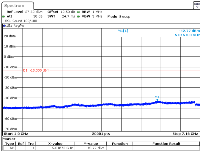
5MHz_15kHz_707.5MHz_DFT-s-OFDM QPSK_RB1@0 -42.77 dBm
