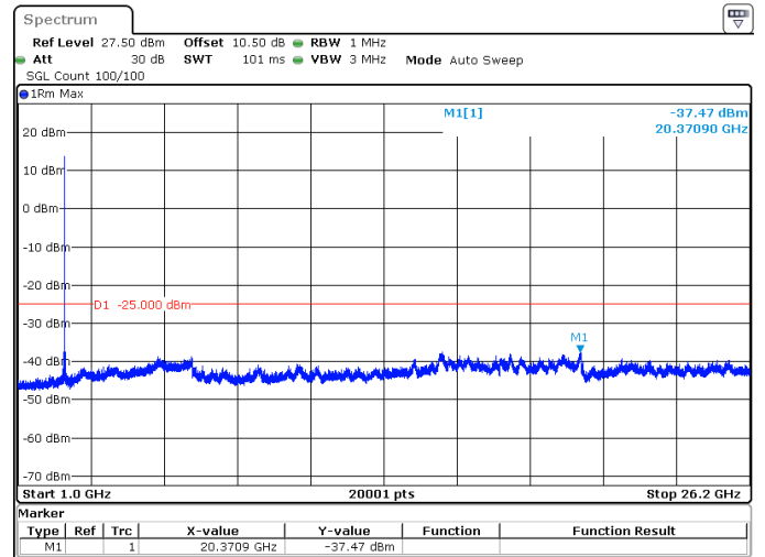
5MHz_15kHz_2595MHz_DFT-s-OFDM QPSK_RB1@24 -37.47 dBm
