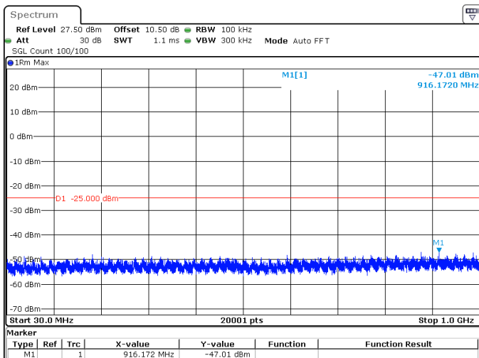
5MHz_15kHz_2595MHz_DFT-s-OFDM QPSK_RB25@0 -47.01 dBm
