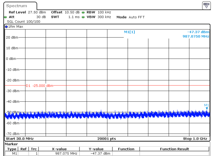
25MHz_30kHz_2595MHz_DFT-s-OFDM QPSK_RB1@0 -47.37 dBm
