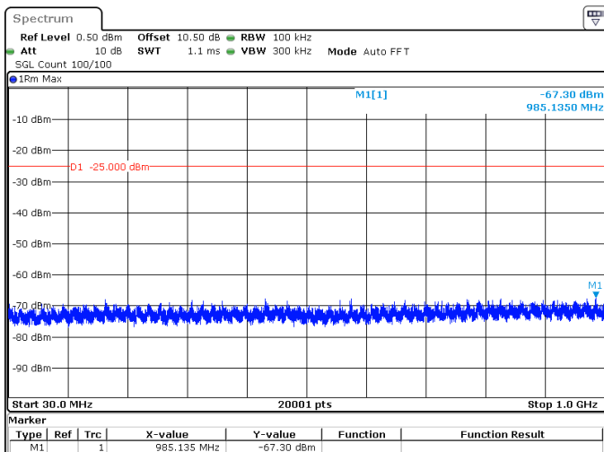
20MHz_30kHz_2580MHz_DFT-s-OFDM QPSK_RB50@0 -67.30 dBm
