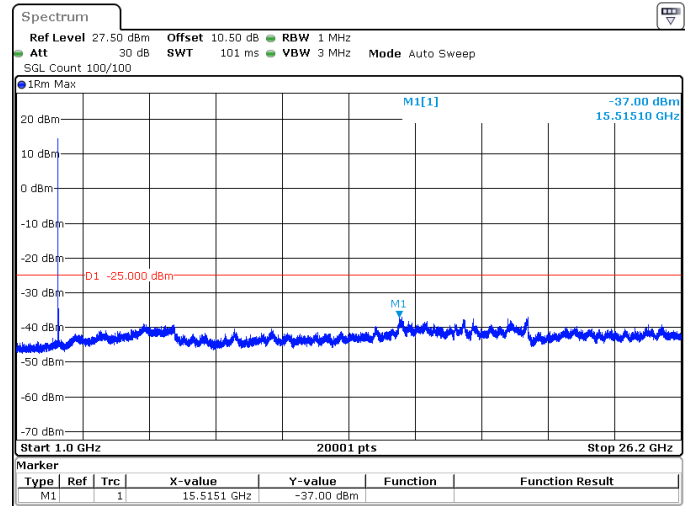
15MHz_30kHz_2577.5MHz_DFT-s-OFDM QPSK_RB1@0 -37.00 dBm
