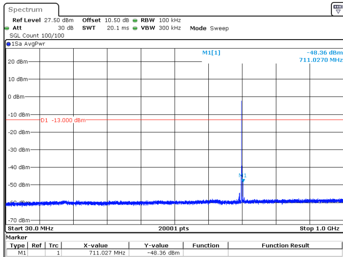
10MHz_15kHz_711MHz_DFT-s-OFDM QPSK_RB1@0 -48.36 dBm
