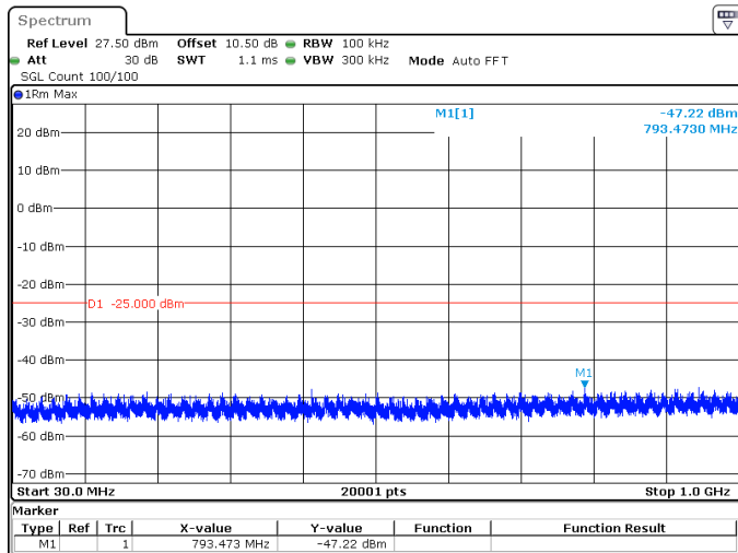
10MHz_30kHz_2595MHz_DFT-s-OFDM QPSK_RB1@0 -47.22 dBm
