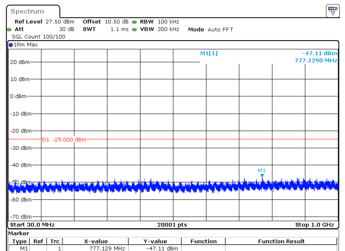
10MHz_30kHz_2501.01MHz_DFT-s-OFDM QPSK_RB24@0 -47.11 dBm
