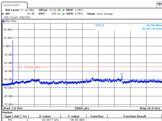
10MHz_15kHz_2685MHz_DFT-s-OFDM QPSK_RB50@0 -36.98 dBm
