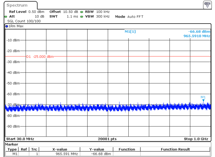
30MHz_30kHz_2605MHz_DFT-s-OFDM QPSK_RB1@0 -66.68 dBm
