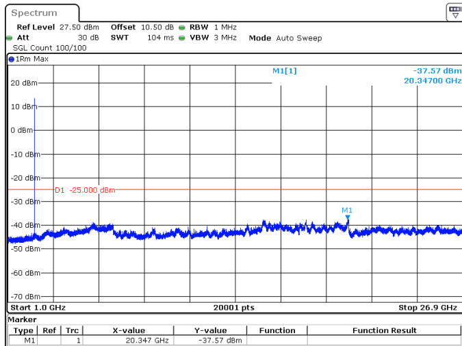
10MHz_30kHz_2501.01MHz_DFT-s-OFDM QPSK_RB1@0 -37.57 dBm
