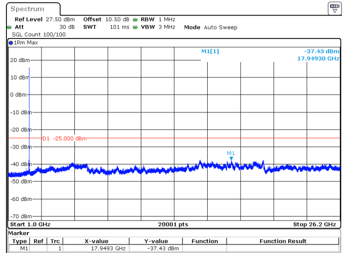
20MHz_30kHz_2580MHz_DFT-s-OFDM QPSK_RB1@50 -37.43 dBm
