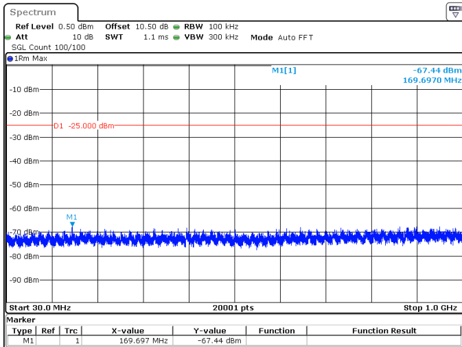
20MHz_30kHz_2580MHz_DFT-s-OFDM QPSK_RB1@50 -67.44 dBm
