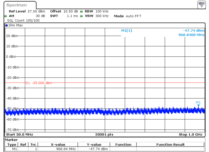
5MHz_15kHz_2617.5MHz_DFT-s-OFDM QPSK_RB1@0 -47.74 dBm
