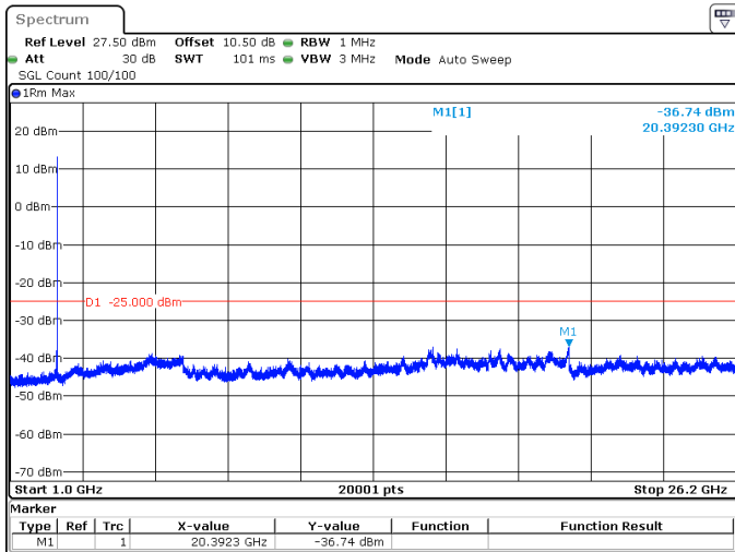
10MHz_30kHz_2615MHz_DFT-s-OFDM QPSK_RB1@23 -36.74 dBm
