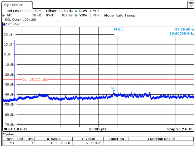
30MHz_30kHz_2585MHz_DFT-s-OFDM QPSK_RB1@0 -37.36 dBm
