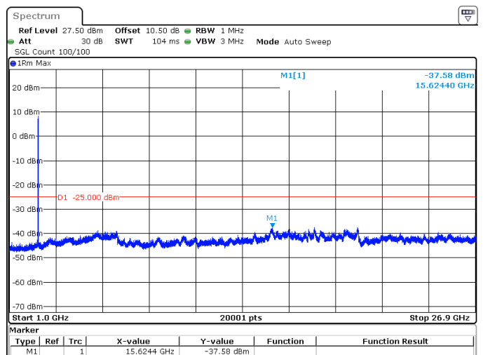
10MHz_15kHz_2593.005MHz_DFT-s-OFDM QPSK_RB50@0 -37.58 dBm
