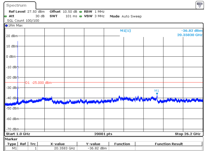
5MHz_15kHz_2617.5MHz_DFT-s-OFDM QPSK_RB1@24 -36.82 dBm
