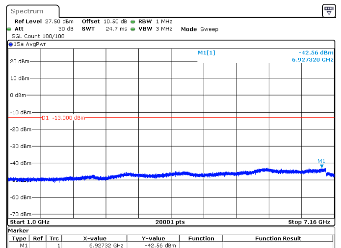
10MHz_15kHz_711MHz_DFT-s-OFDM QPSK_RB50@0 -42.56 dBm
