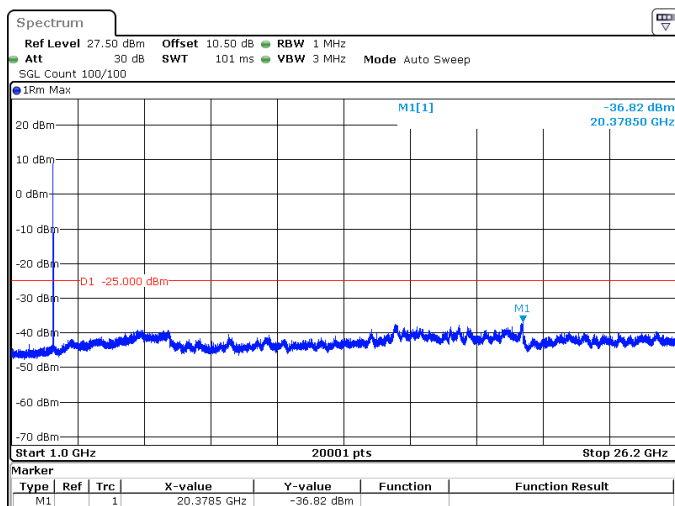
10MHz_30kHz_2575MHz_DFT-s-OFDM QPSK_RB24@0 -36.82 dBm
