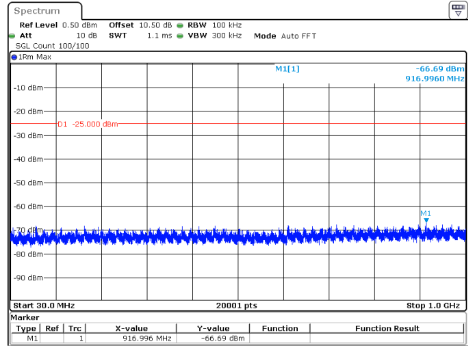
20MHz_30kHz_2595MHz_DFT-s-OFDM QPSK_RB1@50 -66.69 dBm
