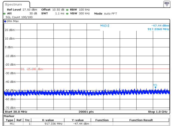
20MHz_30kHz_2610MHz_DFT-s-OFDM QPSK_RB1@50 -47.44 dBm
