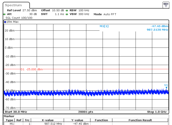
20MHz_30kHz_2610MHz_DFT-s-OFDM QPSK_RB50@0 -47.45 dBm
