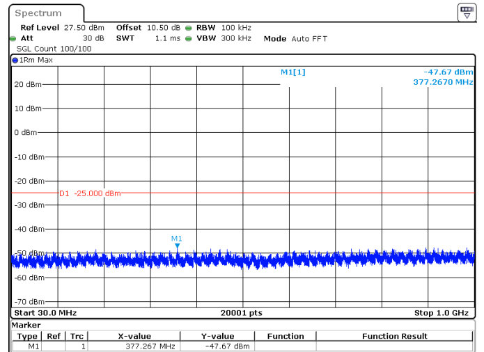
10MHz_30kHz_2501.01MHz_DFT-s-OFDM QPSK_RB1@0 -47.67 dBm
