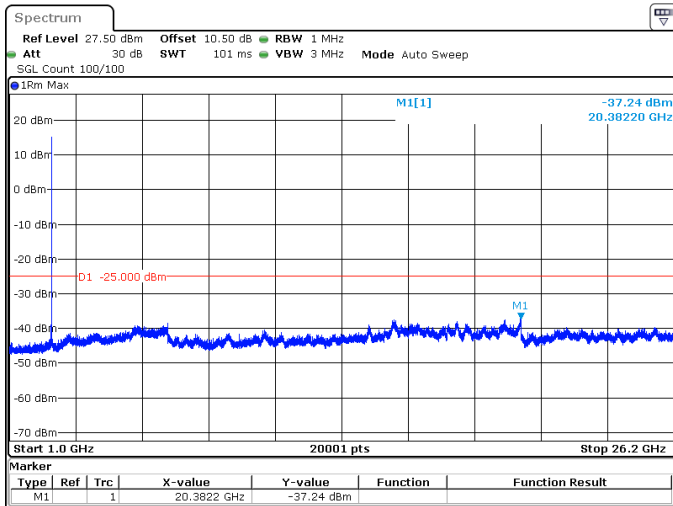
25MHz_30kHz_2582.5MHz_DFT-s-OFDM QPSK_RB1@64 -37.24 dBm
