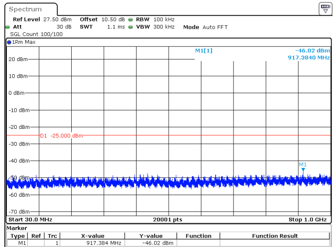
10MHz_15kHz_2593.005MHz_DFT-s-OFDM QPSK_RB1@0 -46.02 dBm
