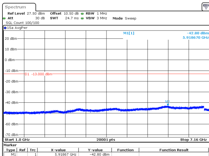
10MHz_15kHz_707.5MHz_DFT-s-OFDM QPSK_RB50@0 -42.80 dBm
