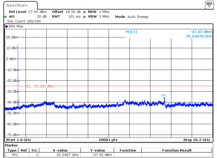
20MHz_30kHz_2610MHz_DFT-s-OFDM QPSK_RB1@0 -37.52 dBm
