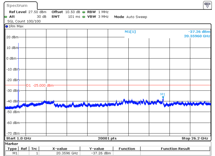
30MHz_30kHz_2605MHz_DFT-s-OFDM QPSK_RB1@77 -37.26 dBm
