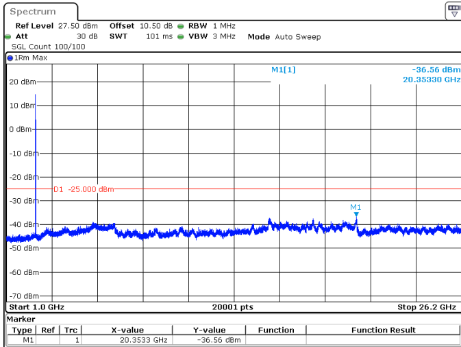
10MHz_30kHz_2615MHz_DFT-s-OFDM QPSK_RB1@0 -36.56 dBm
