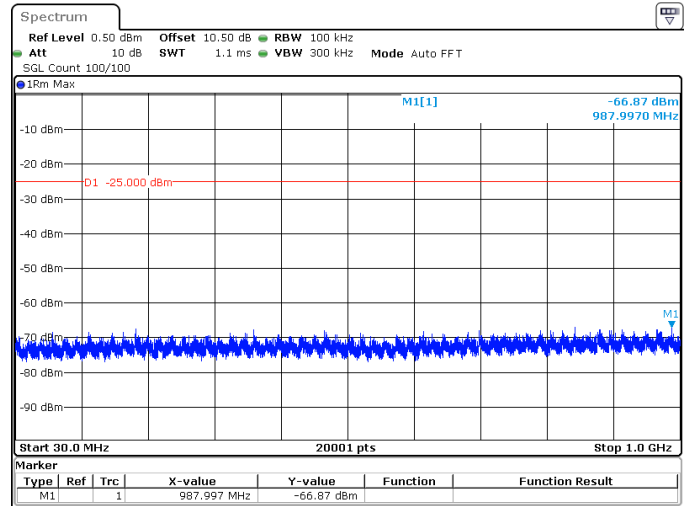
40MHz_30kHz_2600MHz_DFT-s-OFDM QPSK_RB1@0 -66.87 dBm
