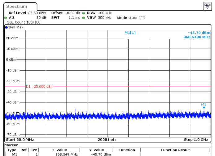
30MHz_30kHz_2595MHz_DFT-s-OFDM QPSK_RB75@0 -45.70 dBm
