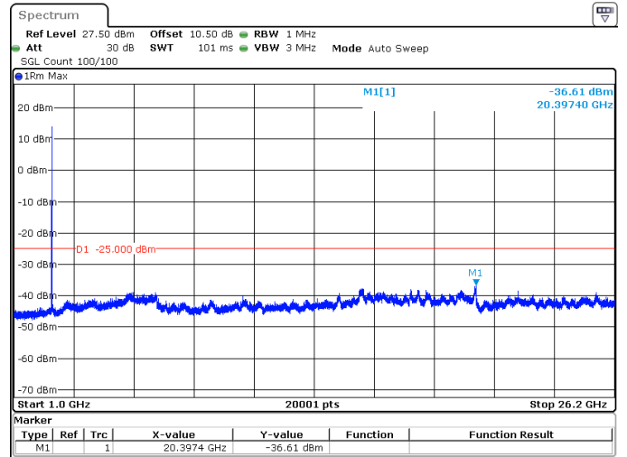
30MHz_30kHz_2595MHz_DFT-s-OFDM QPSK_RB1@0 -36.61 dBm
