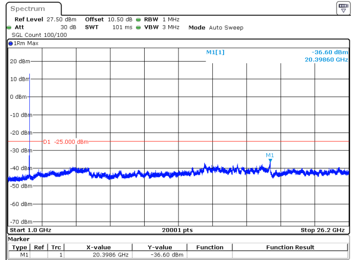
20MHz_30kHz_2595MHz_DFT-s-OFDM QPSK_RB1@0 -36.60 dBm
