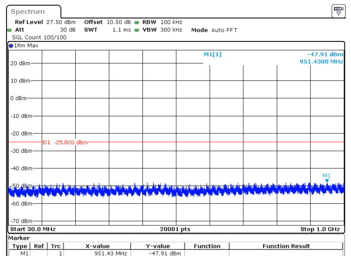
10MHz_30kHz_2575MHz_DFT-s-OFDM QPSK_RB24@0 -47.91 dBm
