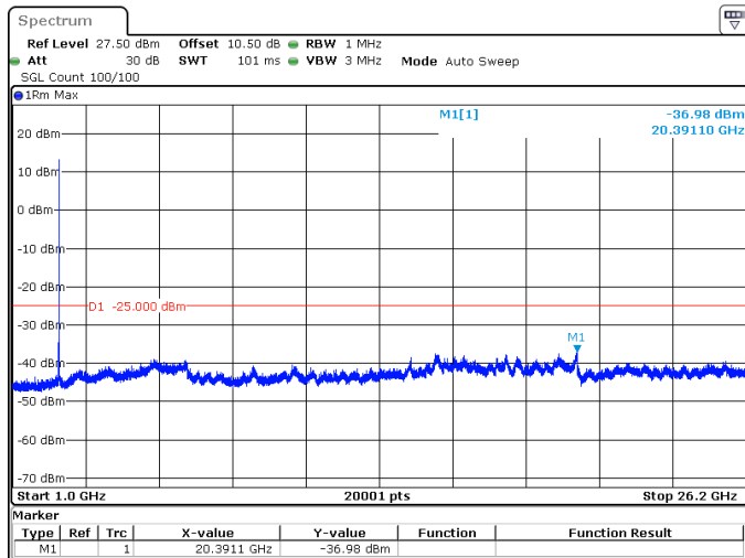
15MHz_30kHz_2595MHz_DFT-s-OFDM QPSK_RB1@0 -36.98 dBm
