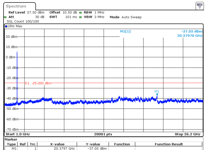
30MHz_30kHz_2585MHz_DFT-s-OFDM QPSK_RB75@0 -37.05 dBm
