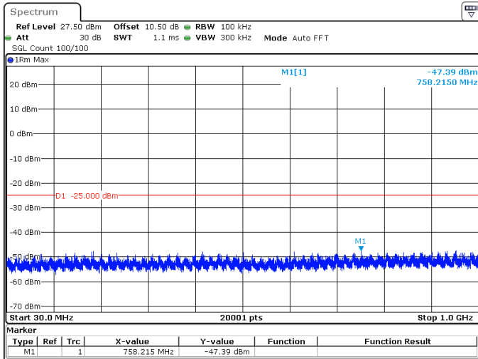
5MHz_15kHz_2595MHz_DFT-s-OFDM QPSK_RB1@0 -47.39 dBm
