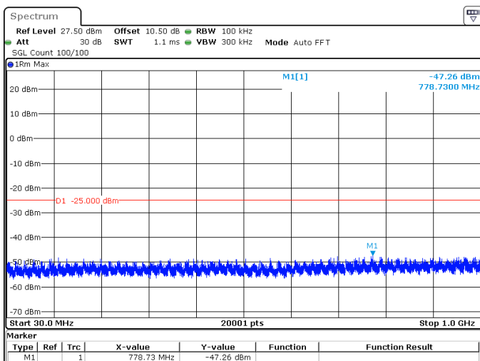
25MHz_30kHz_2595MHz_DFT-s-OFDM QPSK_RB64@0 -47.26 dBm
