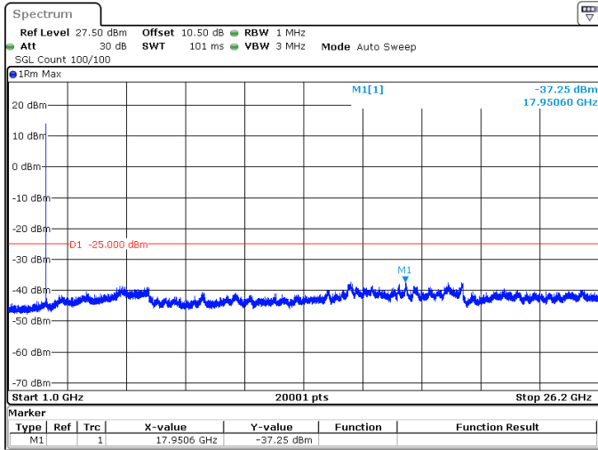
20MHz_30kHz_2595MHz_DFT-s-OFDM QPSK_RB1@50 -37.25 dBm
