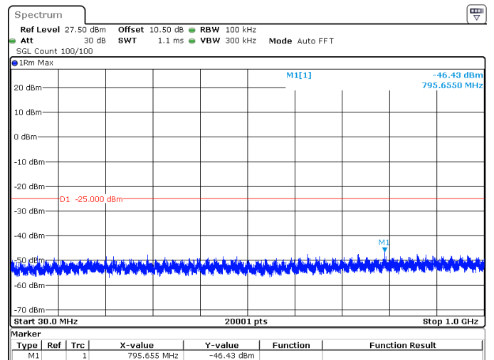
25MHz_30kHz_2595MHz_DFT-s-OFDM QPSK_RB1@64 -46.43 dBm
