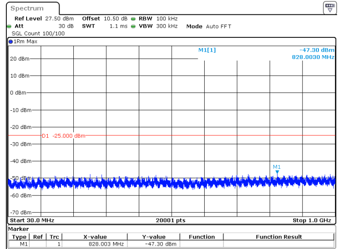
10MHz_30kHz_2615MHz_DFT-s-OFDM QPSK_RB1@0 -47.30 dBm
