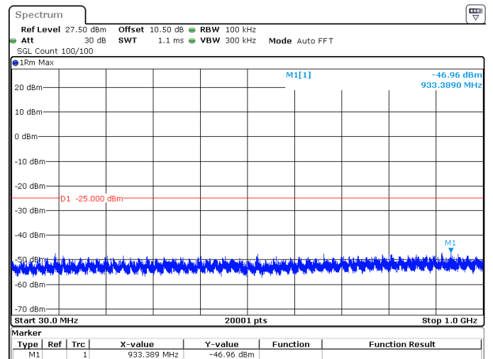
25MHz_30kHz_2607.5MHz_DFT-s-OFDM QPSK_RB1@64 -46.96 dBm
