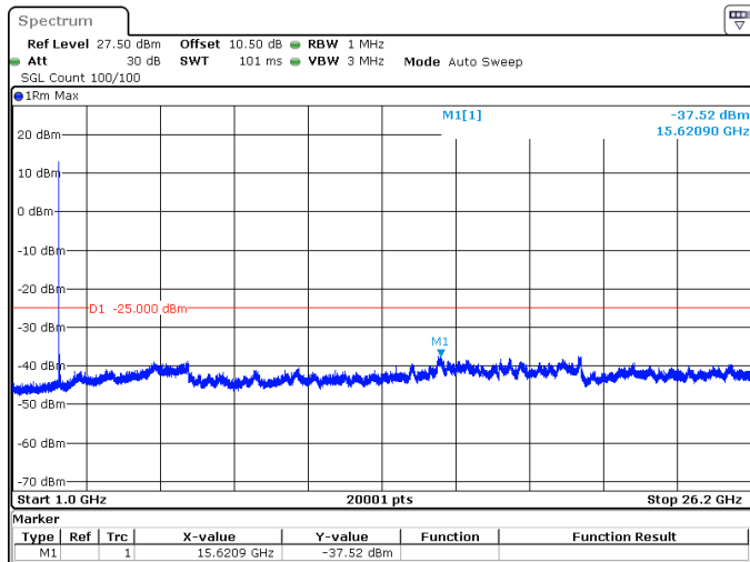
10MHz_30kHz_2575MHz_DFT-s-OFDM QPSK_RB1@0 -37.52 dBm
