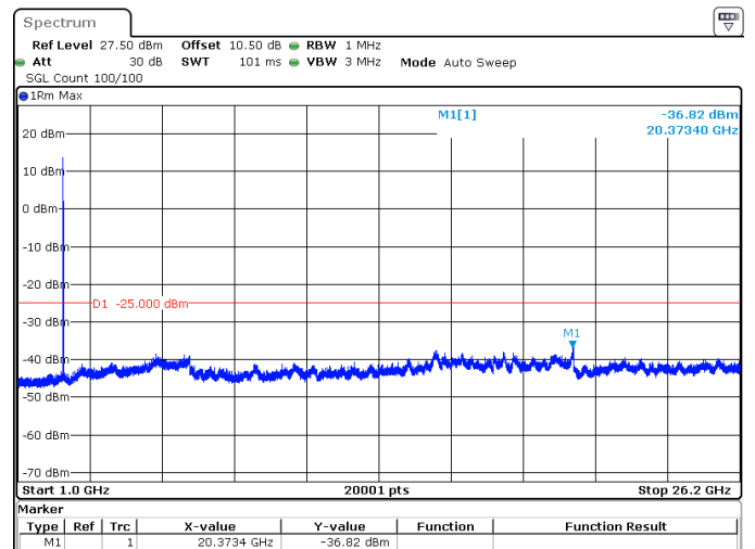
10MHz_30kHz_2575MHz_DFT-s-OFDM QPSK_RB1@23 -36.82 dBm
