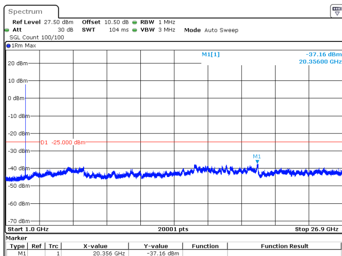
10MHz_30kHz_2501.01MHz_DFT-s-OFDM QPSK_RB24@0 -37.16 dBm
