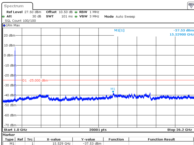
10MHz_30kHz_2615MHz_DFT-s-OFDM QPSK_RB24@0 -37.53 dBm
