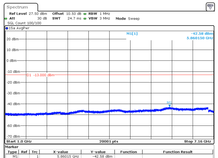
5MHz_15kHz_707.5MHz_DFT-s-OFDM QPSK_RB25@0 -42.58 dBm
