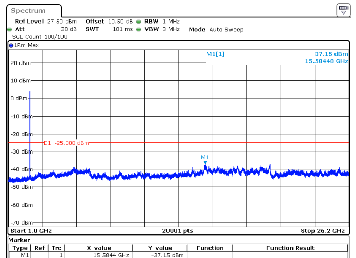
20MHz_30kHz_2580MHz_DFT-s-OFDM QPSK_RB50@0 -37.15 dBm
