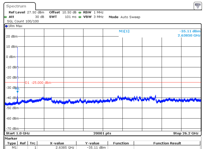
5MHz_15kHz_2617.5MHz_DFT-s-OFDM QPSK_RB25@0 -35.11 dBm
