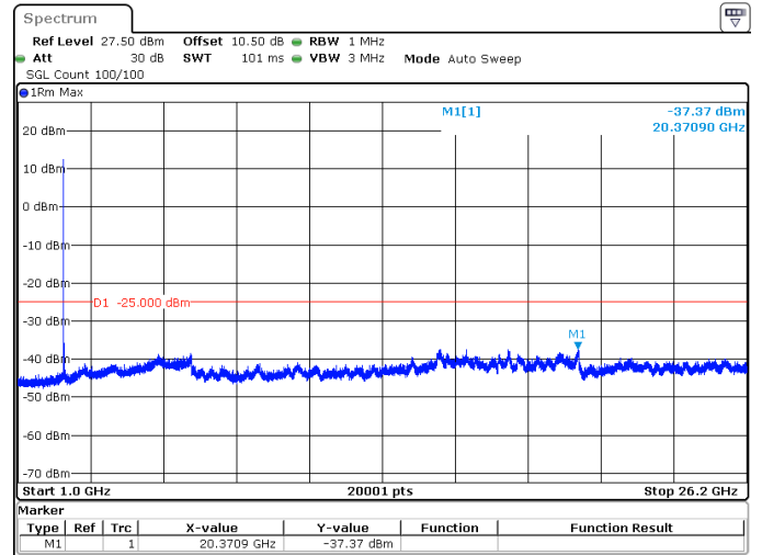
20MHz_30kHz_2580MHz_DFT-s-OFDM QPSK_RB1@0 -37.37 dBm
