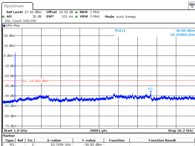
40MHz_30kHz_2600MHz_DFT-s-OFDM QPSK_RB100@0 -36.80 dBm
