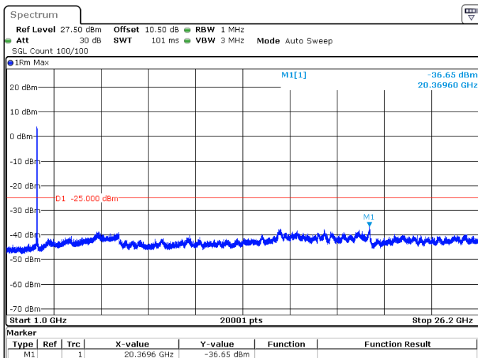
30MHz_30kHz_2605MHz_DFT-s-OFDM QPSK_RB75@0 -36.65 dBm
