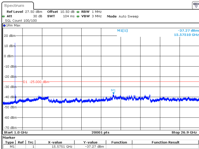
80MHz_30kHz_2649.99MHz_DFT-s-OFDM QPSK_RB1@0 -37.27 dBm
