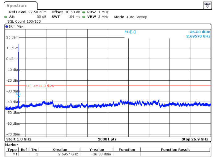
100MHz_30kHz_2640MHz_DFT-s-OFDM QPSK_RB1@272 -36.38 dBm
