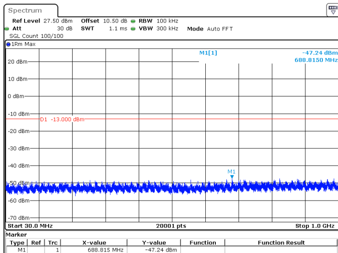
40MHz_15kHz_1760MHz_DFT-s-OFDM QPSK_RB1@215 -47.24 dBm
