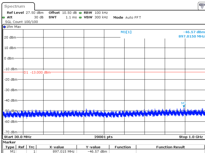
10MHz_15kHz_1745MHz_DFT-s-OFDM QPSK_RB50@0 -46.57 dBm
