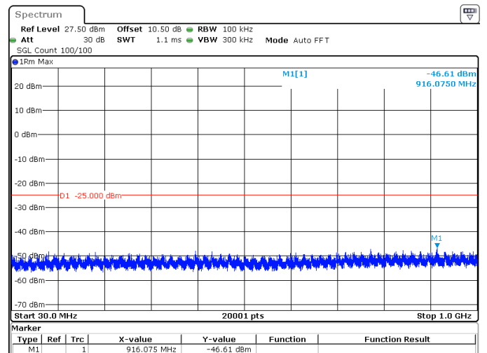
90MHz_30kHz_2541MHz_DFT-s-OFDM QPSK_RB243@0 -46.61 dBm
