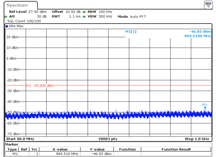
90MHz_30kHz_2541MHz_DFT-s-OFDM QPSK_RB1@0 -46.83 dBm
