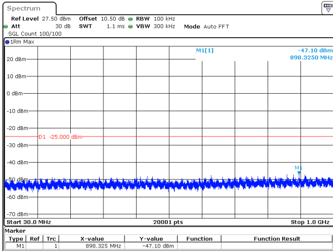
10MHz_15kHz_2535MHz_DFT-s-OFDM QPSK_RB1@0 -47.10 dBm
