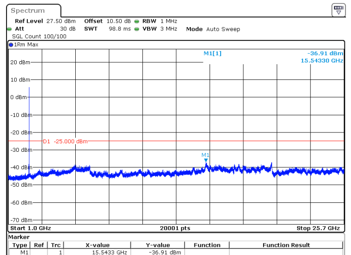
10MHz_15kHz_2535MHz_DFT-s-OFDM QPSK_RB50@0 -36.91 dBm
