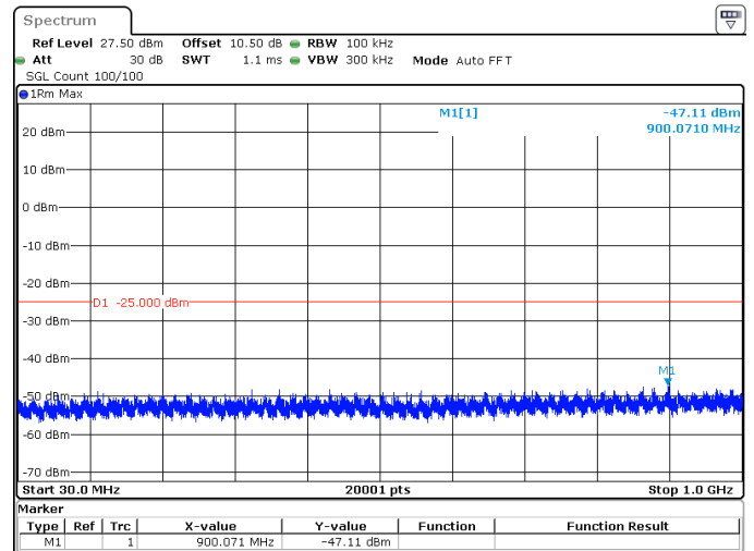
80MHz_30kHz_2649.99MHz_DFT-s-OFDM QPSK_RB1@0 -47.11 dBm
