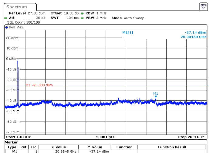
80MHz_30kHz_2649.99MHz_DFT-s-OFDM QPSK_RB216@0 -37.14 dBm
