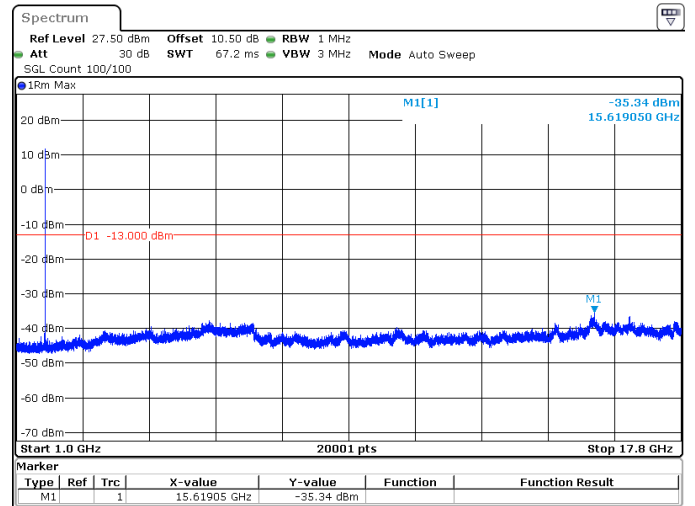
20MHz_15kHz_1720MHz_DFT-s-OFDM QPSK_RB1@105 -35.34 dBm
