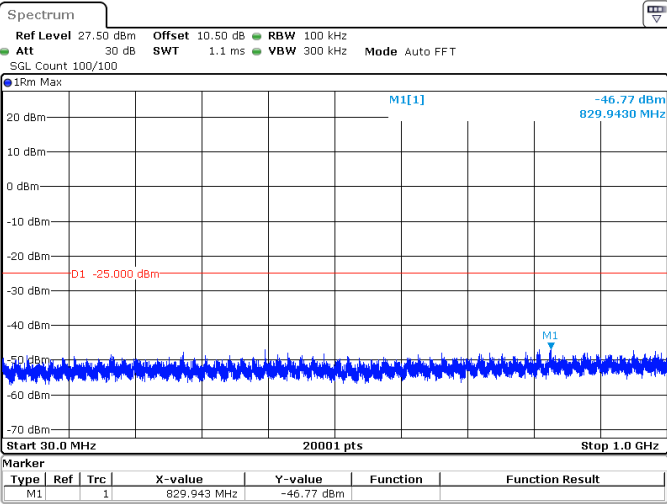
100MHz_30kHz_2592.99MHz_DFT-s-OFDM QPSK_RB1@0 -46.77 dBm
