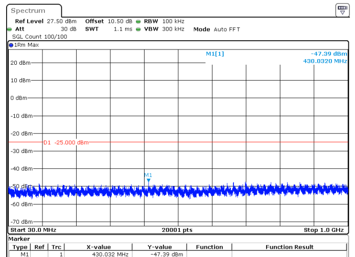
100MHz_30kHz_2640MHz_DFT-s-OFDM QPSK_RB270@0 -47.39 dBm
