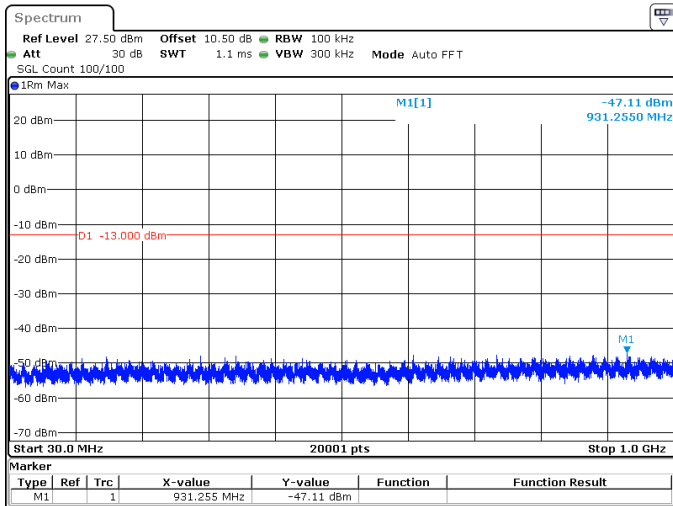
20MHz_15kHz_1720MHz_DFT-s-OFDM QPSK_RB1@105 -47.11 dBm
