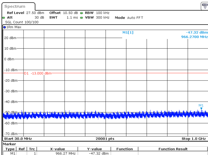
20MHz_15kHz_1720MHz_DFT-s-OFDM QPSK_RB100@0 -47.32 dBm
