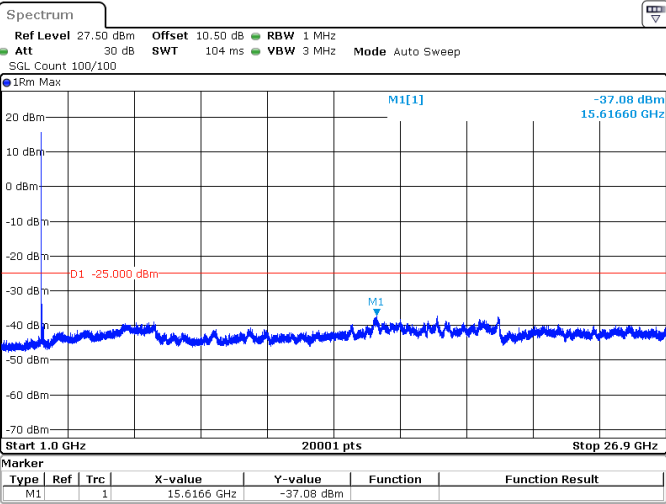
100MHz_30kHz_2592.99MHz_DFT-s-OFDM QPSK_RB1@0 -37.08 dBm
