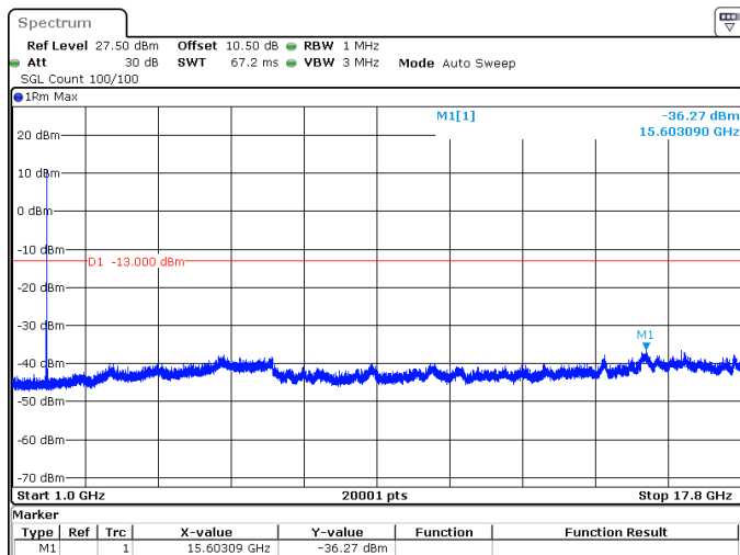
5MHz_15kHz_1777.5MHz_DFT-s-OFDM QPSK_RB1@24 -36.27 dBm
