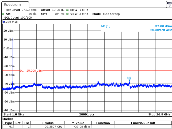
90MHz_30kHz_2541MHz_DFT-s-OFDM QPSK_RB1@244 -37.08 dBm
