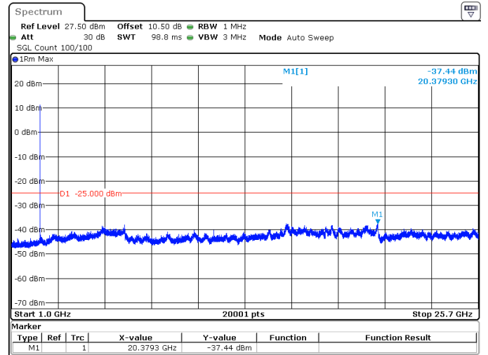
10MHz_15kHz_2505MHz_DFT-s-OFDM QPSK_RB1@0 -37.44 dBm
