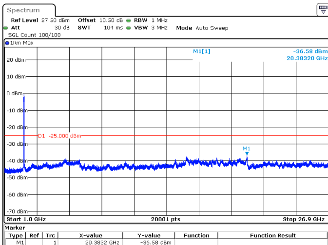
90MHz_30kHz_2541MHz_DFT-s-OFDM QPSK_RB243@0 -36.58 dBm
