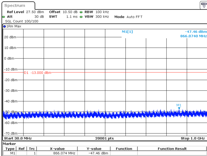
20MHz_15kHz_1770MHz_DFT-s-OFDM QPSK_RB1@105 -47.46 dBm
