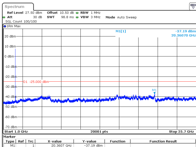
5MHz_15kHz_2535MHz_DFT-s-OFDM QPSK_RB25@0 -37.19 dBm
