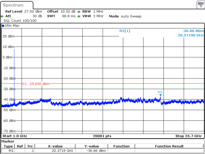
5MHz_15kHz_2567.5MHz_DFT-s-OFDM QPSK_RB25@0 -36.86 dBm
