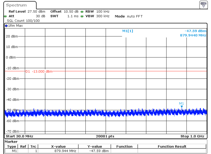
30MHz_15kHz_1765MHz_DFT-s-OFDM QPSK_RB1@0 -47.59 dBm
