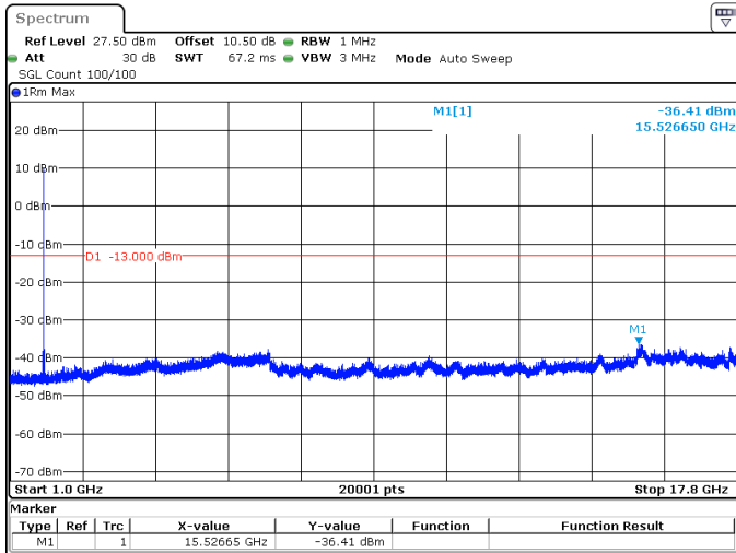
10MHz_15kHz_1775MHz_DFT-s-OFDM QPSK_RB1@0 -36.41 dBm
