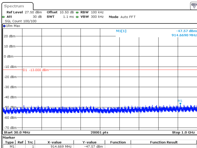
5MHz_15kHz_1745MHz_DFT-s-OFDM QPSK_RB25@0 -47.57 dBm
