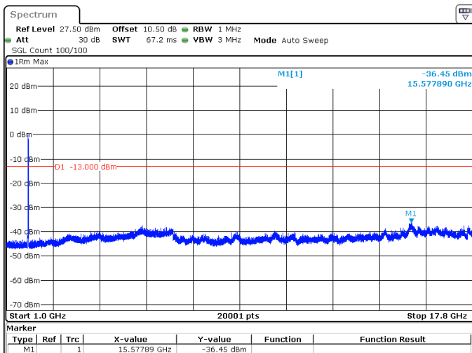
20MHz_15kHz_1770MHz_DFT-s-OFDM QPSK_RB100@0 -36.45 dBm
