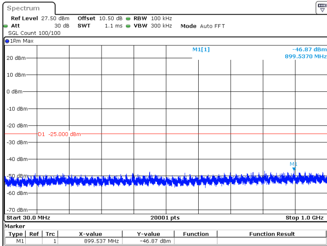
100MHz_30kHz_2640MHz_DFT-s-OFDM QPSK_RB1@0 -46.87 dBm
