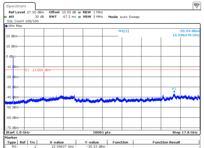
20MHz_15kHz_1720MHz_DFT-s-OFDM QPSK_RB100@0 -35.53 dBm
