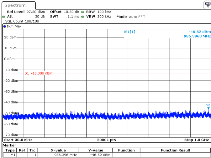
10MHz_15kHz_1745MHz_DFT-s-OFDM QPSK_RB1@0 -46.52 dBm
