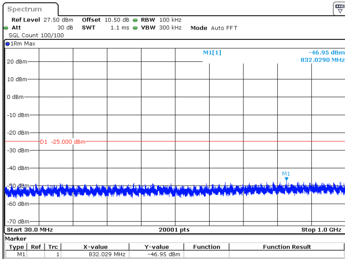
10MHz_15kHz_2505MHz_DFT-s-OFDM QPSK_RB1@51 -46.95 dBm
