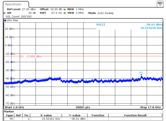
20MHz_15kHz_1770MHz_DFT-s-OFDM QPSK_RB1@105 -36.61 dBm
