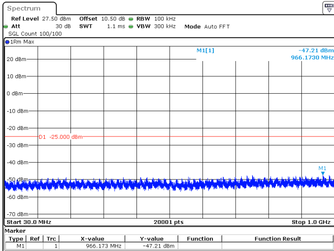
10MHz_15kHz_2505MHz_DFT-s-OFDM QPSK_RB1@0 -47.21 dBm
