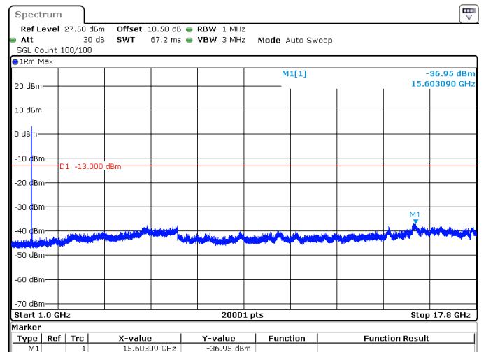
10MHz_15kHz_1715MHz_DFT-s-OFDM QPSK_RB50@0 -36.95 dBm
