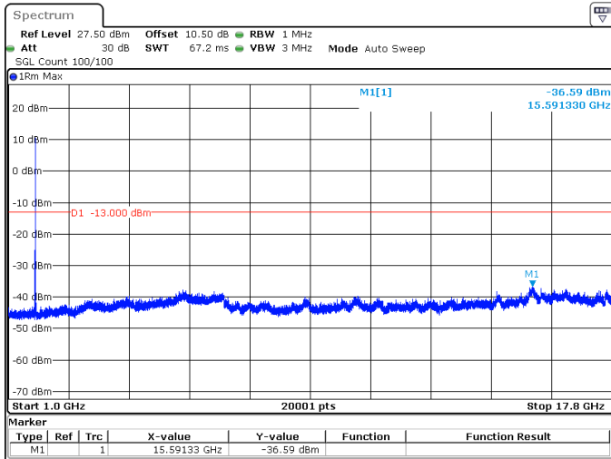
20MHz_15kHz_1745MHz_DFT-s-OFDM QPSK_RB1@0 -36.59 dBm
