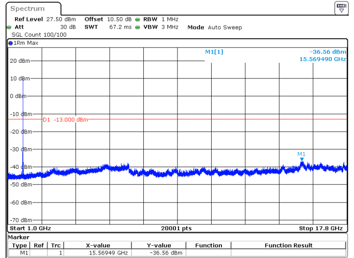
10MHz_15kHz_1745MHz_DFT-s-OFDM QPSK_RB1@0 -36.56 dBm
