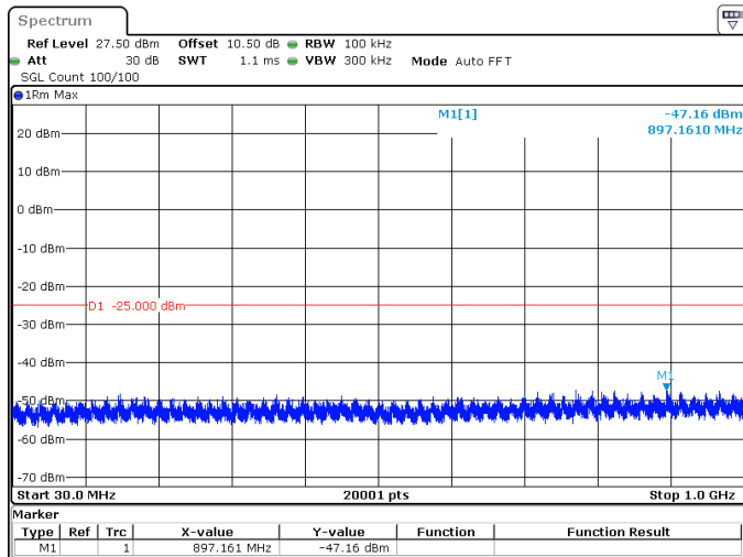
5MHz_15kHz_2535MHz_DFT-s-OFDM QPSK_RB1@0 -47.16 dBm
