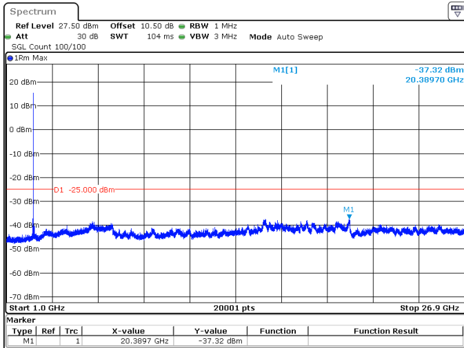
90MHz_30kHz_2541MHz_DFT-s-OFDM QPSK_RB1@0 -37.32 dBm
