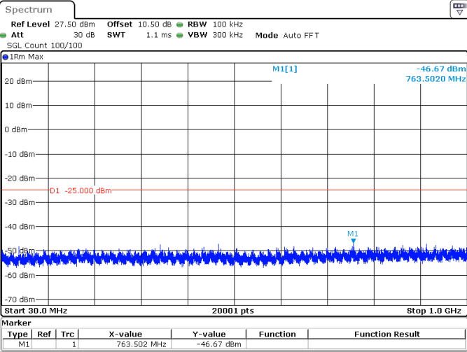
100MHz_30kHz_2592.99MHz_DFT-s-OFDM QPSK_RB270@0 -46.67 dBm
