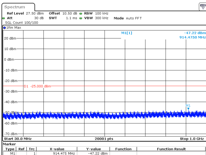
80MHz_30kHz_2649.99MHz_DFT-s-OFDM QPSK_RB216@0 -47.22 dBm
