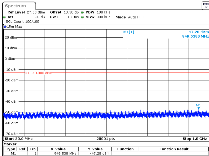
40MHz_15kHz_1760MHz_DFT-s-OFDM QPSK_RB1@0 -47.28 dBm
