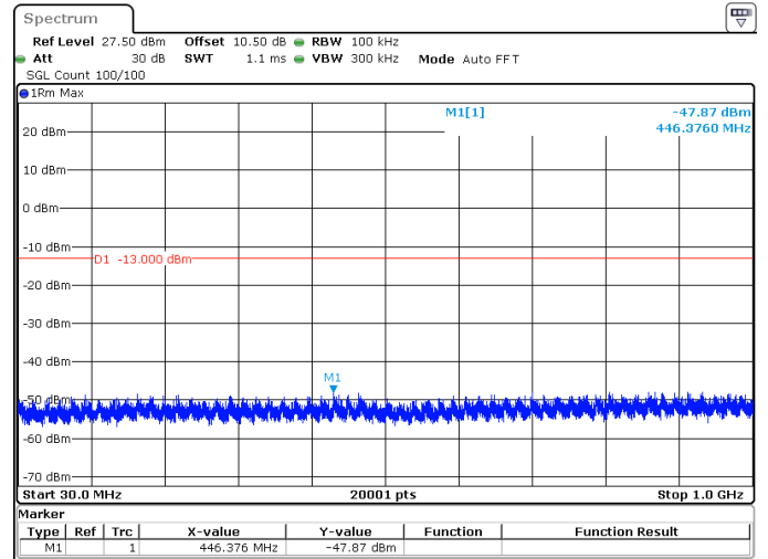
10MHz_15kHz_1775MHz_DFT-s-OFDM QPSK_RB1@0 -47.87 dBm
