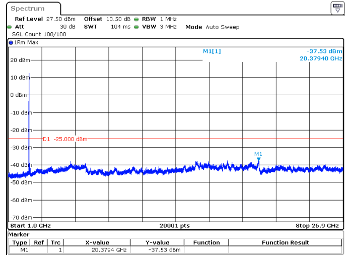
100MHz_30kHz_2640MHz_DFT-s-OFDM QPSK_RB1@0 -37.53 dBm
