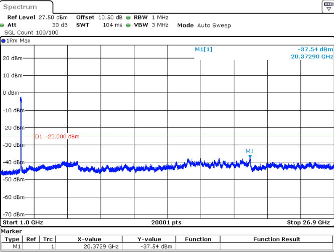
100MHz_30kHz_2546.01MHz_DFT-s-OFDM QPSK_RB270@0 -37.54 dBm
