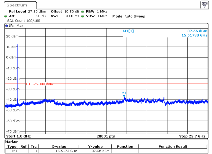
10MHz_15kHz_2535MHz_DFT-s-OFDM QPSK_RB1@0 -37.56 dBm
