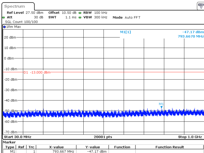
10MHz_15kHz_1715MHz_DFT-s-OFDM QPSK_RB50@0 -47.17 dBm
