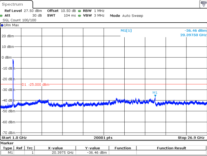
100MHz_30kHz_2592.99MHz_DFT-s-OFDM QPSK_RB270@0 -36.46 dBm
