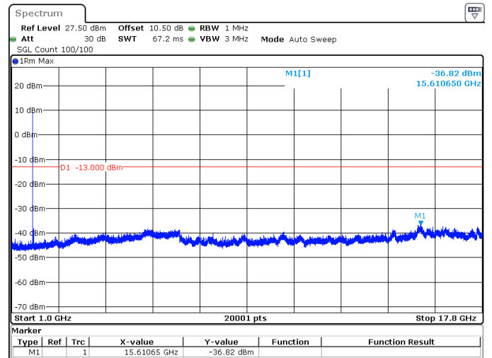
40MHz_15kHz_1760MHz_DFT-s-OFDM QPSK_RB1@0 -36.82 dBm
