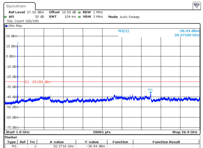
80MHz_30kHz_2649.99MHz_DFT-s-OFDM QPSK_RB1@216 -36.94 dBm
