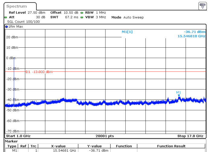
20MHz_15kHz_1745MHz_DFT-s-OFDM QPSK_RB100@0 -36.71 dBm
