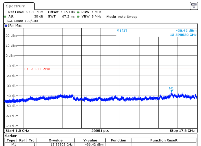
10MHz_15kHz_1745MHz_DFT-s-OFDM QPSK_RB50@0 -36.42 dBm
