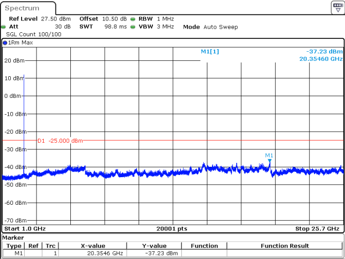
5MHz_15kHz_2567.5MHz_DFT-s-OFDM QPSK_RB1@24 -37.23 dBm
