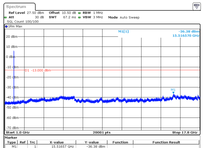
5MHz_15kHz_1777.5MHz_DFT-s-OFDM QPSK_RB25@0 -36.38 dBm
