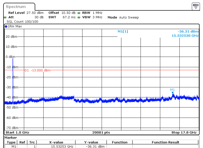
25MHz_15kHz_1722.5MHz_DFT-s-OFDM QPSK_RB128@0 -36.31 dBm
