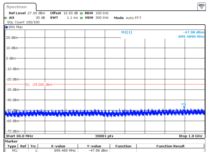
5MHz_15kHz_2535MHz_DFT-s-OFDM QPSK_RB25@0 -47.98 dBm
