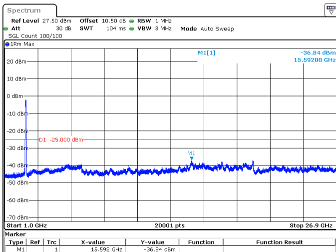
100MHz_30kHz_2640MHz_DFT-s-OFDM QPSK_RB270@0 -36.84 dBm
