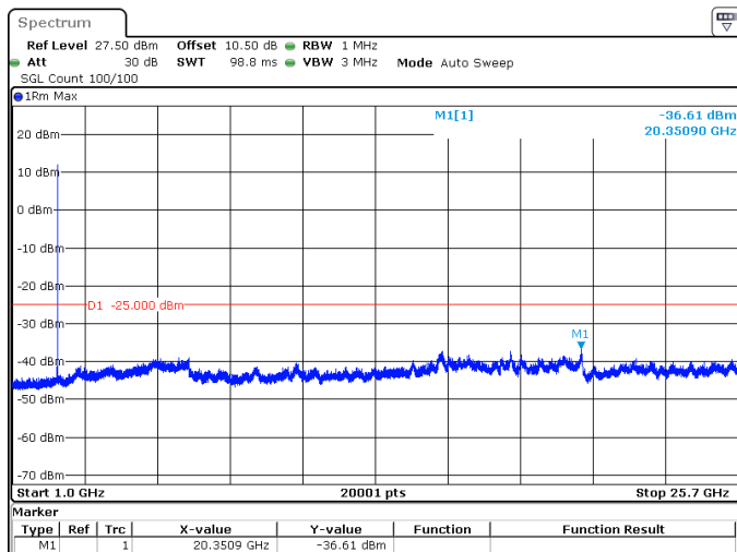
5MHz_15kHz_2535MHz_DFT-s-OFDM QPSK_RB1@24 -36.61 dBm
