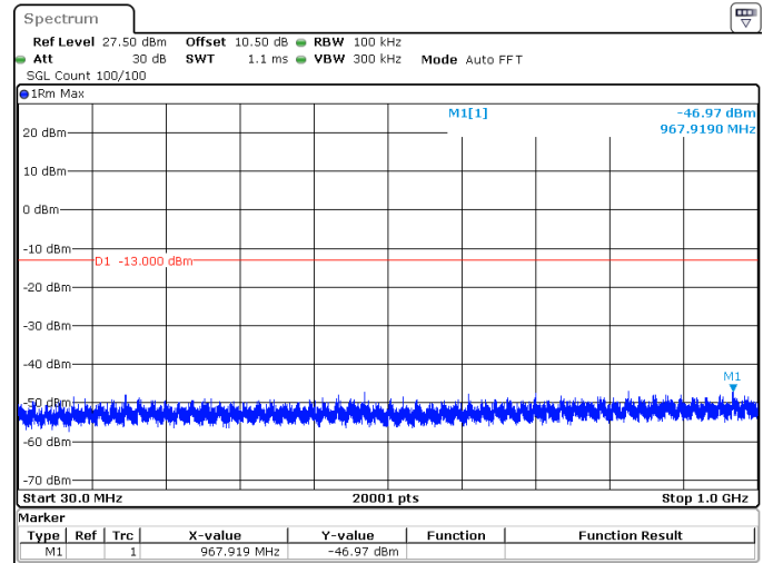
20MHz_15kHz_1745MHz_DFT-s-OFDM QPSK_RB1@0 -46.97 dBm
