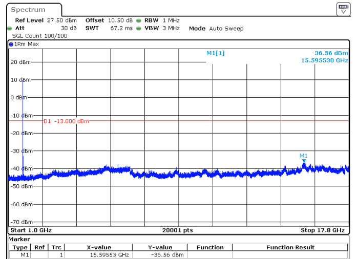
20MHz_15kHz_1720MHz_DFT-s-OFDM QPSK_RB1@0 -36.56 dBm
