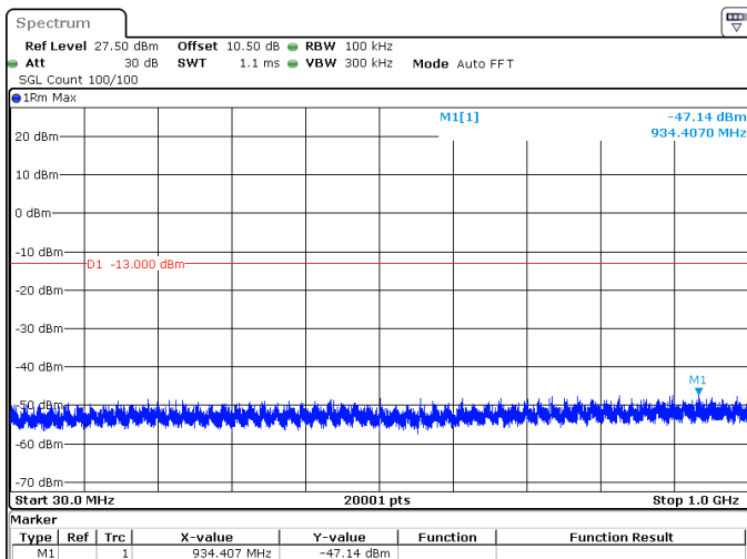
10MHz_15kHz_1775MHz_DFT-s-OFDM QPSK_RB50@0 -47.14 dBm
