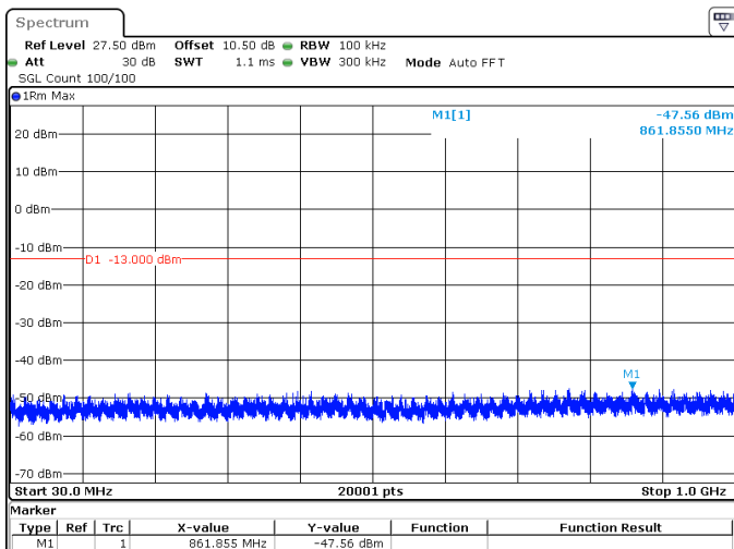
20MHz_15kHz_1745MHz_DFT-s-OFDM QPSK_RB100@0 -47.56 dBm
