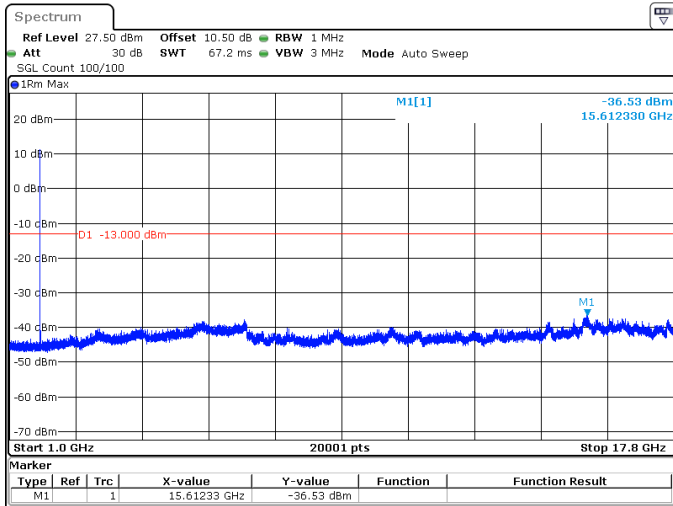
20MHz_15kHz_1770MHz_DFT-s-OFDM QPSK_RB1@0 -36.53 dBm
