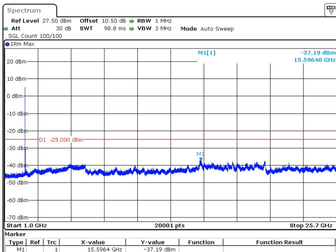
10MHz_15kHz_2505MHz_DFT-s-OFDM QPSK_RB50@0 -37.19 dBm
