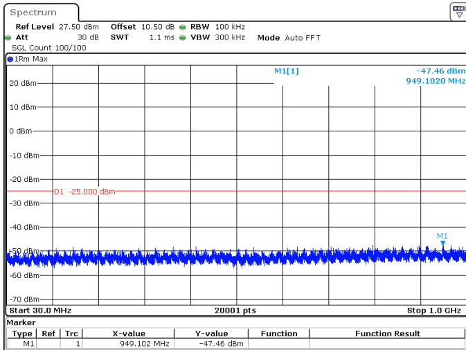
100MHz_30kHz_2640MHz_DFT-s-OFDM QPSK_RB1@272 -47.46 dBm
