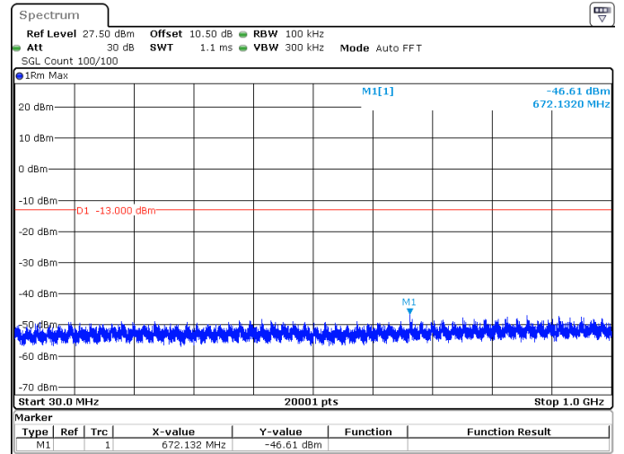
20MHz_15kHz_1770MHz_DFT-s-OFDM QPSK_RB1@0 -46.61 dBm
