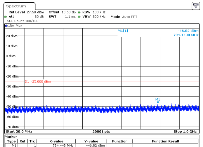
10MHz_15kHz_2505MHz_DFT-s-OFDM QPSK_RB50@0 -46.82 dBm
