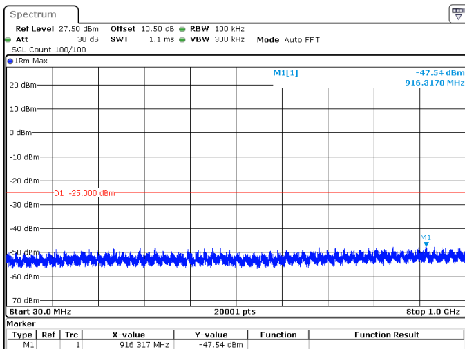
80MHz_30kHz_2649.99MHz_DFT-s-OFDM QPSK_RB1@216 -47.54 dBm
