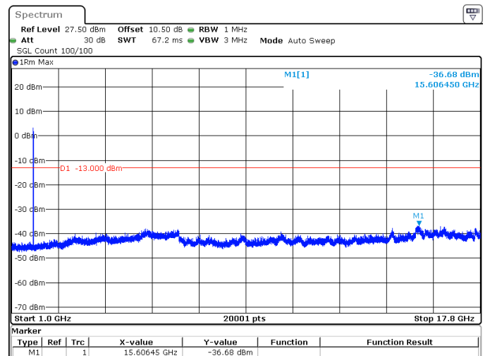
10MHz_15kHz_1775MHz_DFT-s-OFDM QPSK_RB50@0 -36.68 dBm
