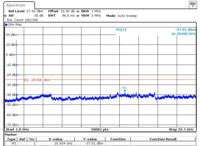
10MHz_15kHz_2505MHz_DFT-s-OFDM QPSK_RB1@51 -37.01 dBm
