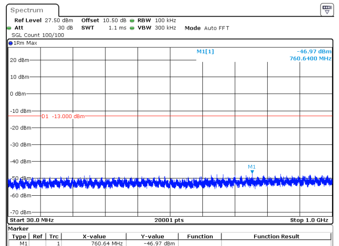
20MHz_15kHz_1770MHz_DFT-s-OFDM QPSK_RB100@0 -46.97 dBm
