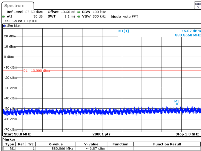
20MHz_15kHz_1720MHz_DFT-s-OFDM QPSK_RB1@0 -46.87 dBm
