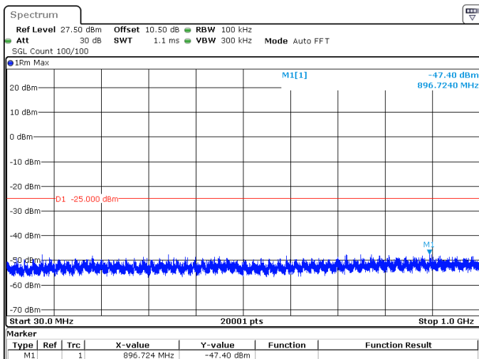
10MHz_15kHz_2535MHz_DFT-s-OFDM QPSK_RB50@0 -47.40 dBm
