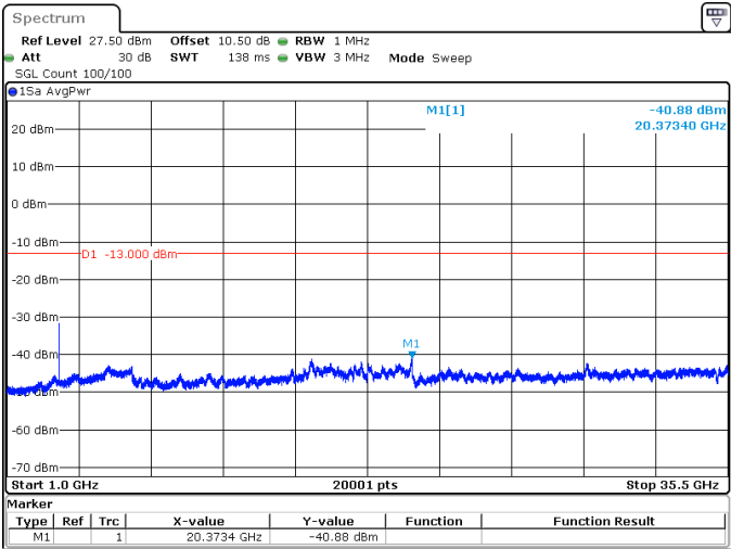
20MHz_15kHz_3500MHz_DFT-s-OFDM QPSK_RB100@0 -40.88 dBm
