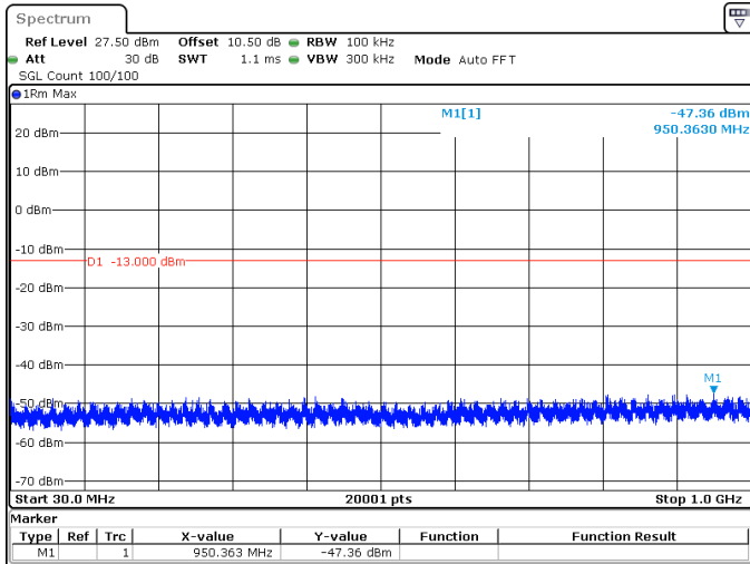
10MHz_30kHz_3455MHz_DFT-s-OFDM QPSK_RB1@0 -47.36 dBm
