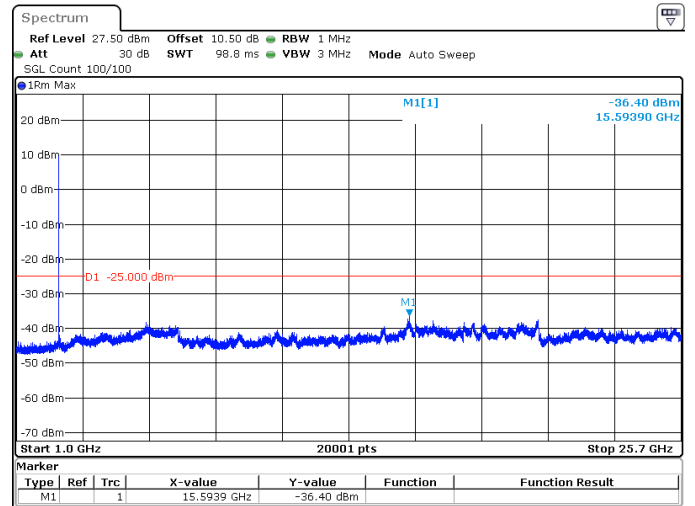
10MHz_15kHz_2565MHz_DFT-s-OFDM QPSK_RB1@51 -36.40 dBm
