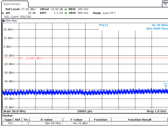
40MHz_15kHz_3470MHz_DFT-s-OFDM QPSK_RB1@215 -46.78 dBm
