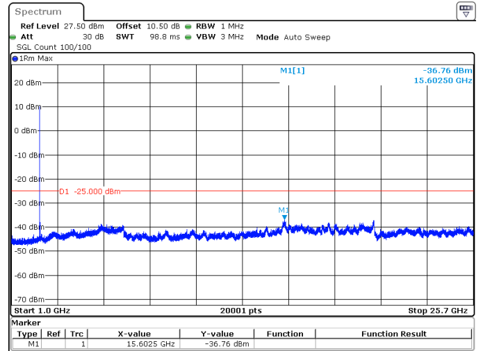
20MHz_15kHz_2510MHz_DFT-s-OFDM QPSK_RB1@0 -36.76 dBm
