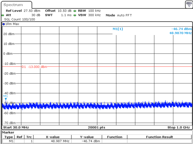
20MHz_30kHz_3460MHz_DFT-s-OFDM QPSK_RB1@0 -46.74 dBm
