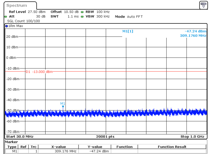
40MHz_15kHz_3500MHz_DFT-s-OFDM QPSK_RB1@215 -47.24 dBm
