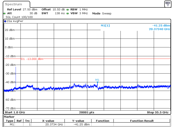
20MHz_15kHz_3460MHz_DFT-s-OFDM QPSK_RB1@0 -41.25 dBm
