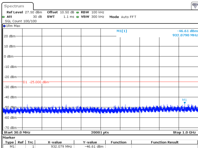
20MHz_15kHz_2510MHz_DFT-s-OFDM QPSK_RB100@0 -46.61 dBm
