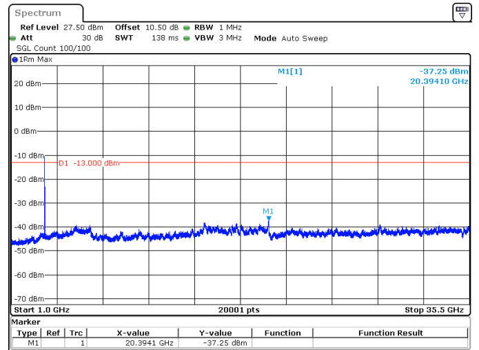
40MHz_15kHz_3530MHz_DFT-s-OFDM QPSK_RB1@0 -37.25 dBm
