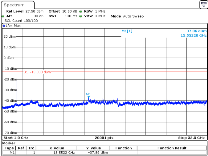
20MHz_30kHz_3460MHz_DFT-s-OFDM QPSK_RB1@50 -37.86 dBm
