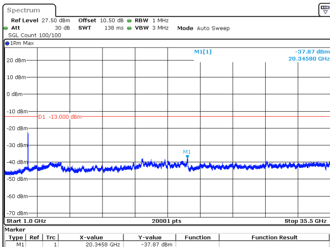
40MHz_30kHz_3470MHz_DFT-s-OFDM QPSK_RB100@0 -37.87 dBm
