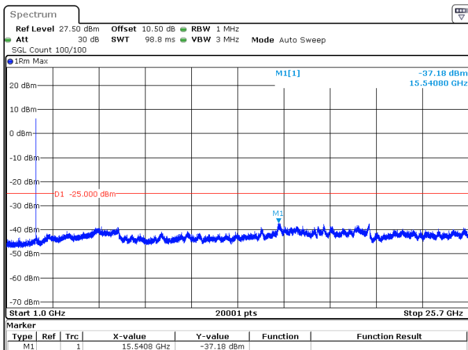
10MHz_15kHz_2565MHz_DFT-s-OFDM QPSK_RB50@0 -37.18 dBm
