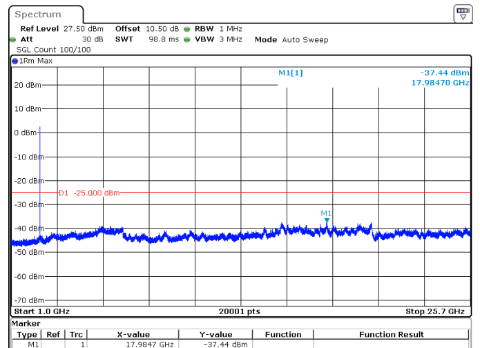
20MHz_15kHz_2535MHz_DFT-s-OFDM QPSK_RB100@0 -37.44 dBm
