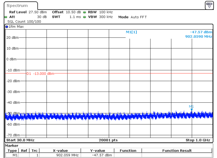
20MHz_30kHz_3540MHz_DFT-s-OFDM QPSK_RB1@50 -47.57 dBm
