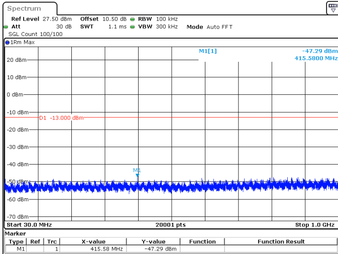
40MHz_15kHz_3470MHz_DFT-s-OFDM QPSK_RB1@0 -47.29 dBm
