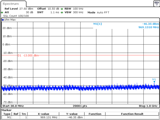
20MHz_30kHz_3460MHz_DFT-s-OFDM QPSK_RB1@50 -46.35 dBm
