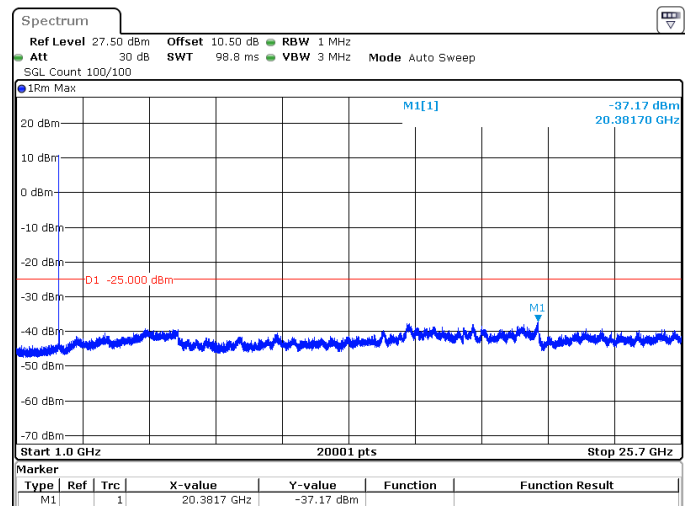
20MHz_15kHz_2560MHz_DFT-s-OFDM QPSK_RB1@105 -37.17 dBm
