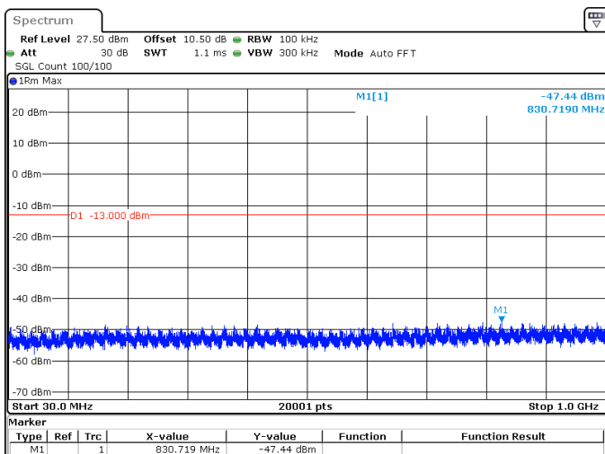
10MHz_30kHz_3500MHz_DFT-s-OFDM QPSK_RB24@0 -47.44 dBm
