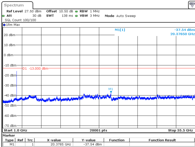
40MHz_30kHz_3470MHz_DFT-s-OFDM QPSK_RB1@105 -37.54 dBm
