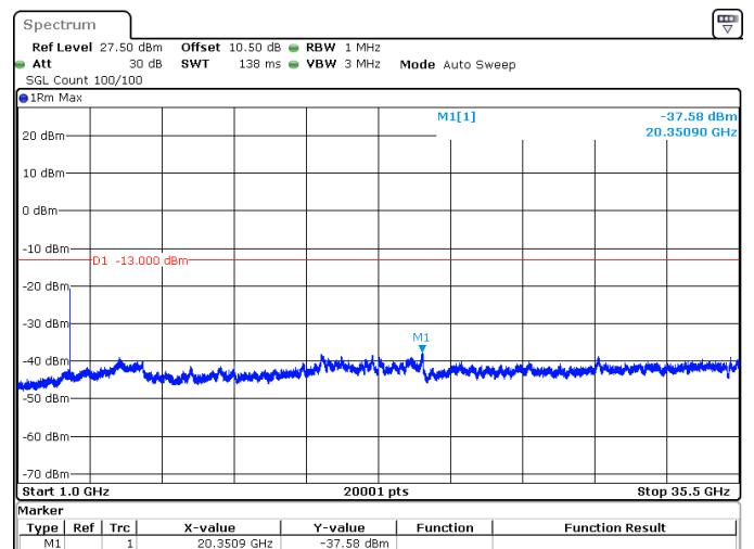
20MHz_30kHz_3500MHz_DFT-s-OFDM QPSK_RB50@0 -37.58 dBm
