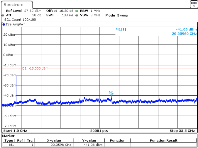
20MHz_15kHz_3500MHz_DFT-s-OFDM QPSK_RB1@105 -41.06 dBm
