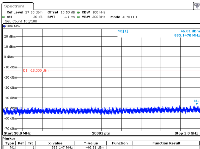
20MHz_30kHz_3540MHz_DFT-s-OFDM QPSK_RB50@0 -46.81 dBm
