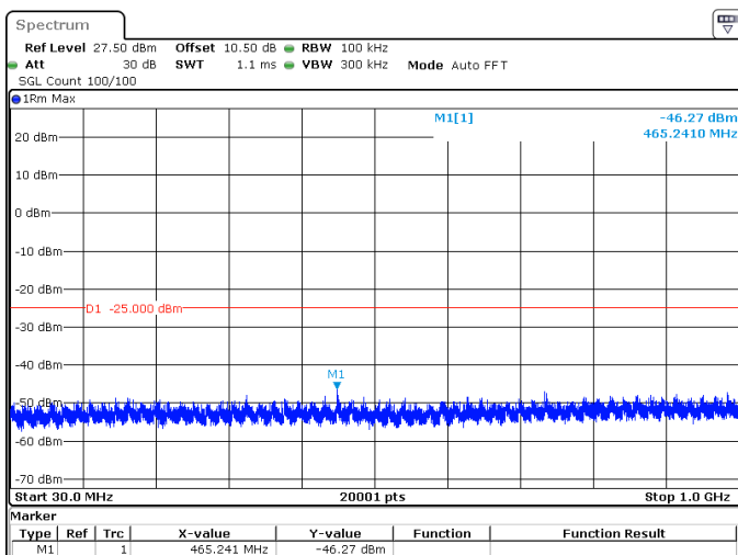
20MHz_15kHz_2560MHz_DFT-s-OFDM QPSK_RB100@0 -46.27 dBm
