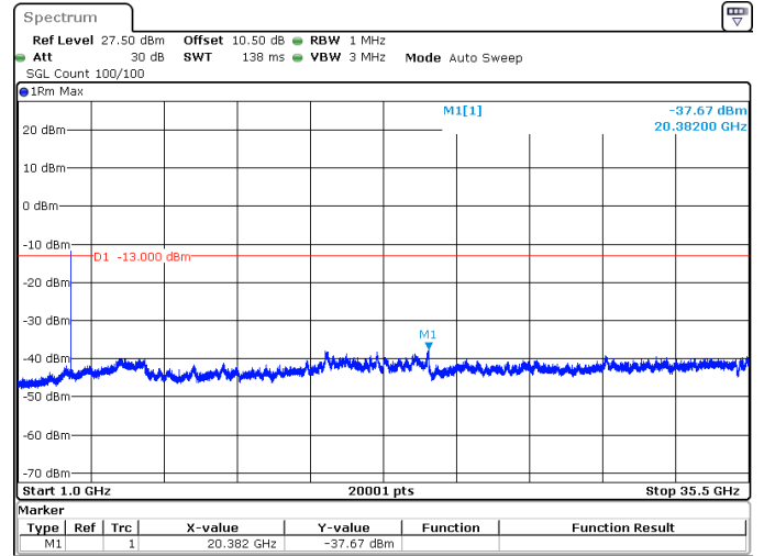
40MHz_15kHz_3470MHz_DFT-s-OFDM QPSK_RB1@215 -37.67 dBm
