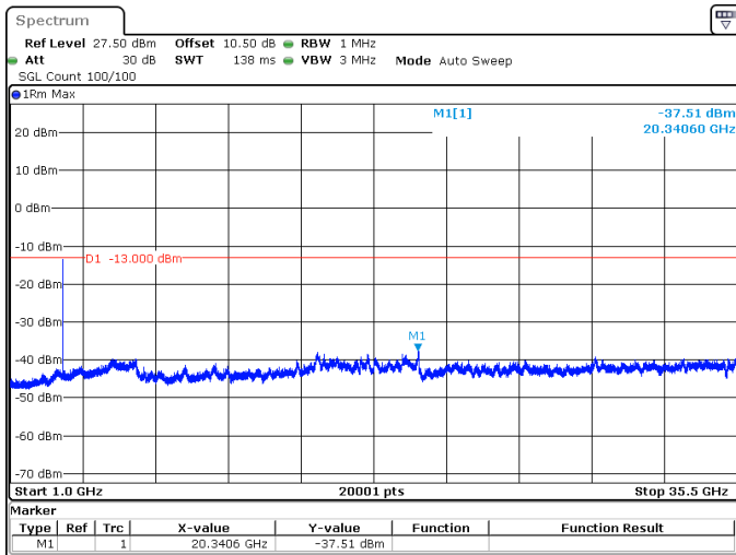
10MHz_30kHz_3500MHz_DFT-s-OFDM QPSK_RB1@0 -37.51 dBm
