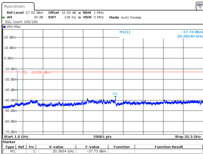
20MHz_30kHz_3500MHz_DFT-s-OFDM QPSK_RB1@50 -37.73 dBm
