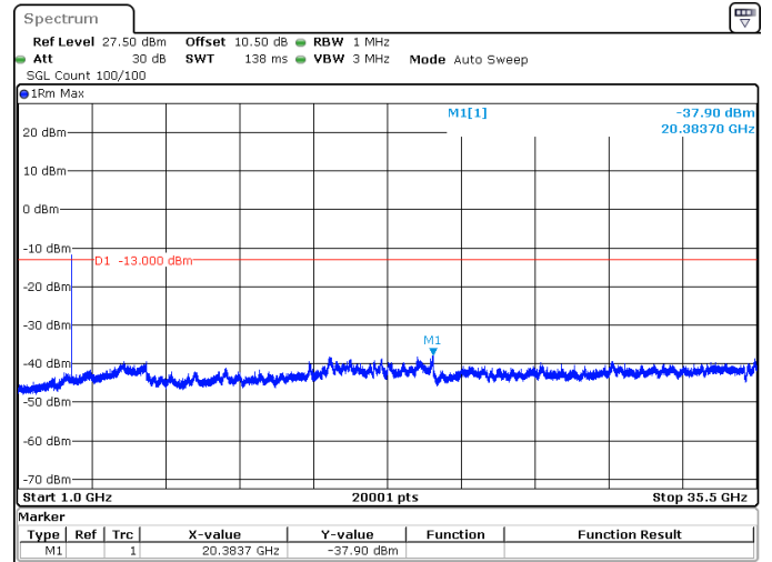
10MHz_15kHz_3500MHz_DFT-s-OFDM QPSK_RB1@0 -37.90 dBm
