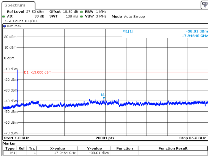
30MHz_15kHz_3465MHz_DFT-s-OFDM QPSK_RB1@0 -38.01 dBm
