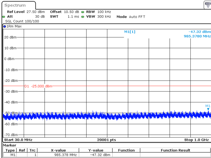
20MHz_15kHz_2510MHz_DFT-s-OFDM QPSK_RB1@0 -47.32 dBm
