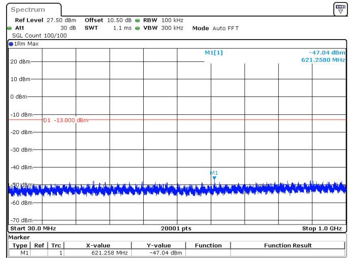
10MHz_30kHz_3500MHz_DFT-s-OFDM QPSK_RB1@0 -47.04 dBm
