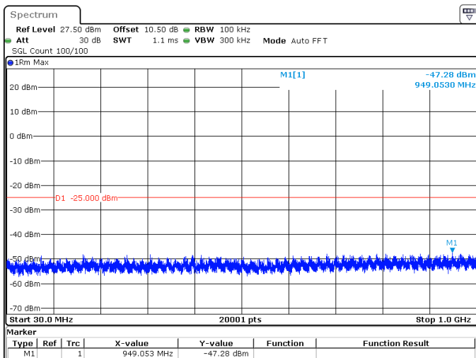
20MHz_15kHz_2560MHz_DFT-s-OFDM QPSK_RB1@105 -47.28 dBm
