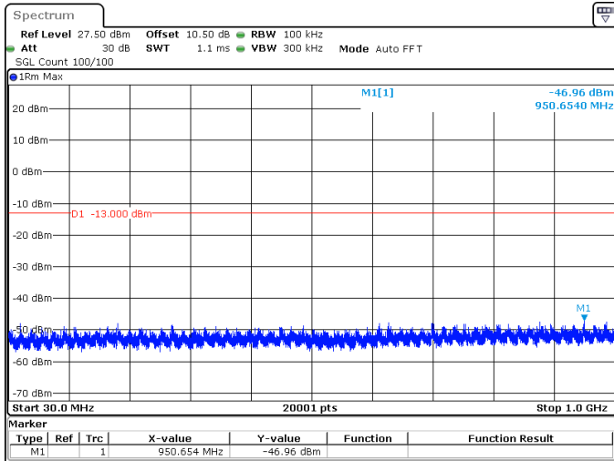
10MHz_15kHz_3500MHz_DFT-s-OFDM QPSK_RB1@0 -46.96 dBm
