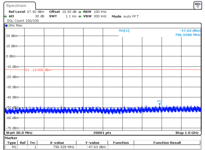
30MHz_15kHz_3535MHz_DFT-s-OFDM QPSK_RB1@0 -47.63 dBm
