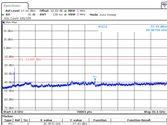
40MHz_15kHz_3530MHz_DFT-s-OFDM QPSK_RB216@0 -37.43 dBm
