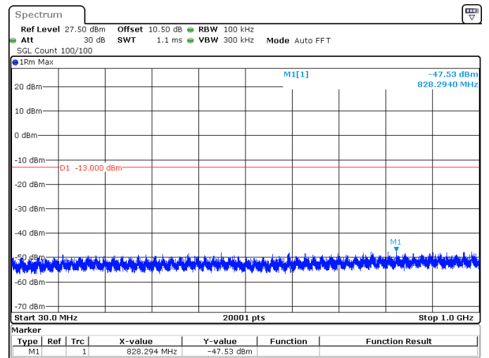
40MHz_15kHz_3530MHz_DFT-s-OFDM QPSK_RB1@215 -47.53 dBm
