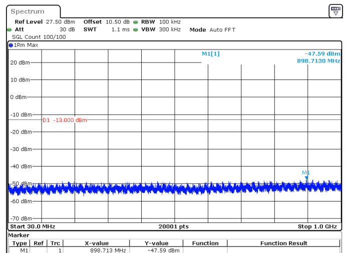
40MHz_15kHz_3530MHz_DFT-s-OFDM QPSK_RB216@0 -47.59 dBm
