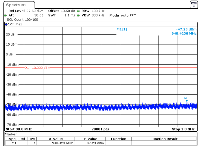
40MHz_30kHz_3470MHz_DFT-s-OFDM QPSK_RB1@0 -47.23 dBm
