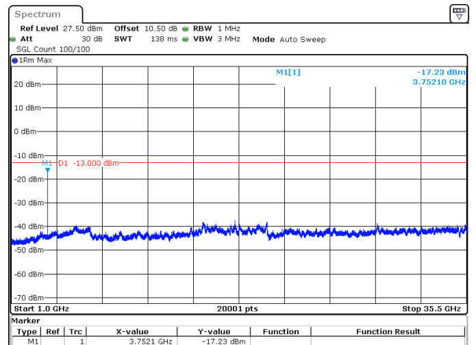
10MHz_15kHz_3500MHz_DFT-s-OFDM QPSK_RB50@0 -17.23 dBm
