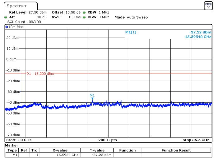
20MHz_30kHz_3500MHz_DFT-s-OFDM QPSK_RB1@0 -37.22 dBm
