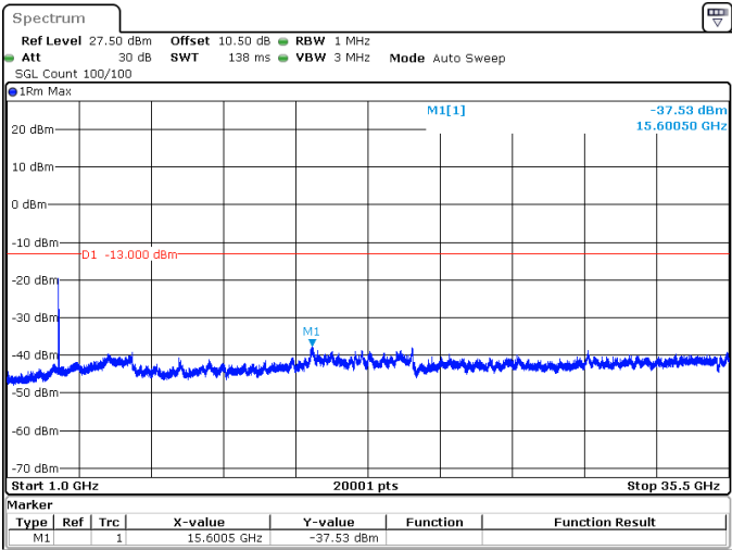
20MHz_30kHz_3460MHz_DFT-s-OFDM QPSK_RB50@0 -37.53 dBm
