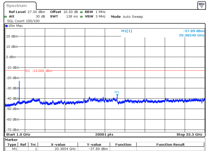
40MHz_15kHz_3470MHz_DFT-s-OFDM QPSK_RB216@0 -37.89 dBm
