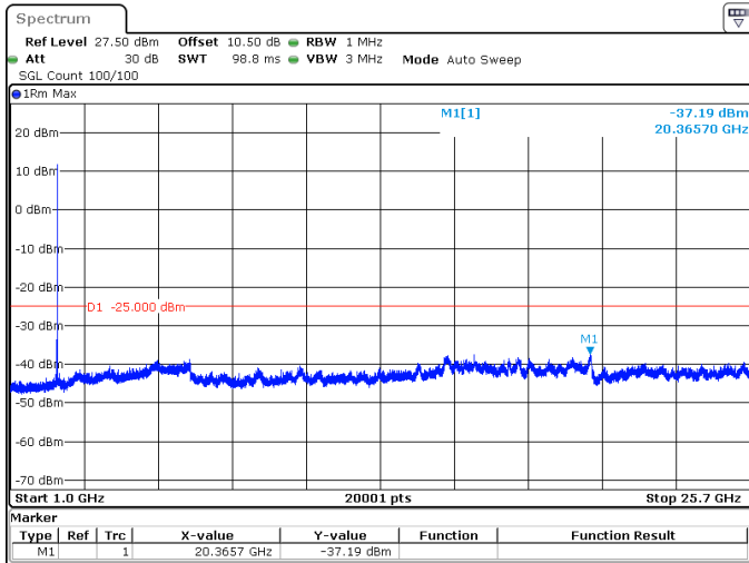
10MHz_15kHz_2565MHz_DFT-s-OFDM QPSK_RB1@0 -37.19 dBm
