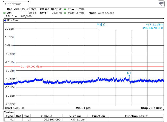
20MHz_15kHz_2535MHz_DFT-s-OFDM QPSK_RB1@0 -37.11 dBm
