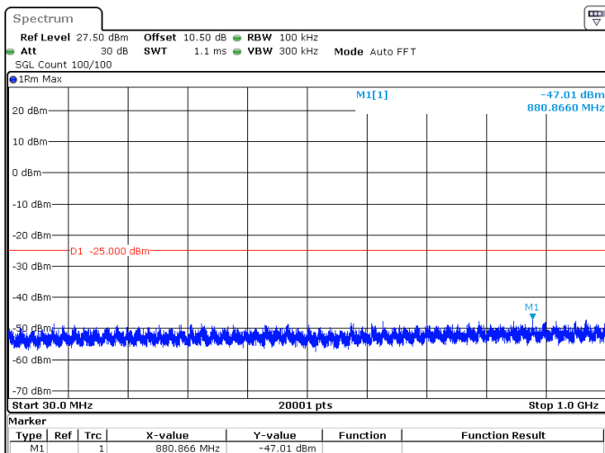
20MHz_15kHz_2535MHz_DFT-s-OFDM QPSK_RB100@0 -47.01 dBm
