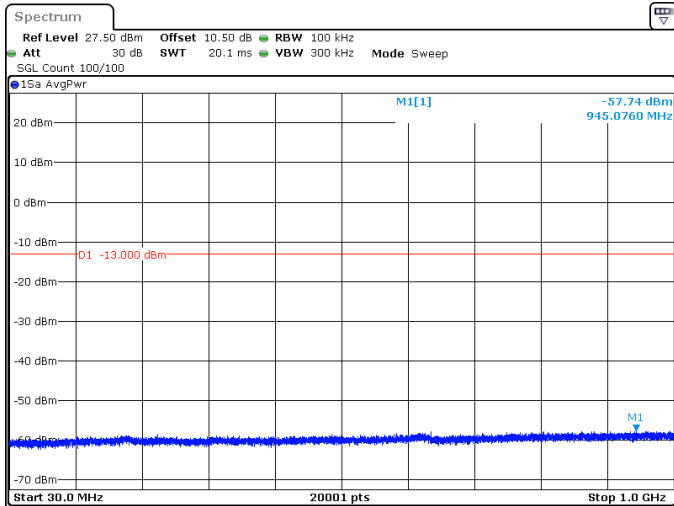
20MHz_15kHz_3460MHz_DFT-s-OFDM QPSK_RB1@0 -57.74 dBm
