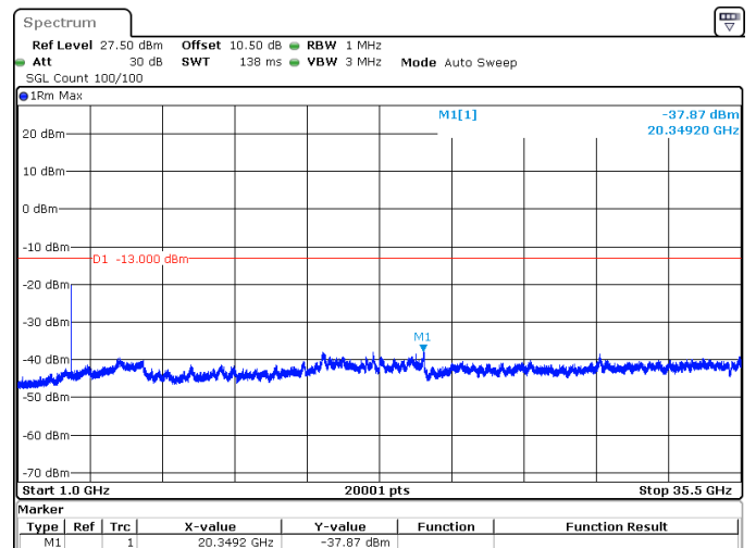
20MHz_30kHz_3540MHz_DFT-s-OFDM QPSK_RB50@0 -37.87 dBm
