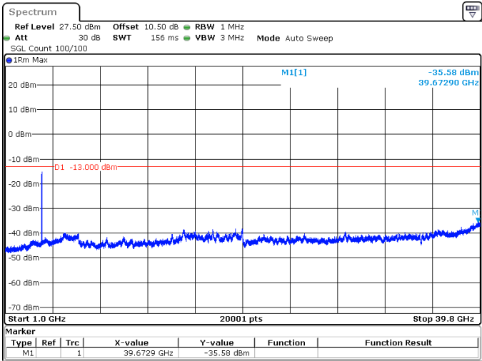
20MHz_15kHz_3970MHz_DFT-s-OFDM QPSK_RB100@0 -35.58 dBm
