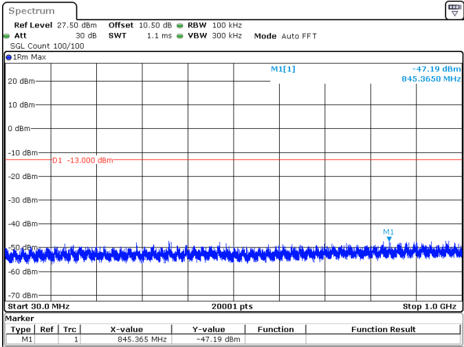
20MHz_15kHz_3970MHz_DFT-s-OFDM QPSK_RB1@105 -47.19 dBm
