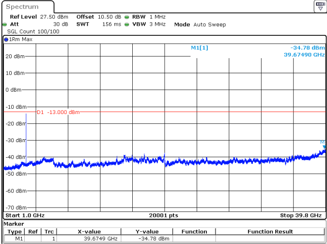
10MHz_30kHz_3705MHz_DFT-s-OFDM QPSK_RB24@0 -34.78 dBm
