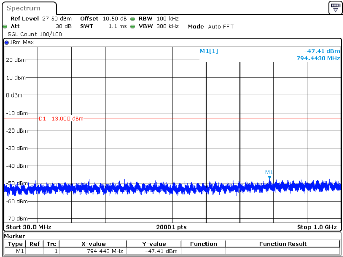
100MHz_30kHz_3500MHz_DFT-s-OFDM QPSK_RB1@272 -47.41 dBm
