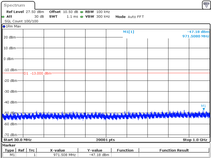
100MHz_30kHz_3500MHz_DFT-s-OFDM QPSK_RB1@0 -47.18 dBm
