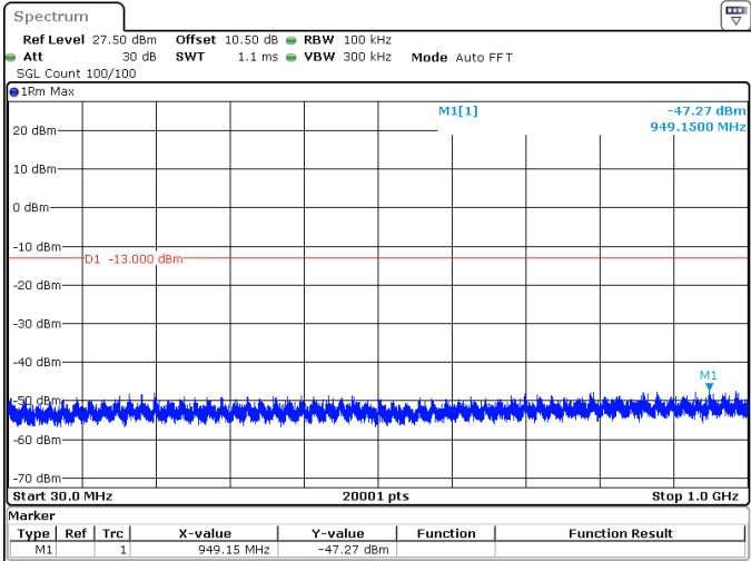
10MHz_30kHz_3705MHz_DFT-s-OFDM QPSK_RB1@0 -47.27 dBm
