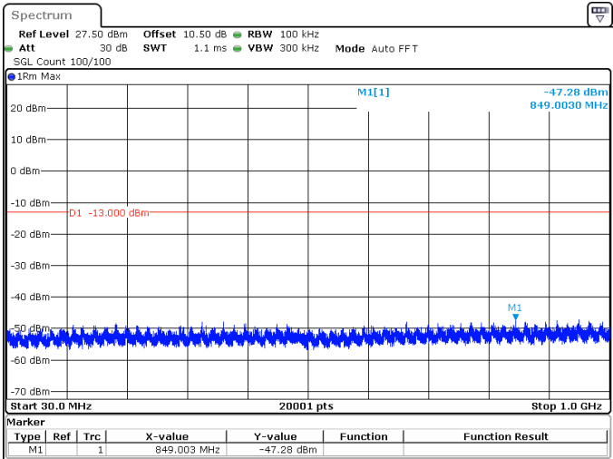
15MHz_15kHz_3707.5MHz_DFT-s-OFDM QPSK_RB1@0 -47.28 dBm
