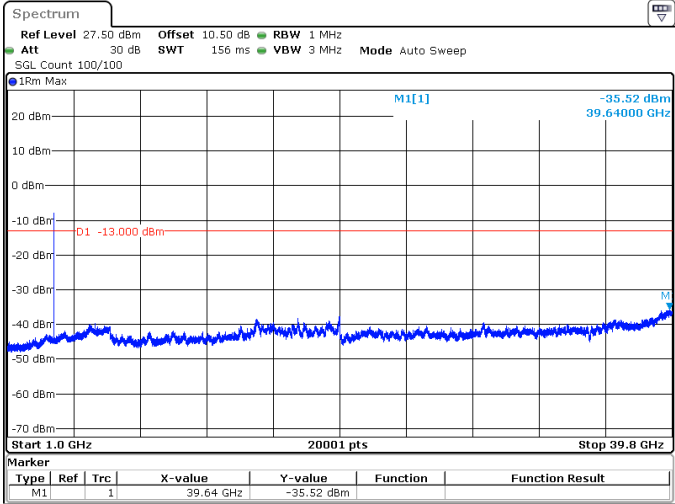
10MHz_30kHz_3705MHz_DFT-s-OFDM QPSK_RB1@23 -35.52 dBm
