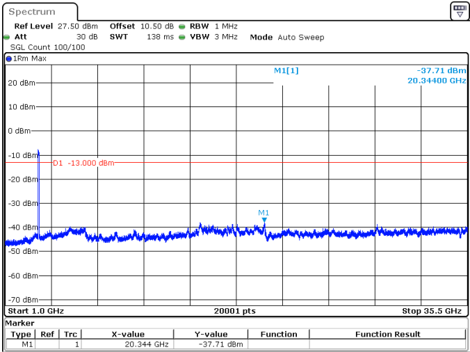
100MHz_30kHz_3500MHz_DFT-s-OFDM QPSK_RB270@0 -37.71 dBm
