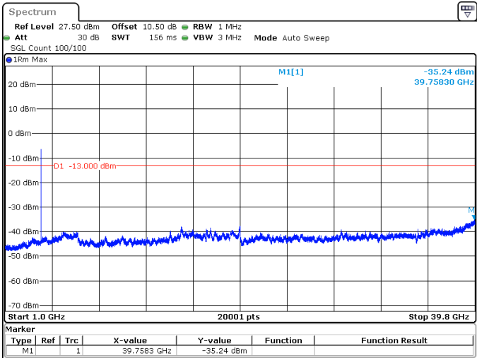
20MHz_15kHz_3970MHz_DFT-s-OFDM QPSK_RB1@0 -35.24 dBm
