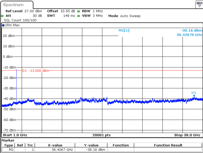
10MHz_15kHz_3705MHz_DFT-s-OFDM QPSK_RB50@0 -38.16 dBm
