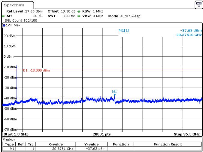
90MHz_30kHz_3495MHz_DFT-s-OFDM QPSK_RB1@0 -37.63 dBm
