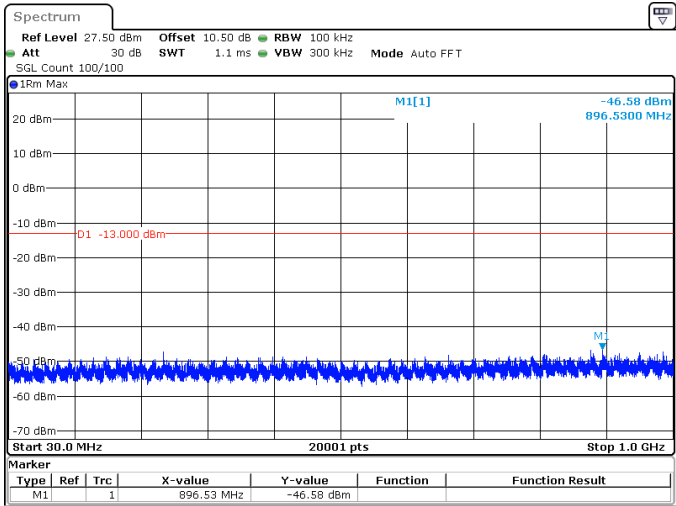
40MHz_30kHz_3500MHz_DFT-s-OFDM QPSK_RB1@0 -46.58 dBm
