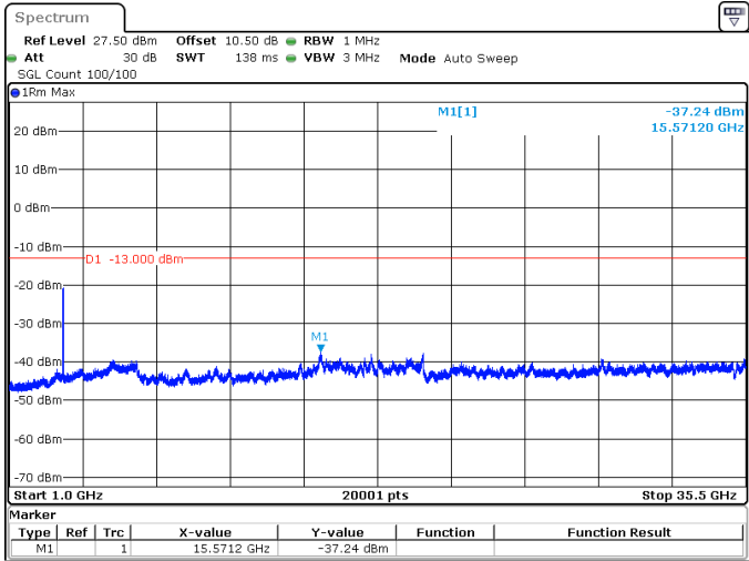
70MHz_30kHz_3515MHz_DFT-s-OFDM QPSK_RB180@0 -37.24 dBm
