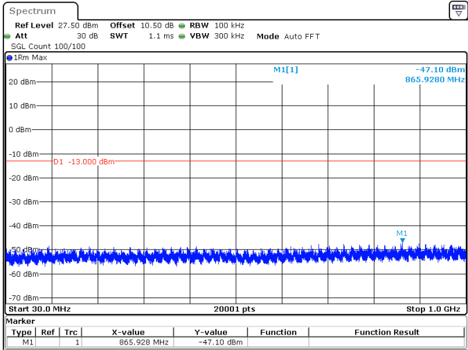
70MHz_30kHz_3485MHz_DFT-s-OFDM QPSK_RB180@0 -47.10 dBm
