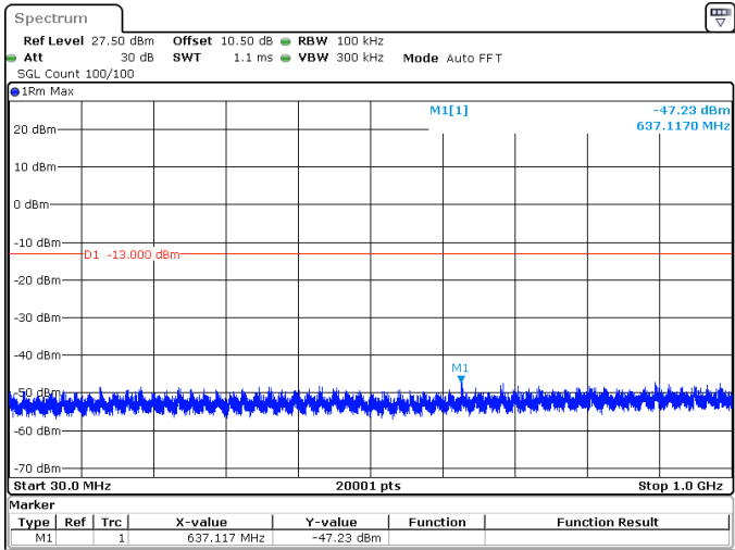
80MHz_30kHz_3510MHz_DFT-s-OFDM QPSK_RB1@0 -47.23 dBm
