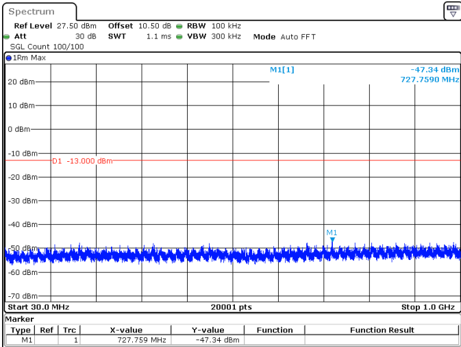
30MHz_30kHz_3465MHz_DFT-s-OFDM QPSK_RB1@77 -47.34 dBm
