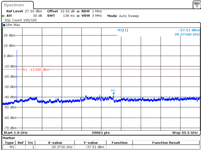
40MHz_30kHz_3470MHz_DFT-s-OFDM QPSK_RB1@105 -37.51 dBm
