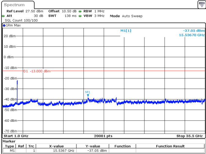
90MHz_30kHz_3495MHz_DFT-s-OFDM QPSK_RB243@0 -37.05 dBm
