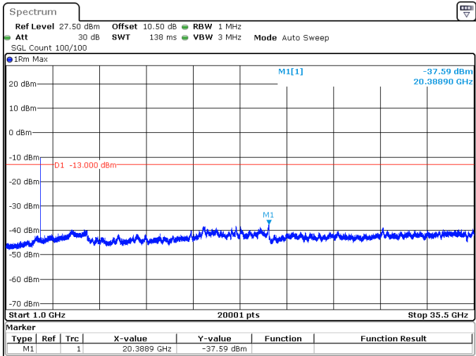
80MHz_30kHz_3510MHz_DFT-s-OFDM QPSK_RB1@216 -37.59 dBm
