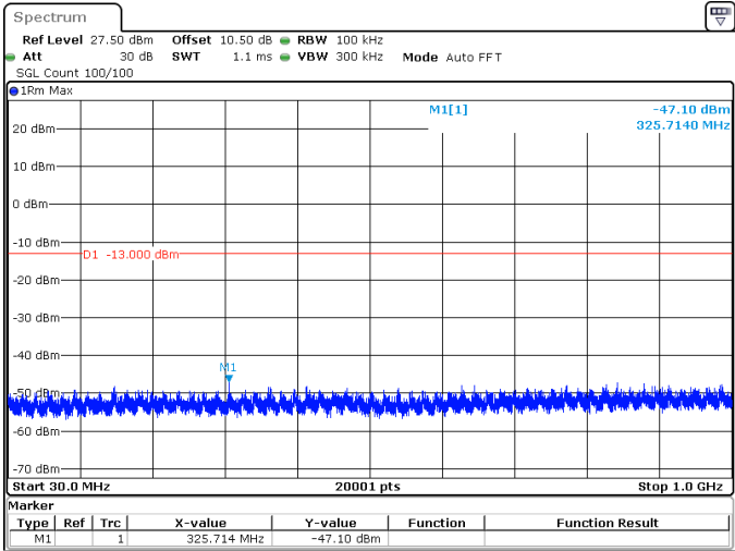
100MHz_30kHz_3500MHz_DFT-s-OFDM QPSK_RB270@0 -47.10 dBm
