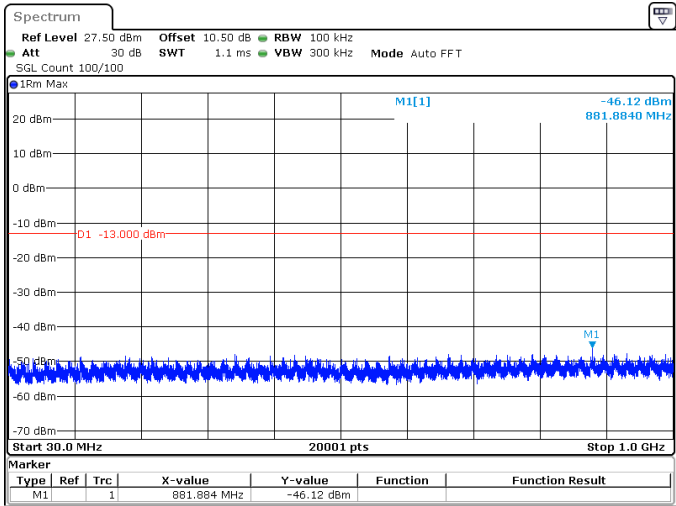
70MHz_30kHz_3500MHz_DFT-s-OFDM QPSK_RB1@0 -46.12 dBm
