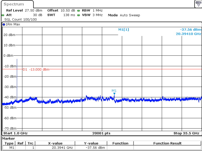
30MHz_30kHz_3535MHz_DFT-s-OFDM QPSK_RB75@0 -37.56 dBm
