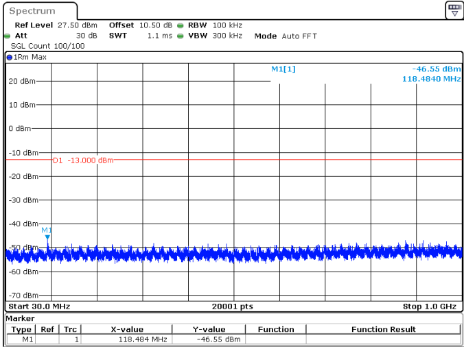
80MHz_30kHz_3510MHz_DFT-s-OFDM QPSK_RB216@0 -46.55 dBm
