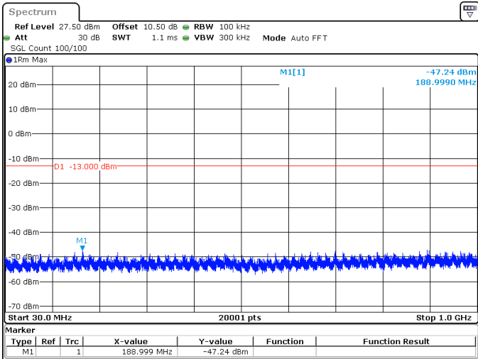
25MHz_30kHz_3500MHz_DFT-s-OFDM QPSK_RB1@64 -47.24 dBm
