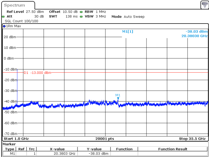
100MHz_30kHz_3500MHz_DFT-s-OFDM QPSK_RB1@0 -38.03 dBm
