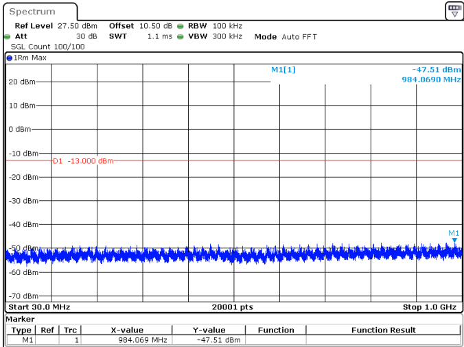
90MHz_30kHz_3505MHz_DFT-s-OFDM QPSK_RB1@244 -47.51 dBm
