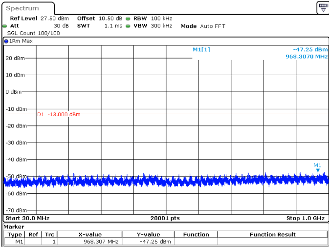
25MHz_30kHz_3537.5MHz_DFT-s-OFDM QPSK_RB1@0 -47.25 dBm
