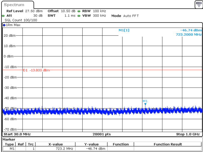
90MHz_30kHz_3505MHz_DFT-s-OFDM QPSK_RB243@0 -46.74 dBm
