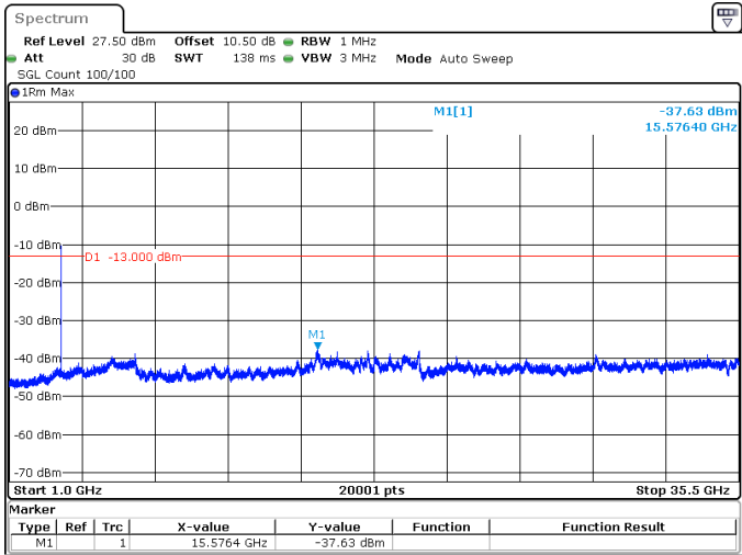
80MHz_30kHz_3490MHz_DFT-s-OFDM QPSK_RB1@0 -37.63 dBm
