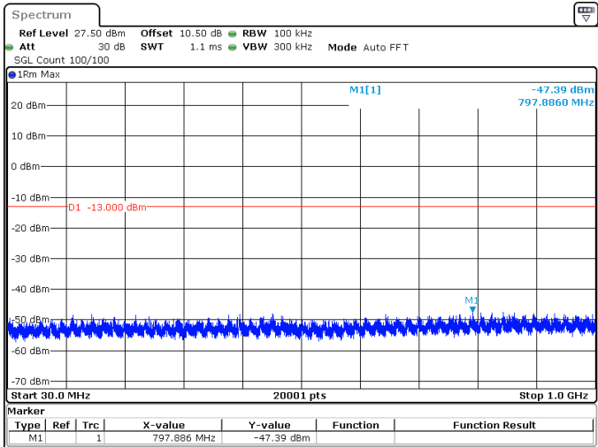
90MHz_30kHz_3495MHz_DFT-s-OFDM QPSK_RB1@244 -47.39 dBm
