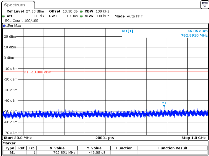
40MHz_30kHz_3470MHz_DFT-s-OFDM QPSK_RB100@0 -46.05 dBm
