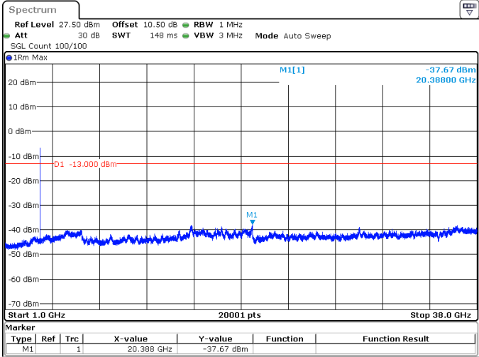
10MHz_15kHz_3705MHz_DFT-s-OFDM QPSK_RB1@0 -37.67 dBm
