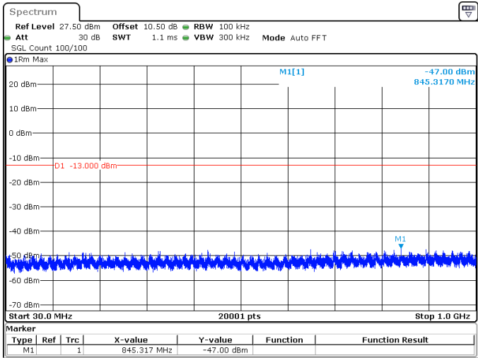
90MHz_30kHz_3500MHz_DFT-s-OFDM QPSK_RB1@0 -47.00 dBm
