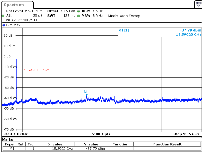
30MHz_30kHz_3465MHz_DFT-s-OFDM QPSK_RB75@0 -37.79 dBm
