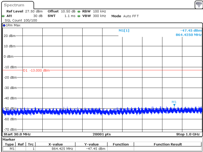
50MHz_30kHz_3525MHz_DFT-s-OFDM QPSK_RB1@0 -47.45 dBm
