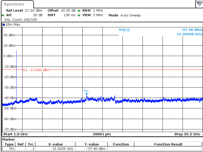
40MHz_30kHz_3470MHz_DFT-s-OFDM QPSK_RB1@0 -37.40 dBm
