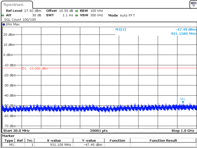
25MHz_30kHz_3500MHz_DFT-s-OFDM QPSK_RB64@0 -47.49 dBm
