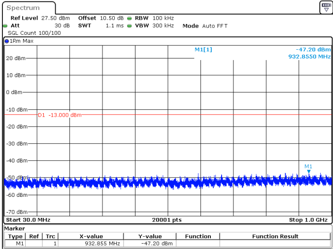
80MHz_30kHz_3500MHz_DFT-s-OFDM QPSK_RB216@0 -47.20 dBm
