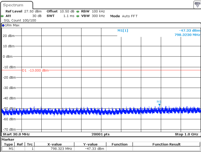
10MHz_15kHz_3750MHz_DFT-s-OFDM QPSK_RB1@0 -47.33 dBm
