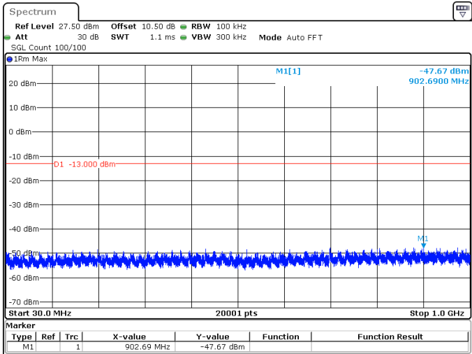
70MHz_30kHz_3485MHz_DFT-s-OFDM QPSK_RB1@188 -47.67 dBm
