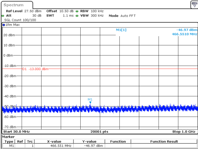
30MHz_30kHz_3500MHz_DFT-s-OFDM QPSK_RB1@0 -46.97 dBm
