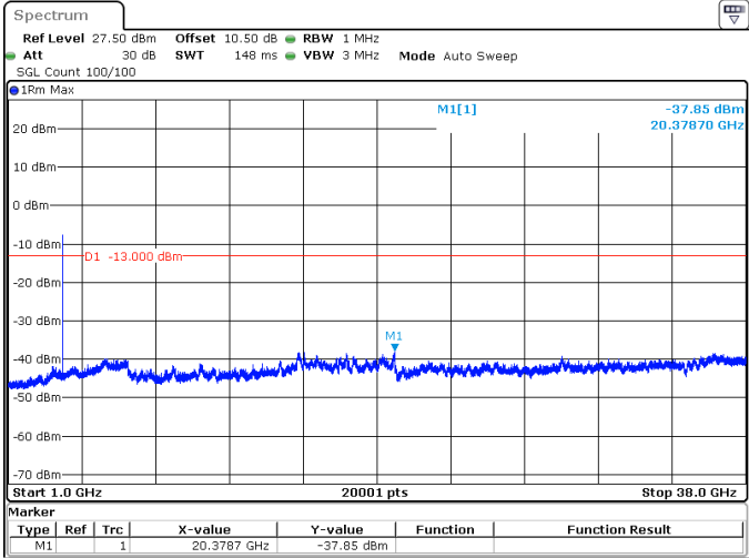
30MHz_15kHz_3750MHz_DFT-s-OFDM QPSK_RB1@0 -37.85 dBm
