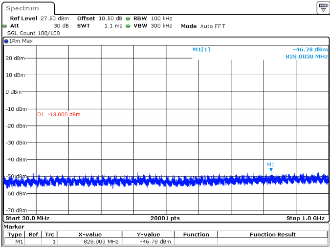
40MHz_30kHz_3750MHz_DFT-s-OFDM QPSK_RB1@0 -46.78 dBm
