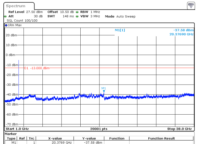
30MHz_15kHz_3785MHz_DFT-s-OFDM QPSK_RB1@0 -37.58 dBm
