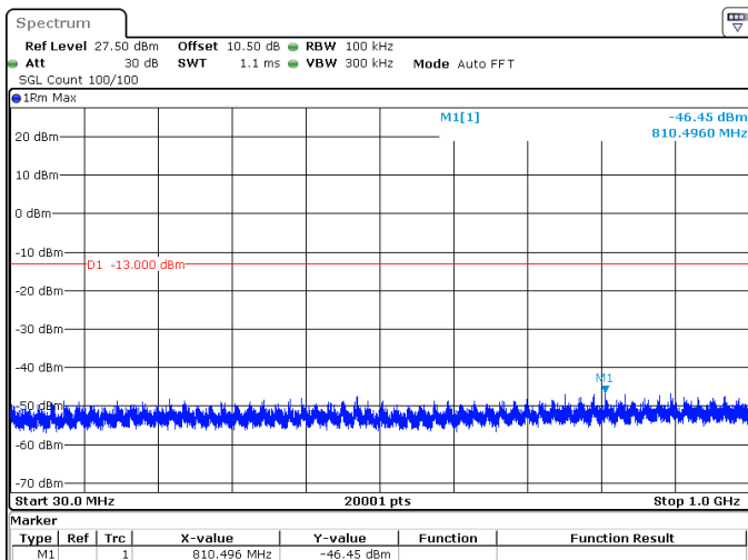
30MHz_15kHz_3785MHz_DFT-s-OFDM QPSK_RB1@0 -46.45 dBm
