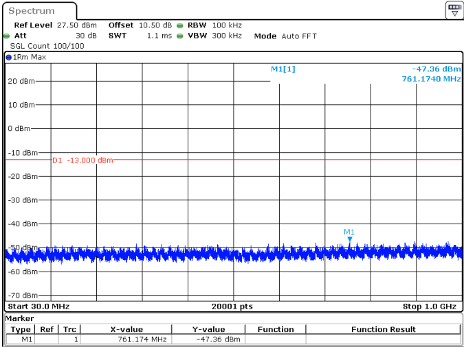
40MHz_30kHz_3720MHz_DFT-s-OFDM QPSK_RB100@0 -47.36 dBm
