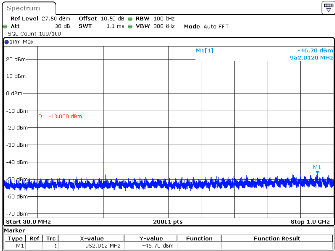
60MHz_30kHz_3750MHz_DFT-s-OFDM QPSK_RB1@0 -46.70 dBm
