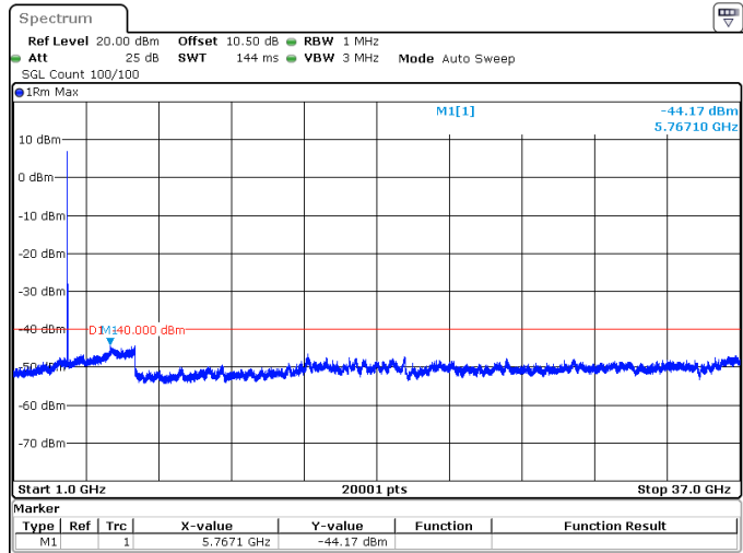
40MHz_30kHz_3680MHz_DFT-s-OFDM QPSK_RB1@0 -44.17 dBm
