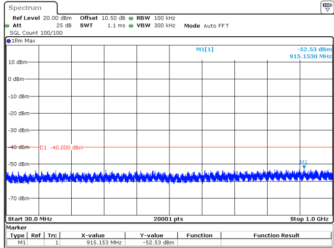
40MHz_30kHz_3680MHz_DFT-s-OFDM QPSK_RB1@105 -52.53 dBm
