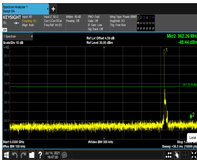
Band5-10MHz-QPSK-20525:30~1000MHz
