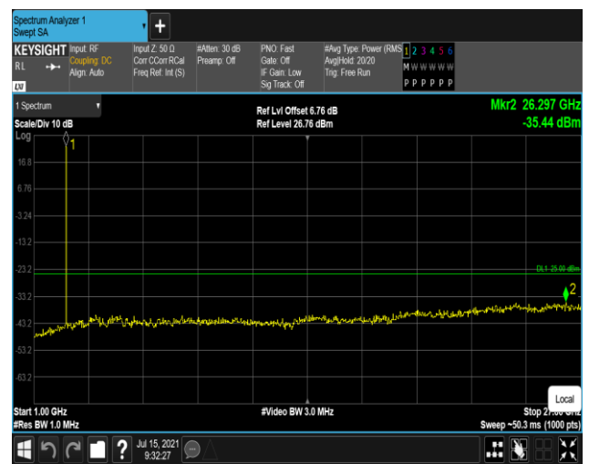
Band41-5MHz-QPSK-40640:1000~27000MHz
