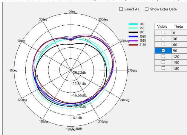
PCS/ WCDMA B1/B2/ LTE B1/B2/B25/B12/B13/B17/B28A/B28B Theta=90deg
