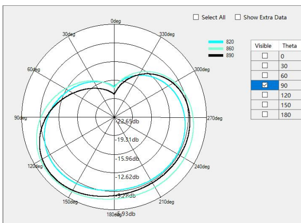
GSM 850/ WCDMA B5/ LTE B5/B26 Theta=90deg
