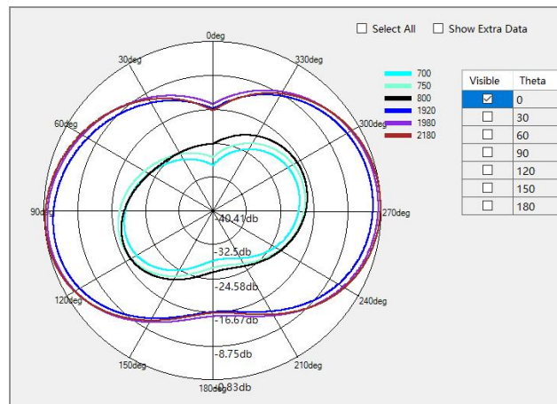
PCS/ WCDMA B1/B2/ LTE B1/B2/B25/B12/B13/B17/B28A/B28B Phi=0deg
