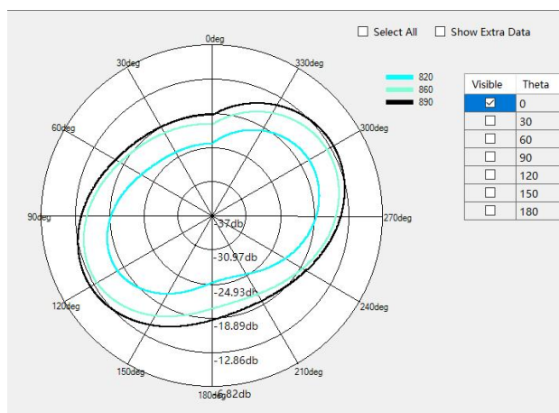
GSM 850/ WCDMA B5/ LTE B5/B26 Phi=0deg
