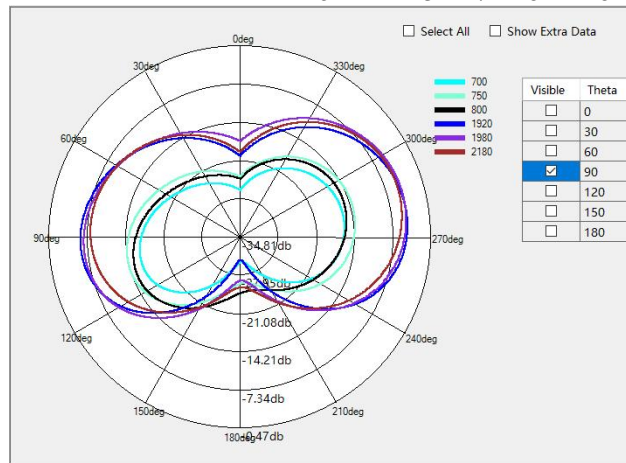
PCS/ WCDMA B1/B2/ LTE B1/B2/B25/B12/B13/B17/B28A/B28B Phi=0deg
