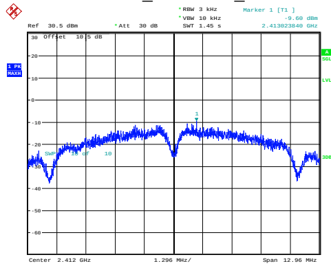
802.11b_2412MHz_Chain 0
