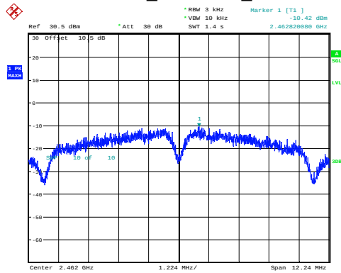
802.11b_2462MHz_Chain 0
