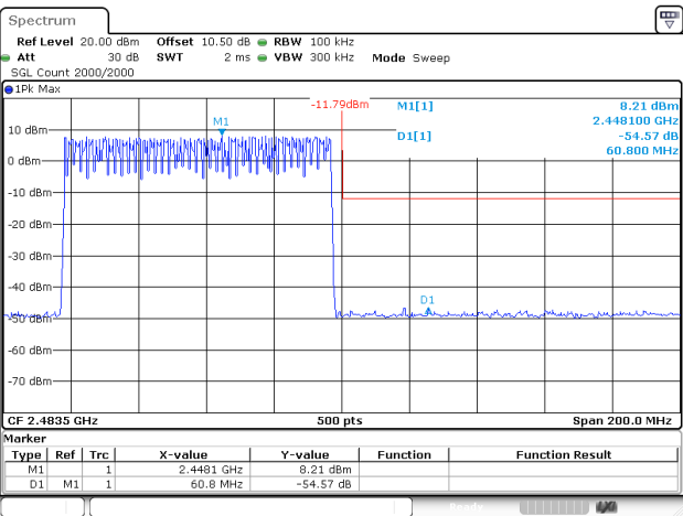
DH1_Hopping_Upper
