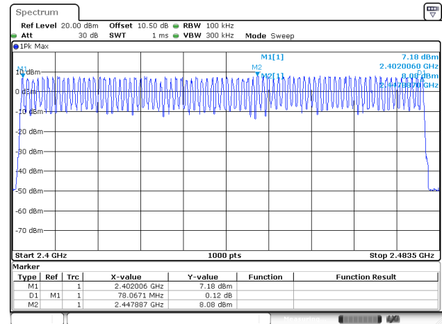
DH1_Hopping
