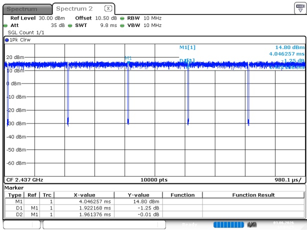
802.11n20_2437MHz
