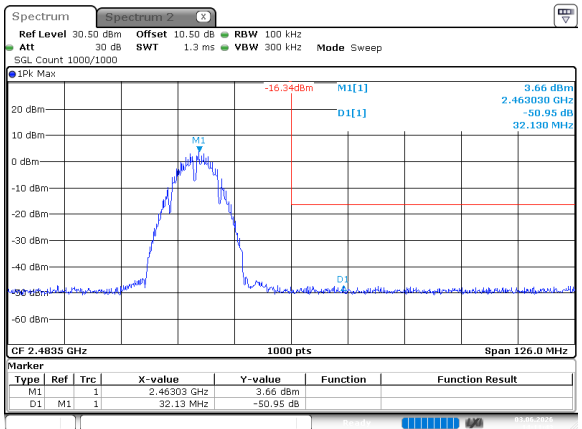
802.11b_2462MHz
