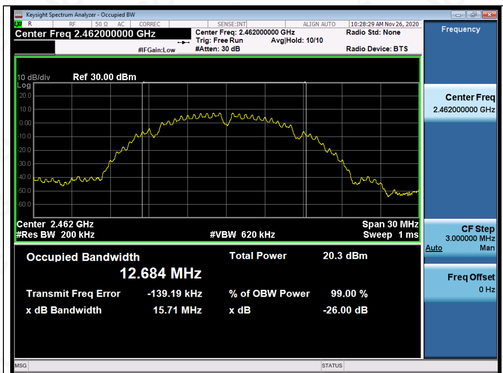
Test_Graph_802.11b_ANT1_2462_1Mbps_OBW
