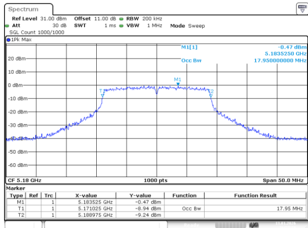
802.11ac20_5180MHz
