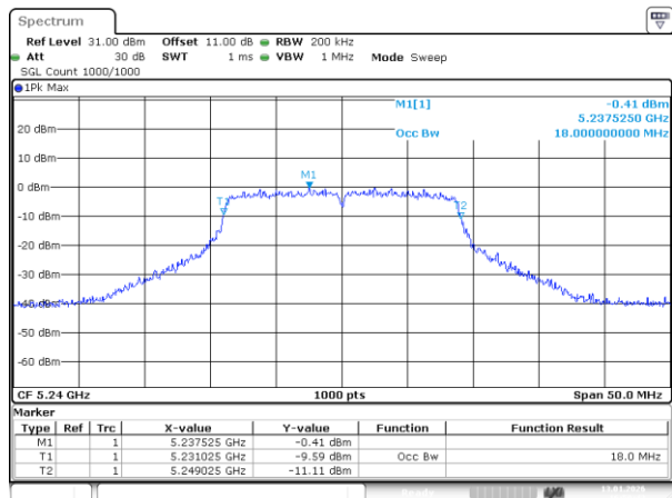
802.11ac20_5240MHz
