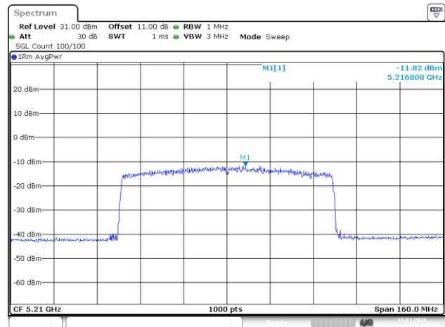
802.11ax80_5210MHz_RU_Full
