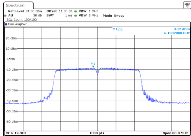
802.11ac40_5190MHz
