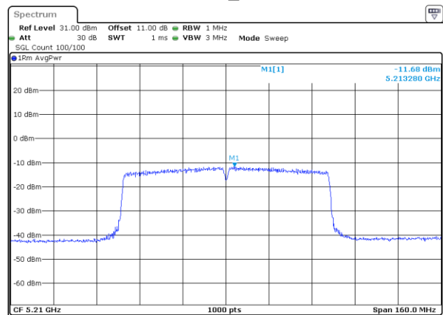
802.11ac80_5210MHz
