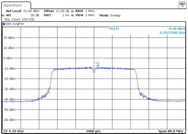
802.11ac40_5230MHz
