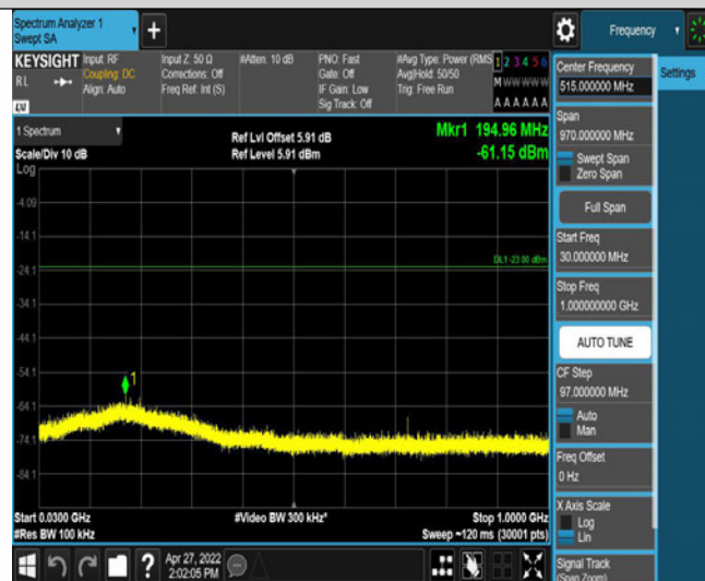
Band2-9538-1-30~1000MHz
