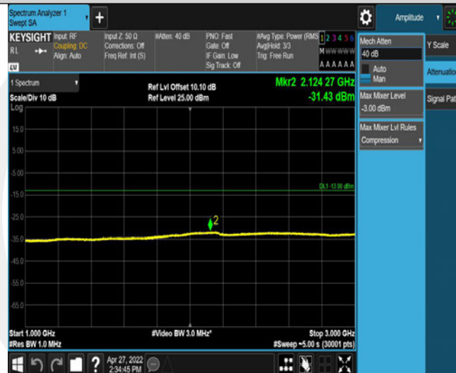
Band2-9538-5-1000~3000MHz
