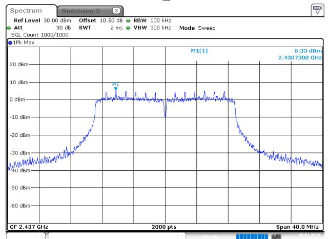
802.11n20_2437MHz
