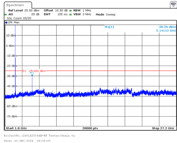
5MHz_Low_QPSK_25@0(1GHz~27.2GHz)
