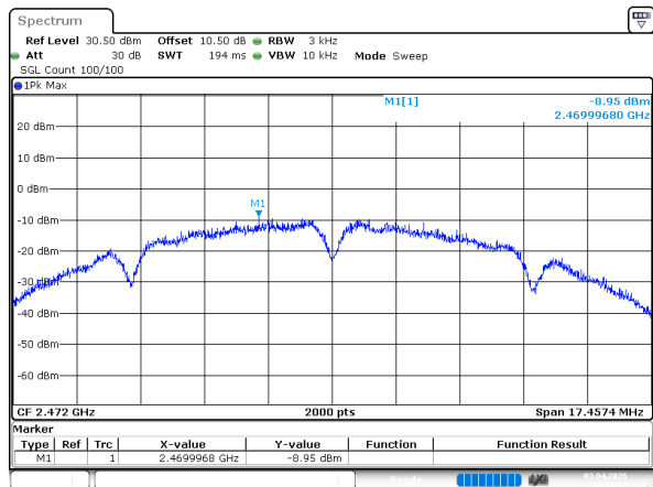
802.11b_2472MHz
