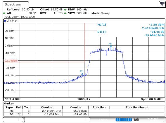
802.11n20_2412MHz
