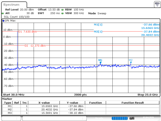
802.11b_2442MHz
