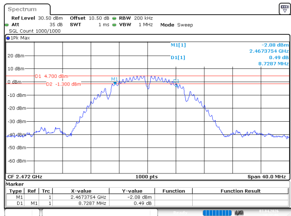
802.11b_2472MHz
