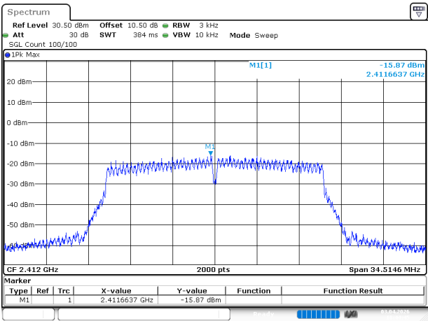
802.11n20_2412MHz
