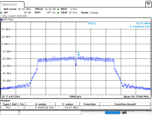
802.11n20_2442MHz
