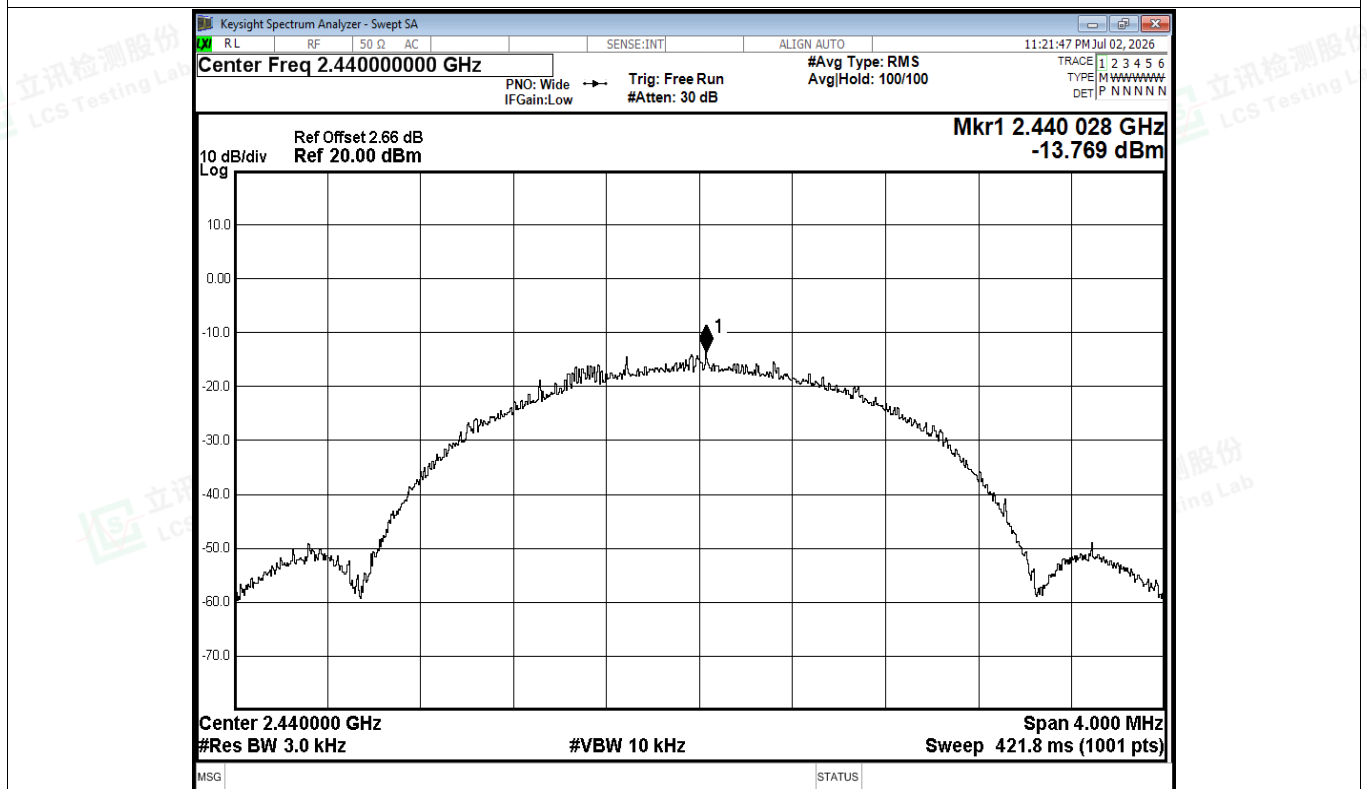
PSD NVNT BLE 2M 2440MHz Ant1
