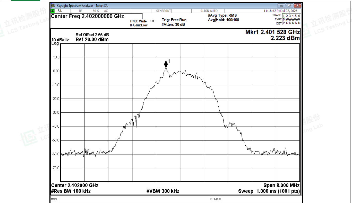
Band Edge NVNT BLE 2M 2402MHz Ant1 Ref
