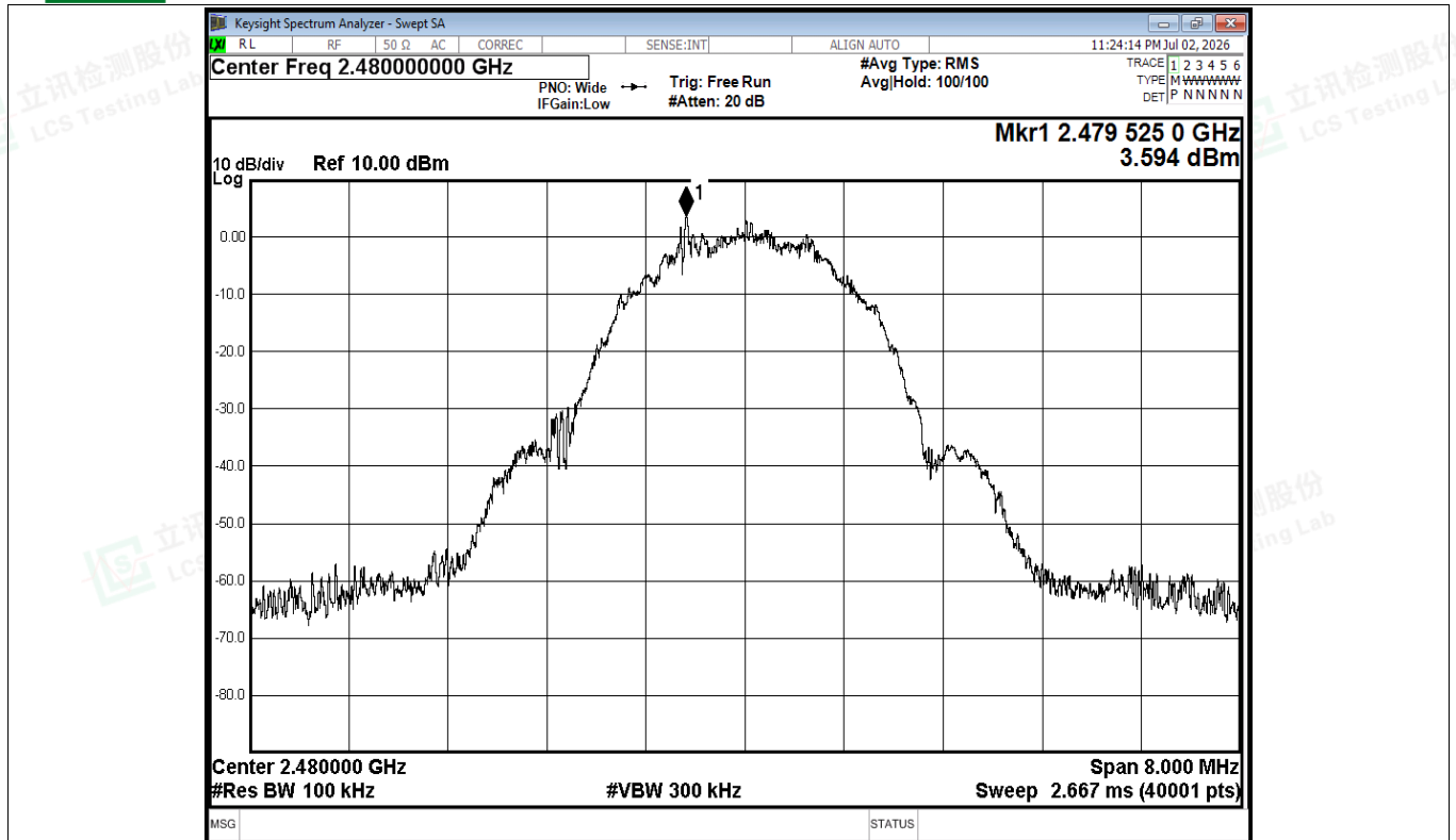
Tx. Spurious NVNT BLE 2M 2480MHz Ant1 Ref
