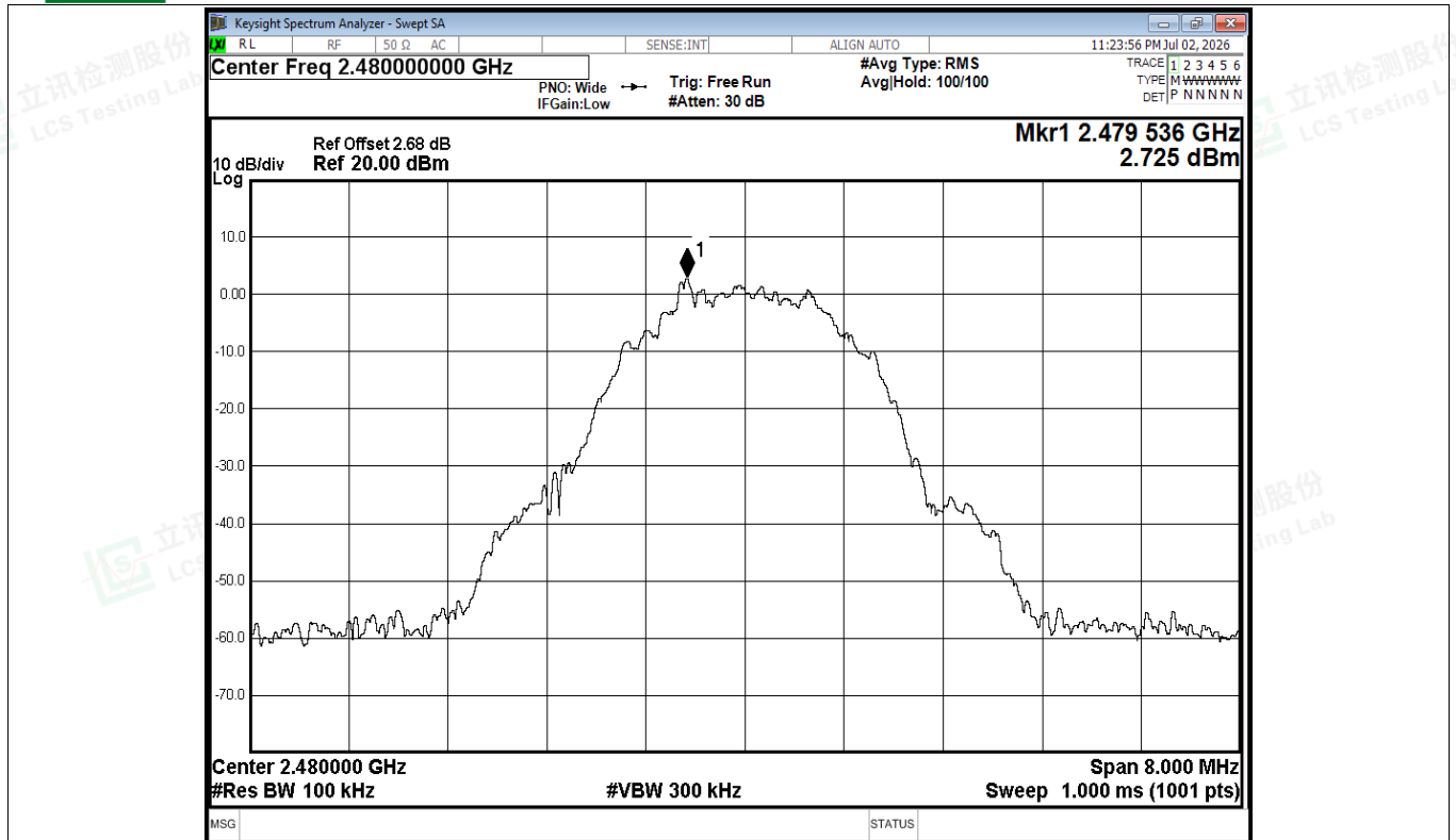
Band Edge NVNT BLE 2M 2480MHz Ant1 Ref
