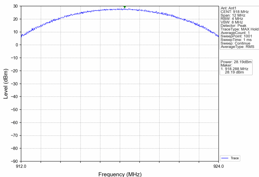
4M_MCH_918MHz_Ant1_NTNV
