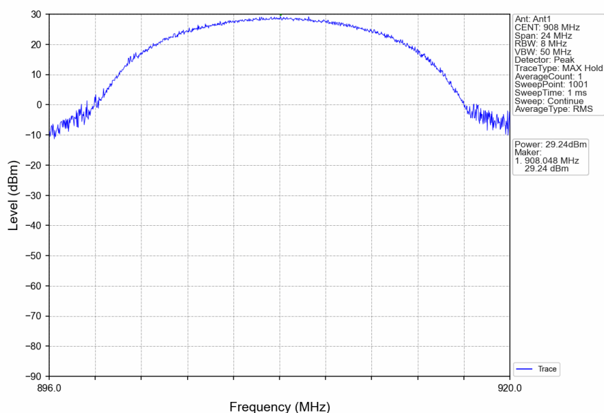
8M_LCH_908MHz_Ant1_NTNV
