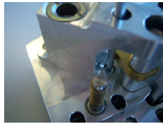
Schrauben mit W.6 lösen remove the screws with W.6
