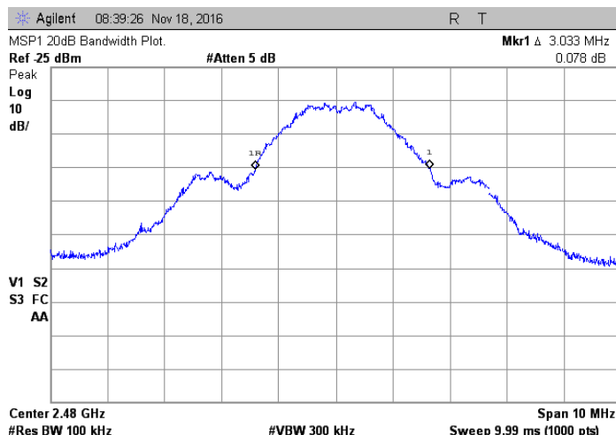
MSP1; 2480 MHz
