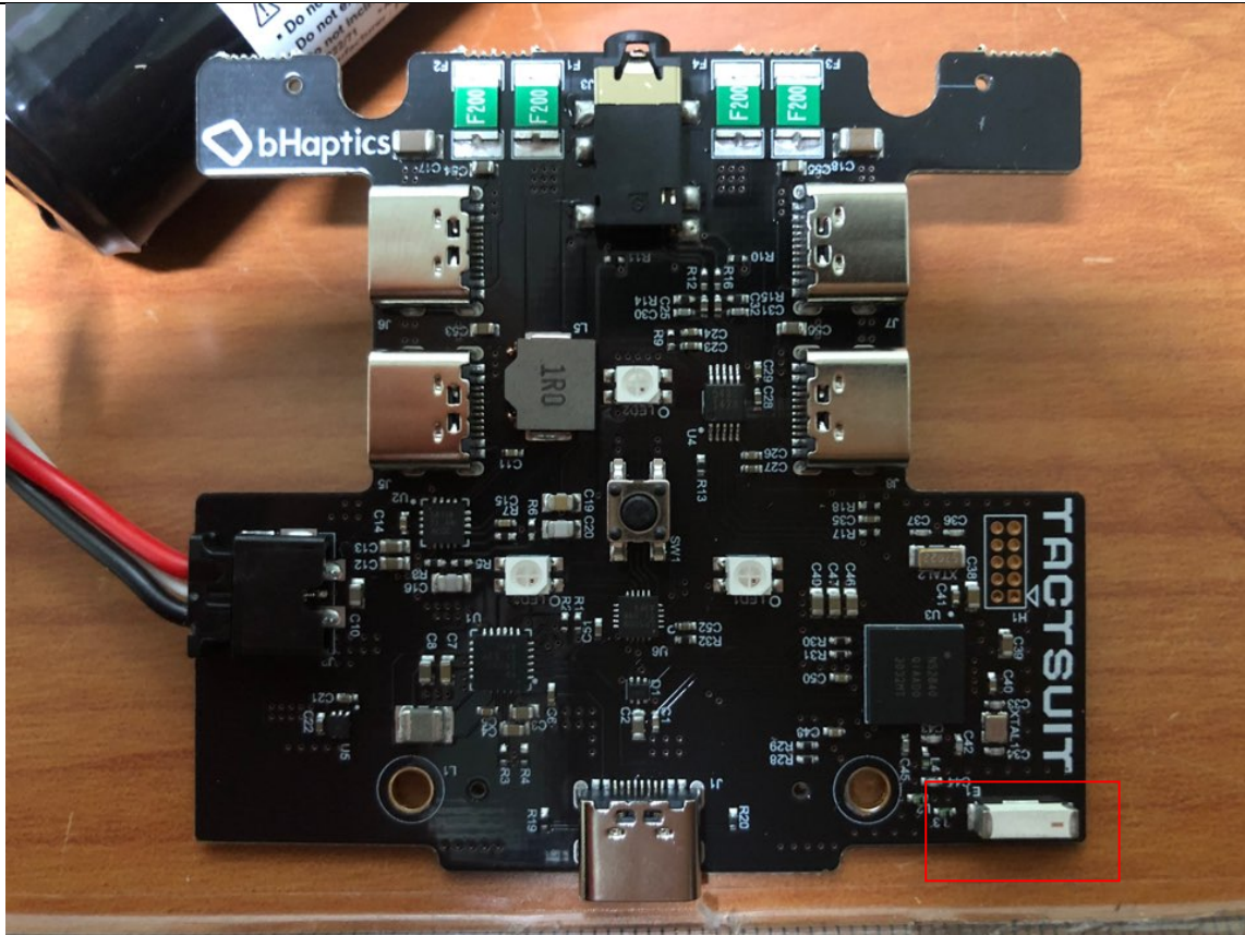
ANTENNA(2.4 GHz)
