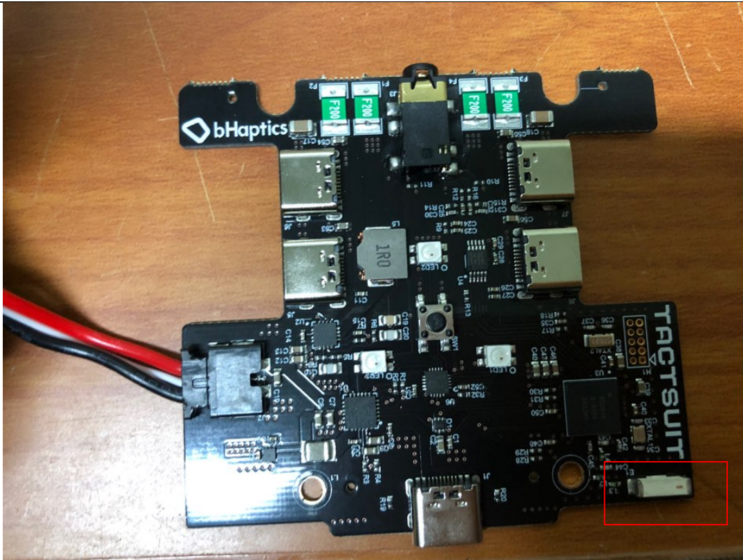
ANTENNA(2.4 GHz)
