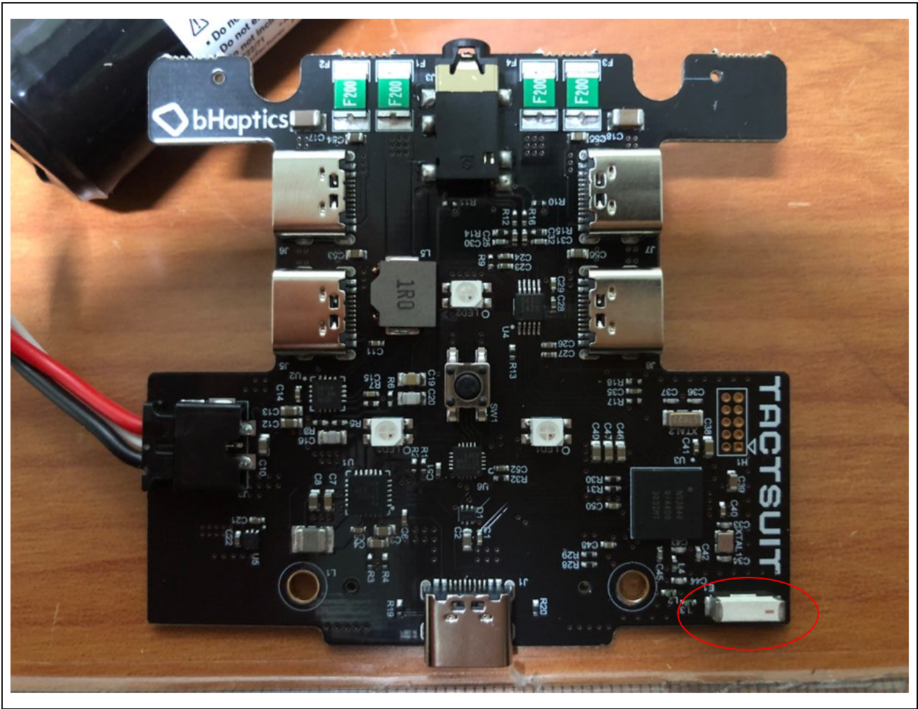
Antenna
