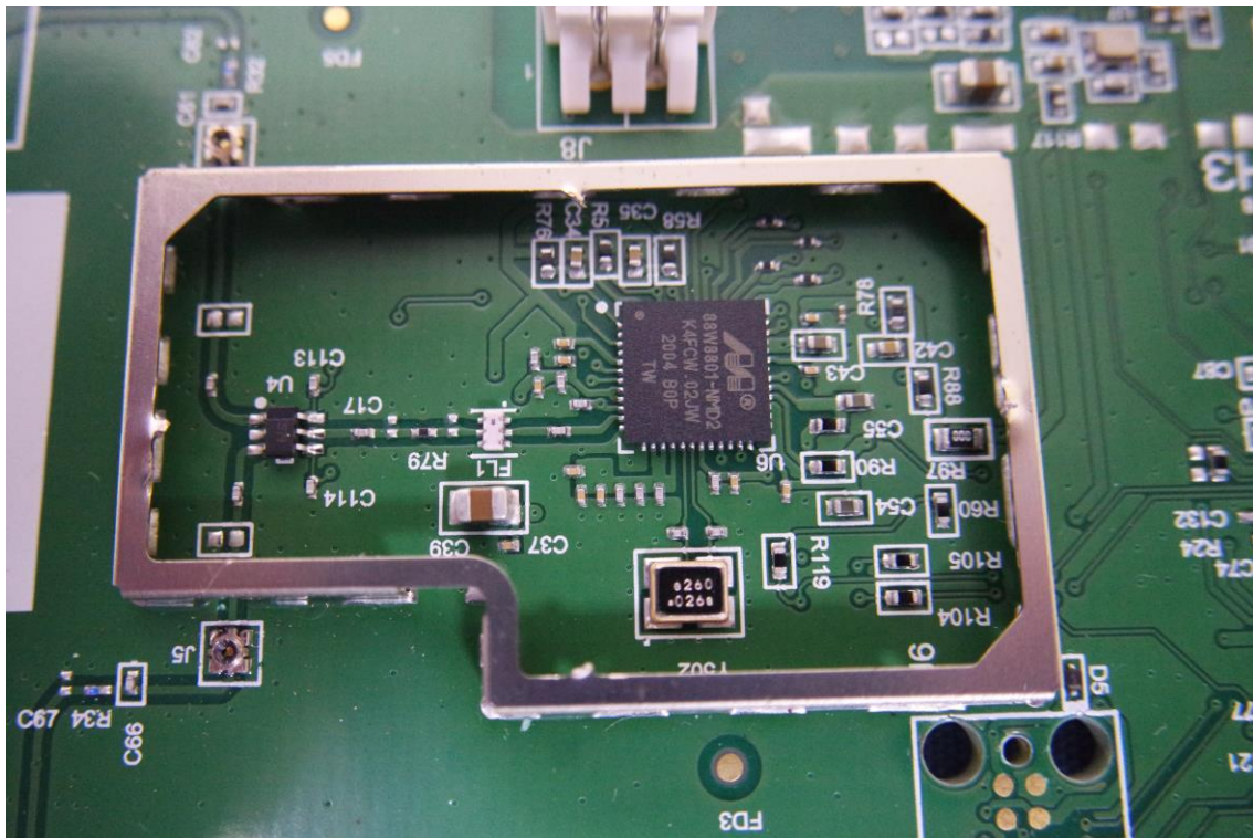
Wifi Module
